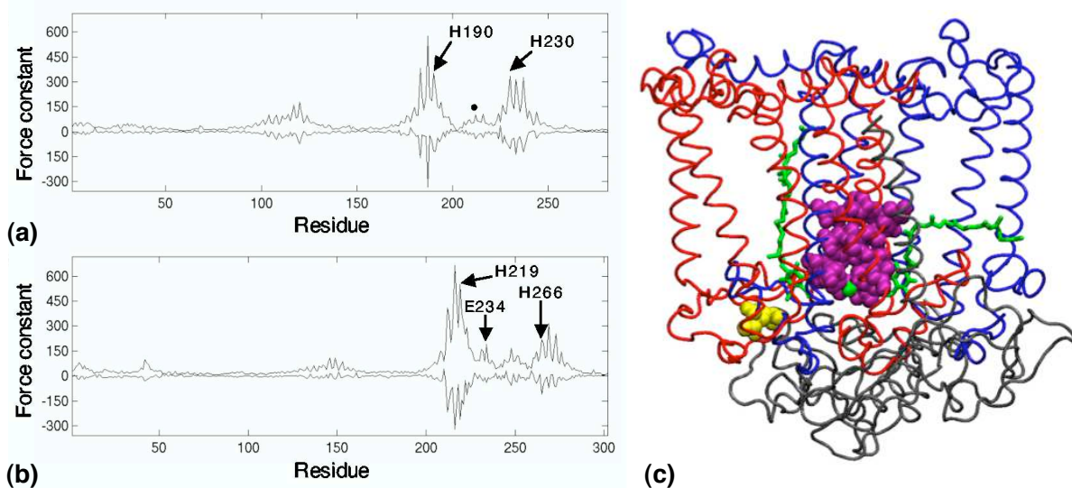
FIG. 2.6 – Profils de rigidité du CR de R. Sphaeroides , la ligne supérieure indique les constantes de forces des résidus dans la protéine native, tandis que la ligne inférieure indique les variations de flexibilité quand on passe au mutant AA, les résidus mutés sont signalés par un point noir, (a) chaîne L, (b) chaîne M. (c) Structure du mutant AA du CR de R. Sphaeroides avec les chaînes L (bleue), M (rouge) et H (noir). Les quinones Q_A et Q_B , ainsi que l'atome de fer hors-hème impliqué dans le transfert d'électron, sont indiqués en vert. Les résidus mutés L212 et L213 sont en jaune et les résidus dont les propriétés mécaniques sont les plus perturbées par la mutation sont en violet.
