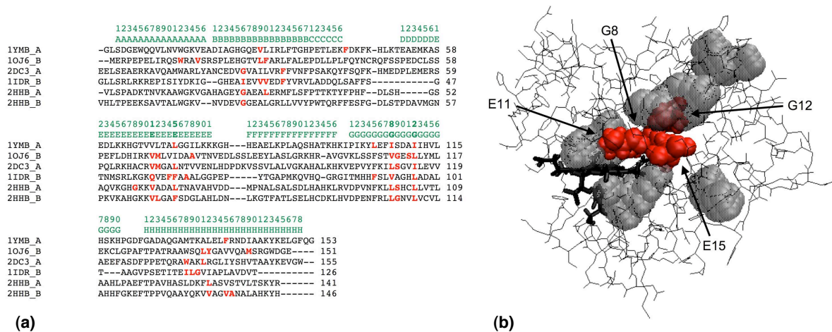
FIG. 2.8 – (a) Alignement des six séquences de globines, les résidus mécaniquement sensibles sont marqués en rouge (b) Noyau mécanique, en rouge, au cœur du réseau de cavités internes de la myoglobine.
