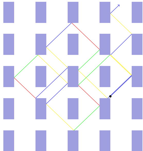
FIGURE 1.1 – Un morceau de trajectoire dans la table de billard V(a, b) avec a = 0.33 et b = 0.65 .
