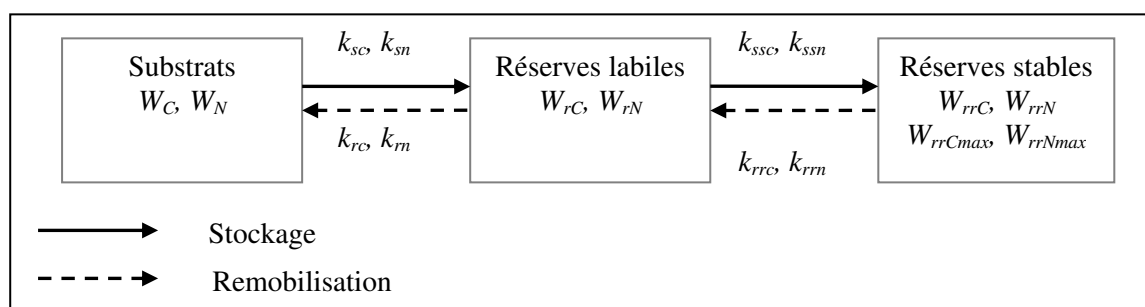
Fig. 6. Schéma en série du stockage et de la remobilisation des réserves dans PaSim.
