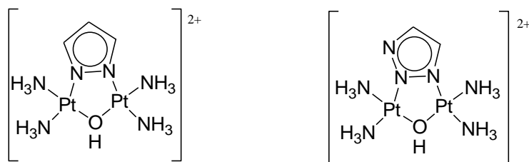
Figure 25. Complexes binucléaires de platine comportant des ligands pyrazolate et 1,2,3-triazolate.
