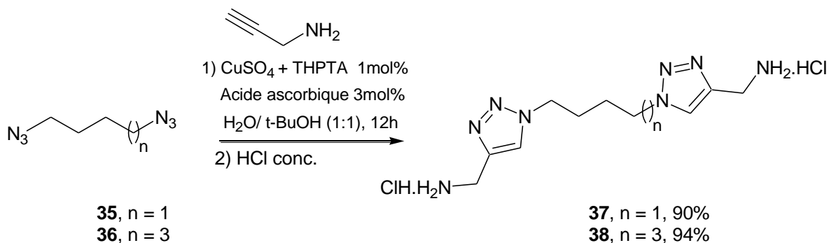
Schéma 11. Etape de cycloaddition entre composé diazotures et la propargylamine.
