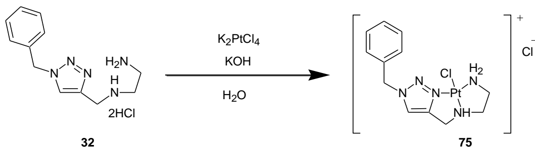
Figure 91. Complexation du platine par ligand triazole tridenté.
