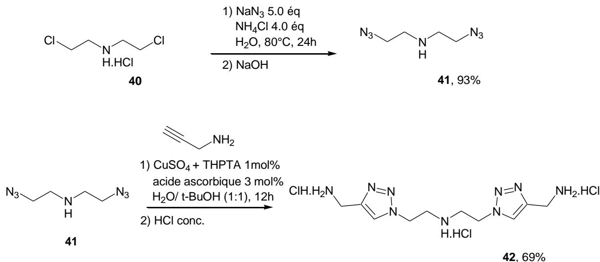
Schéma 13. Synthèse du ligand bis-triazole avec un pont aliphatique intégrant une amine.
