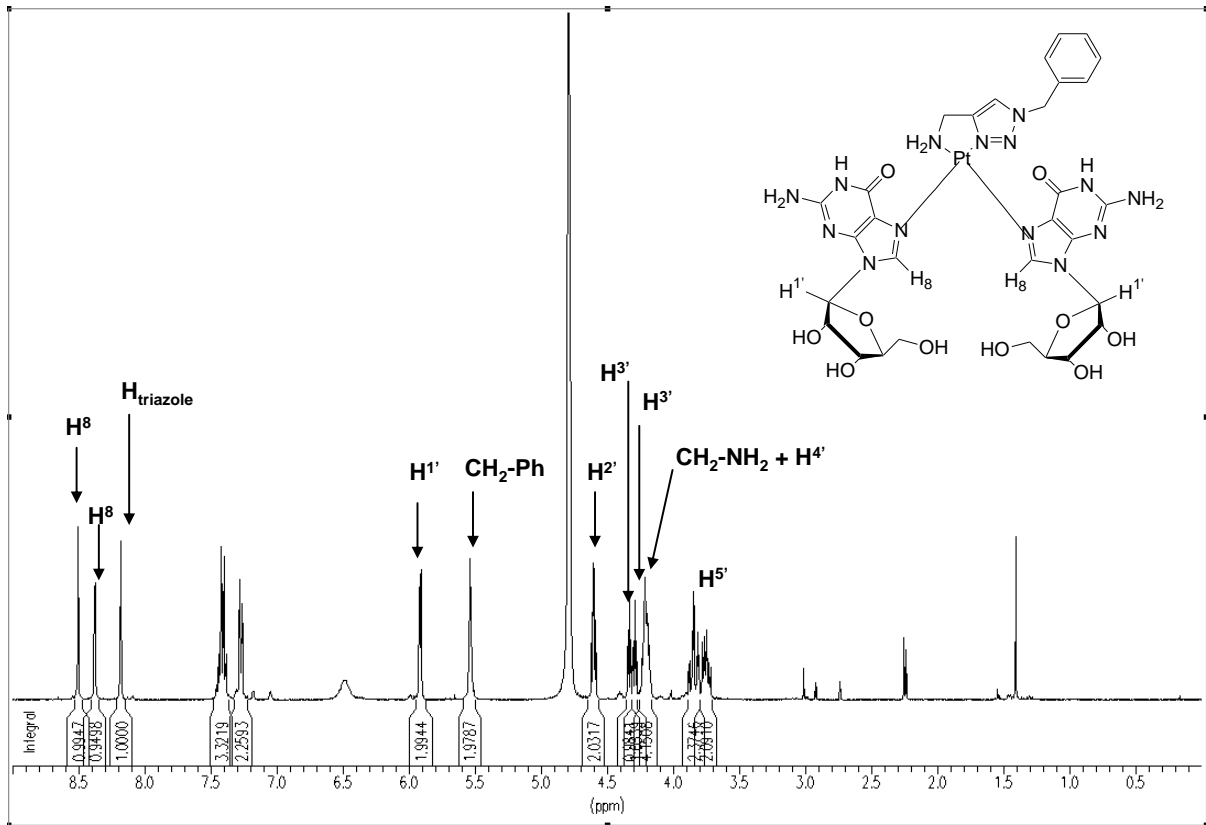
Figure 104. Spectre RMN 1 H du complexe platine guanosine 89 dans D 2 O (300 K).
