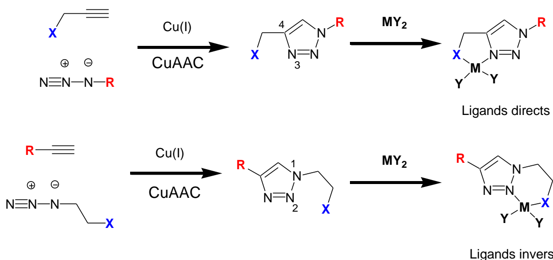
Figure 68. Stratégies de synthèse de complexes de platine comportant des ligands 1,2,3-triazoles bidentes.
