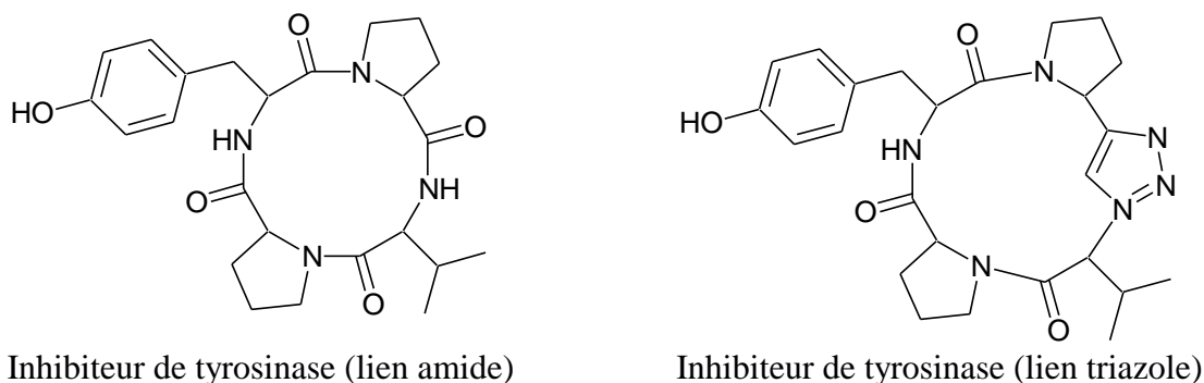
Figure 56. Peptide cyclique Tyr-Pro-Val-Pro inhibiteur de la tyrosinase.
