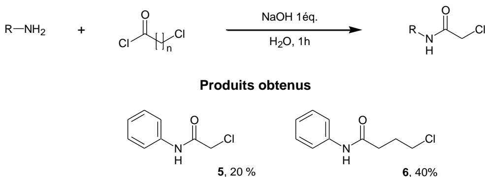
Figure 72. Essais d'acylation d'amine par méthode de Schotten-Baumann dans l'eau.
