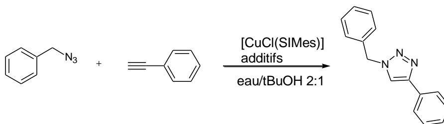
Figure 127. Criblage d'additifs pour la réaction de CuAAC entre l'azoture de benzyle et le phénylacétylène catalysée par le complexe [CuCl(SIMes)].
