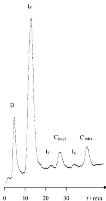
Figure 112. Chromatogramme HPLC du mélange réactionnel issu de l'action du dérivé diaqua du cisplatine avec l'hairpin. D : hairpin libre, I 5' , I 3' , I G : monoadduit respectivement sur G 1 , G 2 et G 3 , C intra : chelation intrabrin, C inter : pontage interbrins. 185
