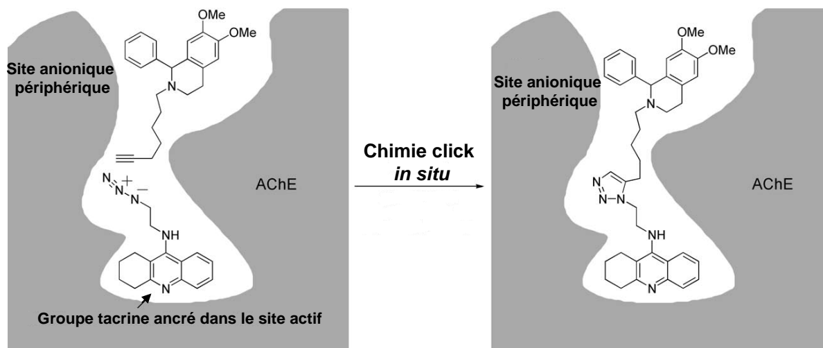
Figure 61. Représentation schématique de la réaction de cycloaddition alcyne-azote à l'intérieur du site actif de l'acétylcholinestérase (AChE).
