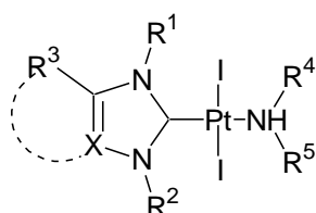
Figure 17. Structure générale des complexes (NHC)PtI 2 (amine).
