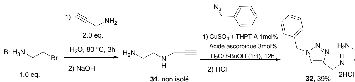
Schéma 8. Les étapes successives pour la synthèse du ligand 1,2,3-triazole tridenté.
