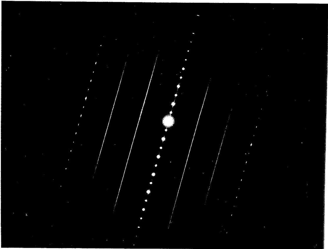
Fig. 30 Diagramme de microdiffraction électronique de clinochlore totalement désordonné Dora Maira-Italie
