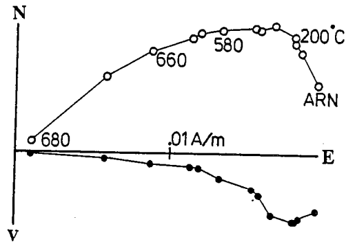
Fig.II.15 - Courbe de désaimantation (projection orthogonale) site TM.
