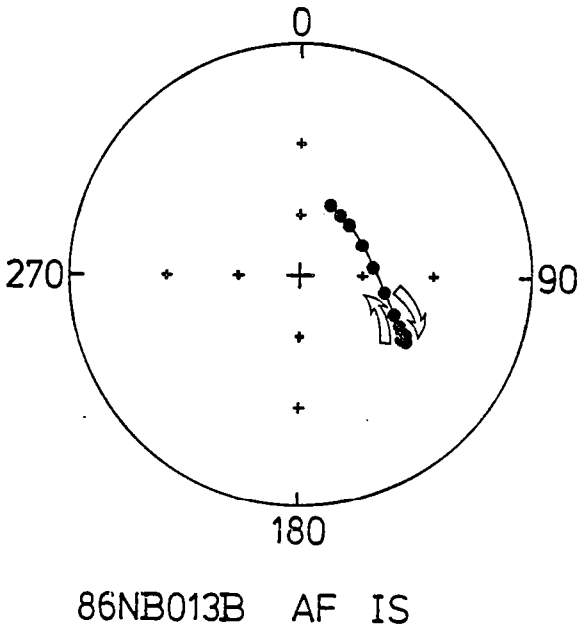
Fig.I.40 - Courbes de désaimantations (diagrammes orthogonaux) et projections stéréographiques de l'échantillon 86NB013 a : désaimantation thermique ; b : par champs alternatifs
