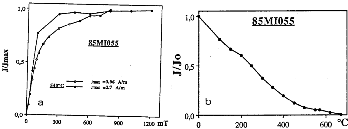
Fig.I.43 - ARI : (a) ARI avant et après chauffe de l'échantillon 85MI055. (b) : désaimantation thermique de l'ARI.
