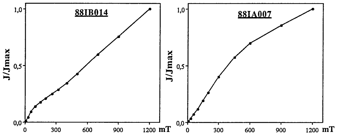
Fig.II.37 - Courbes d'ARI indiquant la présence de champs coercitifs élevés.
