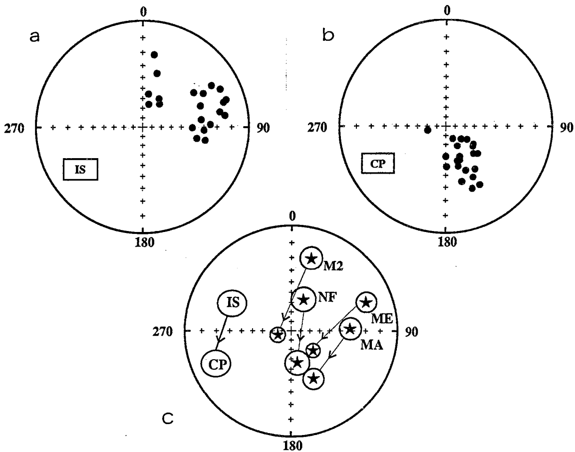
Fig.I.36 - Aimantations HT (hautes températures).
