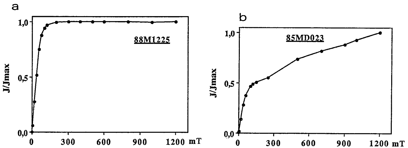
Fig.I.34 - ARI : courbes d'acquisitions d'aimantations isothermes. a : minéral à coercivité faible ; b : présence simultanée de deux coercivités (faible et forte)
