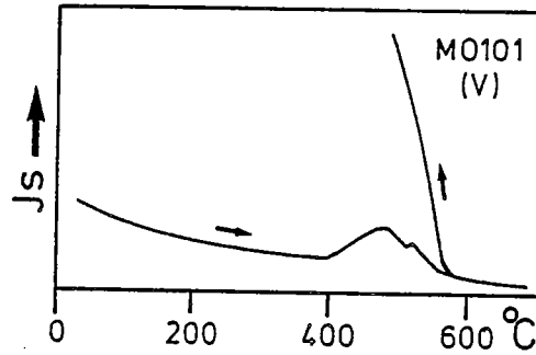
Fig.I.25 - Courbe thermomagnétique montrant des transformations minéralogiques.
