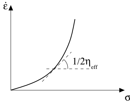
FIG. A.5: Réponse rhéologique d'un corps visqueux non linéaire selon une loi puissance de fluage. La viscosité varie avec la contrainte (ou avec le taux de déformation).
