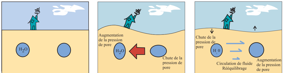
FIG. 3.1: Schéma simplifié du rééquilibrage de la pression de pore à la suite d'un séisme sur une faille décrochante (Jónsson et al., 2002).
