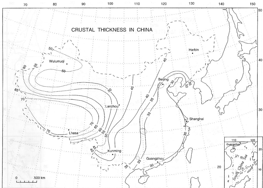
FIG. 1.11: Epaisseur crustale sous la Chine obtenue principalement à partir de données de sismique-réfraction (Li et Mooney, 1998). Les contours représentés par des lignes sont plus fiables que ceux représentés par des pointillés.
