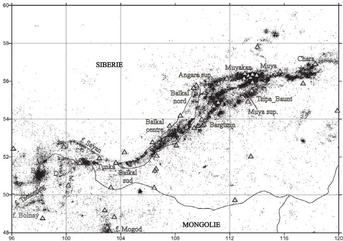
FIG. 1.29: Carte de la sismicité dans la région du rift Baïkal entre 1960 et 2000 (Déverchère et al., 2001). Catalogue de l'Institut de la Croûte Terrestre, Irkoutsk, établi sur la base du réseau régional (triangles). B : Busingol, D : Darkhat, K : Khubsugul, f. pour faille.
