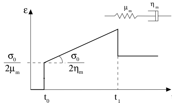
FIG. A.7: Modèle rhéologique de Maxwell.
