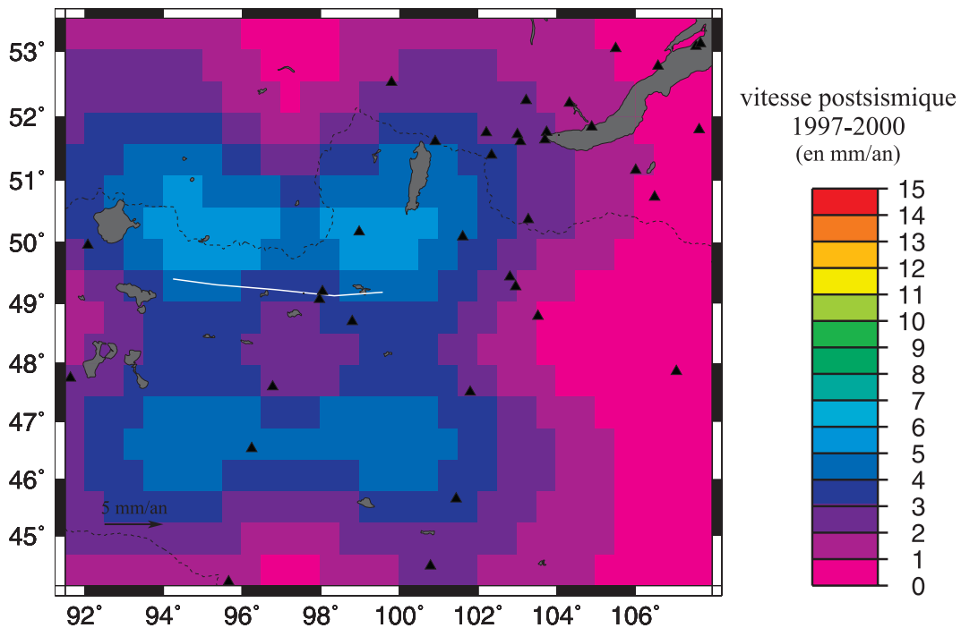
FIG. 3.5: Vitesses postsismiques 1997-2000 pour un modèle de Terre composé d'une croûte supérieure élastique de 30 km d'épaisseur, d'une croûte inférieure viscoélastique de 15 km d'épaisseur avec \eta_c = 3 \times 10^{18} Pa.s et d'un manteau supérieur élastique. Le trait blanc correspond à la rupture simplifiée de Bolnai (Vergnolle, 2000).
