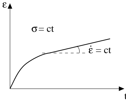
FIG. A.4: Réponse rhéologique d'un corps visqueux linéaire. \varepsilon = f(t) est la courbe de fluage à \sigma constant.
