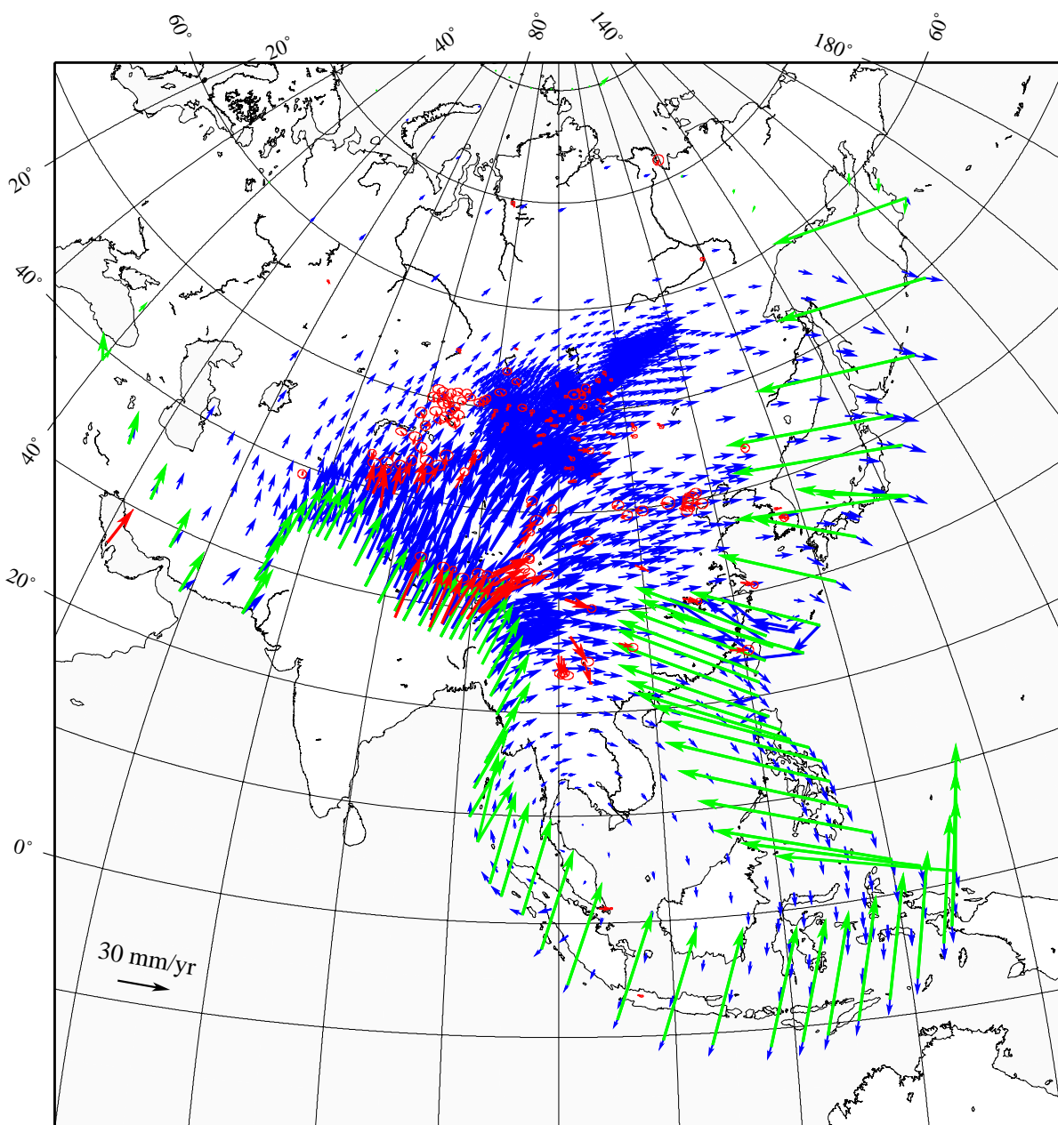
FIG. 6.7: Vitesses horizontales prédites par un modèle utilisant les paramètres suivants : rhéologie 2 , T_c = 25 MPa, T_o = 2 MPa, f_i = 0,9 et f_f = 0,08 . Flèches vertes : vitesses aux limites, flèches bleues : vitesses modélisées, flèches rouges : vitesses GPS.
