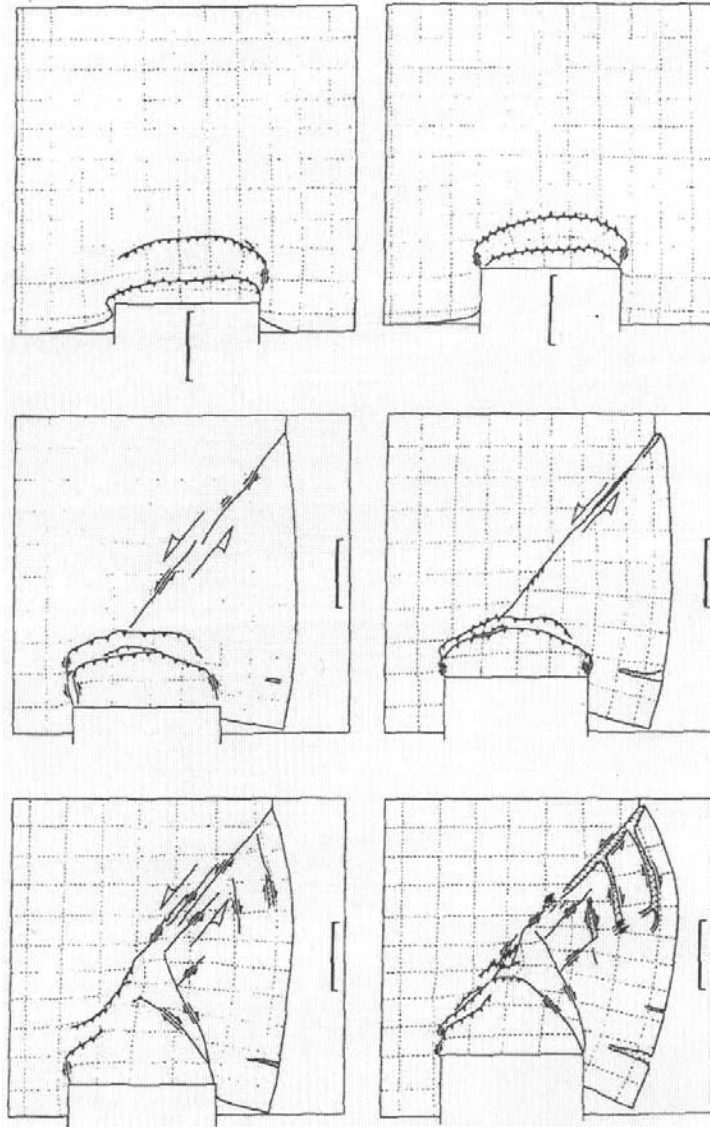
FIG. 1.34: Schémas de poinçonnement d'une lithosphère à trois couches (sable-silicone-miel) par un piston rigide en fonction du degré de confinement latéral sur le bord est : confinement rigide (en haut), modéré (au milieu) et faible (en bas) (Davy et Cobbold, 1988). Dans l'expérience modérément confinée et faiblement confinée sur le bord est, il y a développement de failles inverses au nord du front de collision, d'une seule grande faille sénestre, équivalent de la zone sismogène Tien Shan-Baïkal-Sakhaline, et apparition tardive de petits décrochements dextres transtensionnels parallèles à la marge orientale dans l'expérience faiblement confinée.
