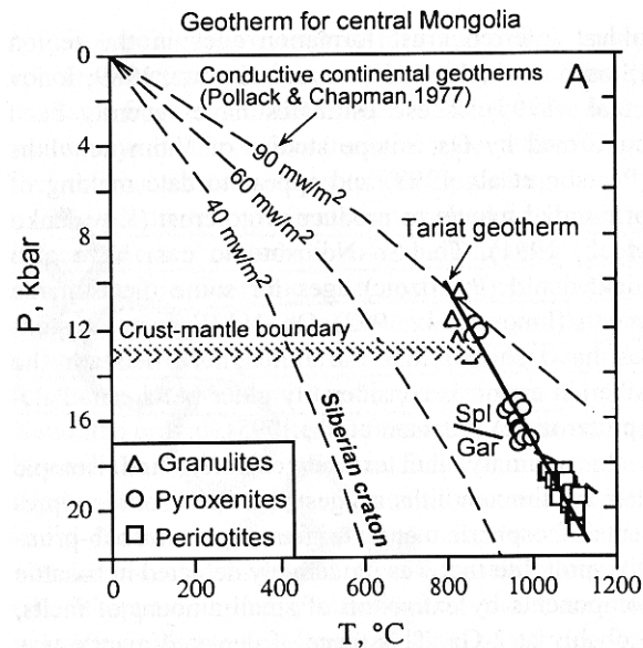
FIG. 1.18: Géotherme calculé à partir de l'analyse pétrologique et thermobarométrique de xénolithes crustales et mantelliques échantillonnés dans le champ volcanique du Tariat (NE du dôme de Hangai) (Ionov et al., 1998).
