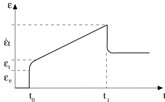
FIG. A.6: Déformation théorique d'un corps viscoélastique en fonction du temps sous une contrainte constante appliquée entre t_0 et t_1 .
