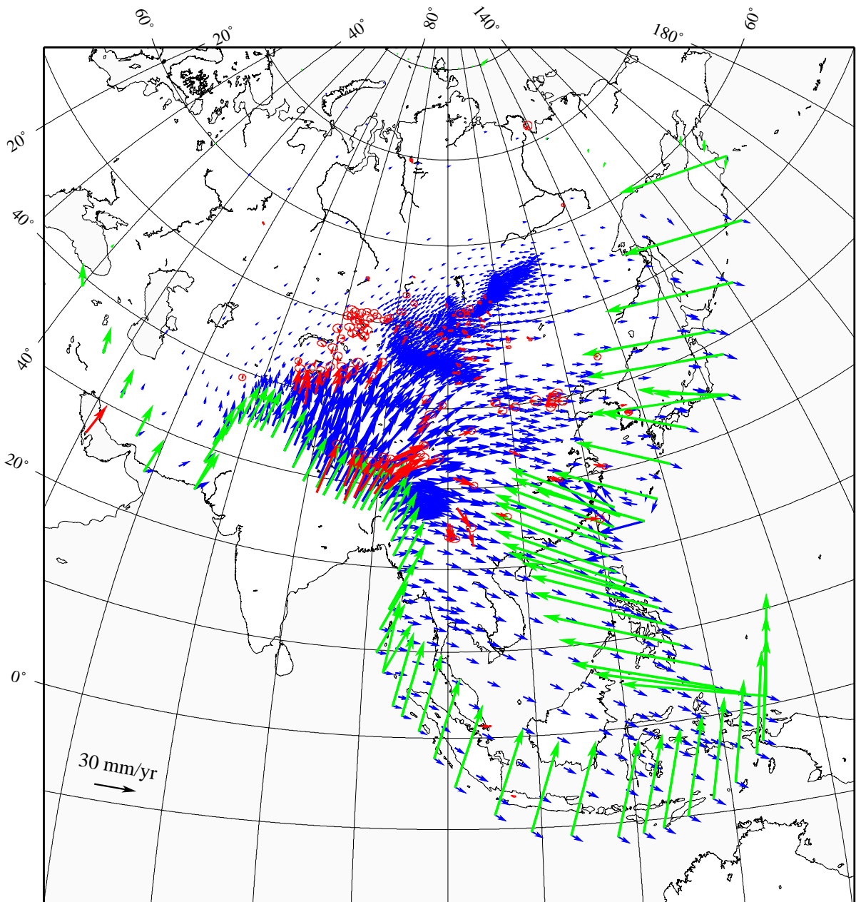
FIG. 6.4: Modèle de référence. Vitesses horizontales prédites par un modèle utilisant les paramètres suivants : rhéologie 1, T_c = 25 MPa, T_o = 1 MPa, f_i = 0,9 et f_f = 0,08 . Flèches vertes : vitesses aux limites, flèches bleues : vitesses modélisées, flèches rouges : vitesses GPS.
