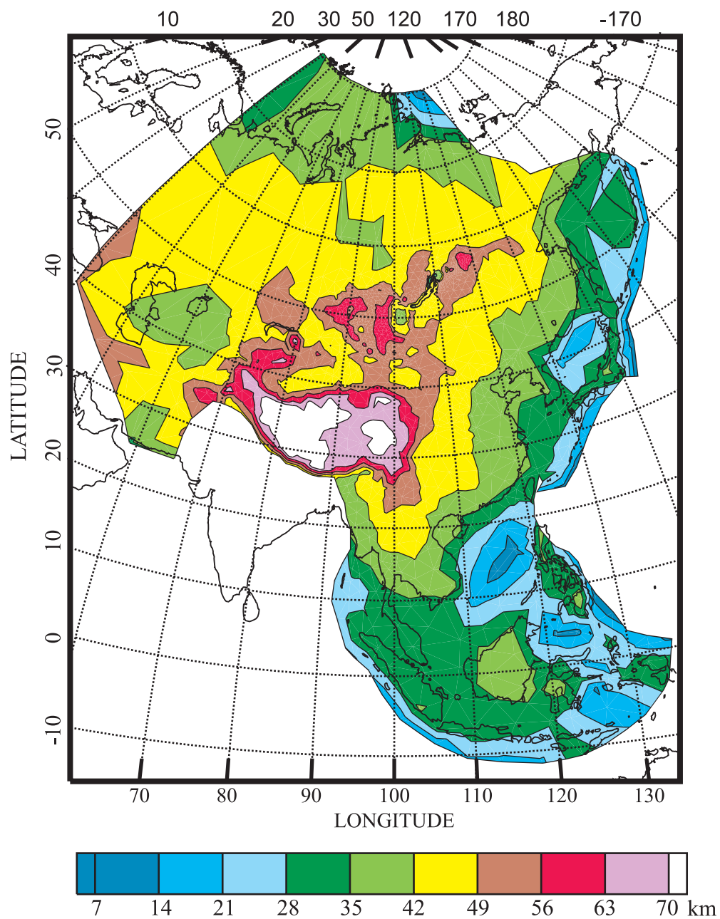
FIG. 5.9: Epaisseur crustale calculée à partir des paramètres de la rhéologie 2.
