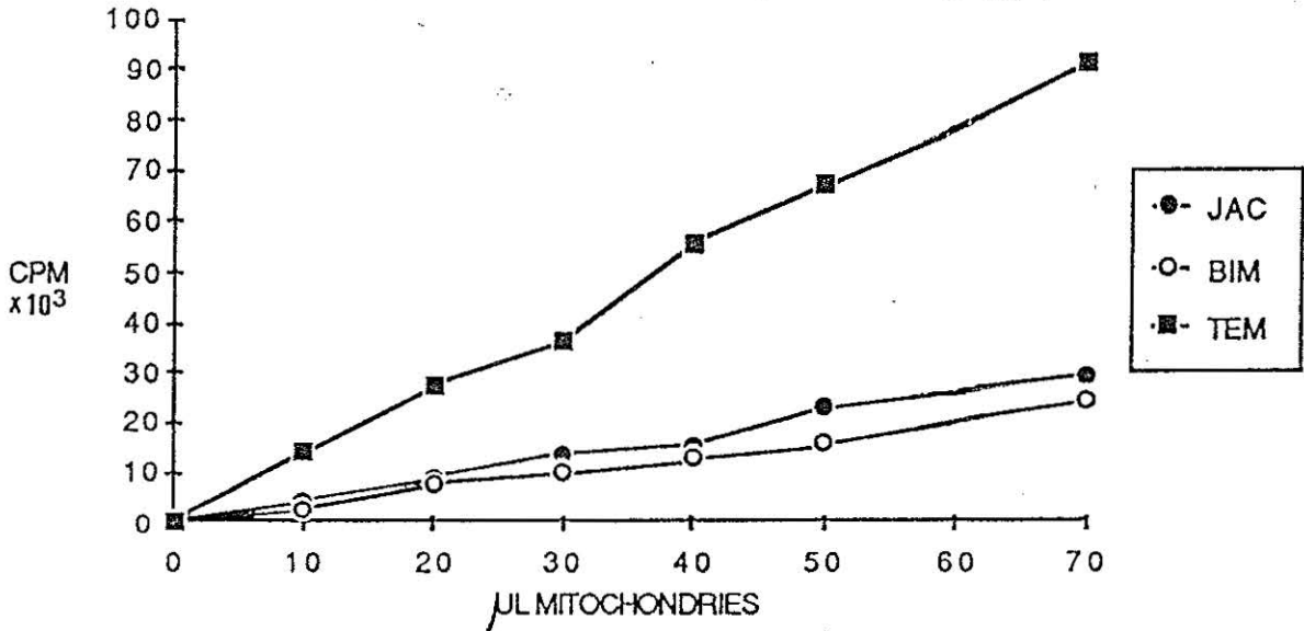
Fig. 55 : Immunoprécipitation des monoamine oxydases de foie humain par les anticorps anti-M6 : effet de la quantité de protéines mitochondriales.
