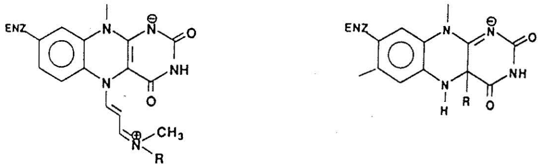
Fig. 50 : Structure de certains inhibiteurs irréversibles des monoamine oxydases.
