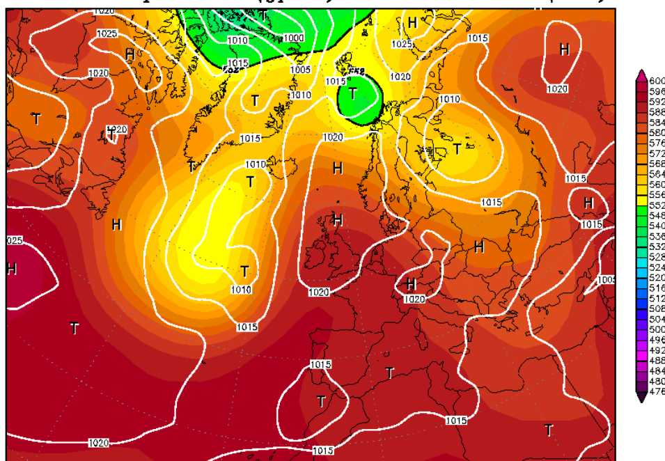
Figure 11.2 : Géopotentiels à 500hPa issues des réanalyses NCEP du 8 août 2003 (Source : www.wetterzentrale.de )
