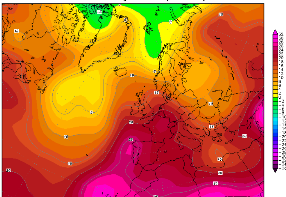
Figure 11.3 : Températures en °C sur l'Europe Occidentale à 850 hPa le 8 août 2003 issues des réanalyses NCEP (Source : www.wetterzentrale.de )
