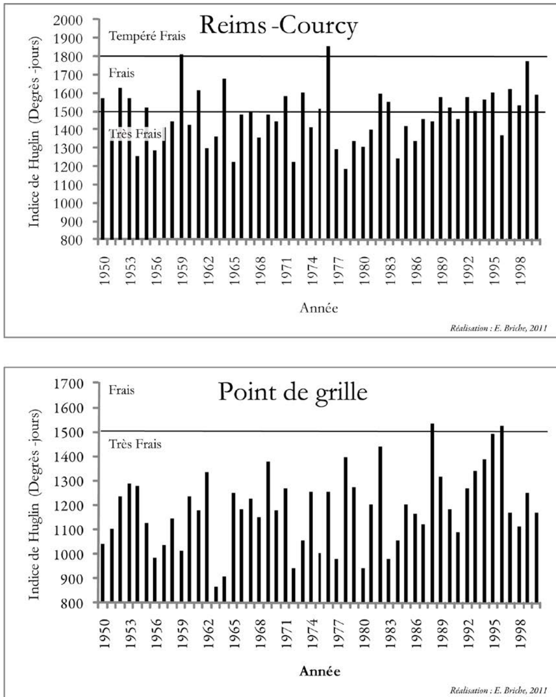
Figure 8.12 : Évolution de l'indice de Hugin de 1950 à 2000 pour le point de grille et la station Reims-Courcy (Données : Météo-France – CNRM).
