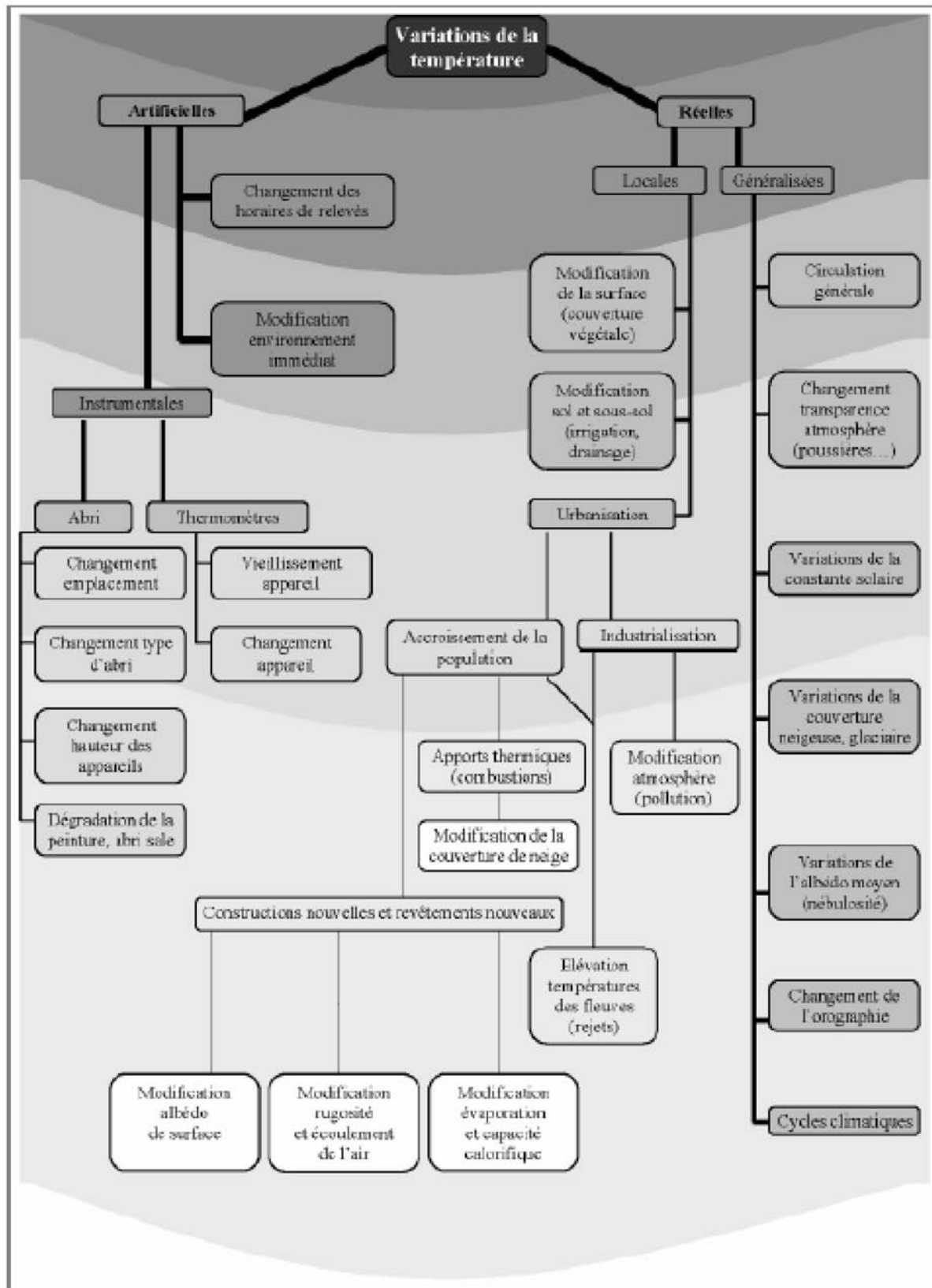
Figure 4.4 : Liste des facteurs de toutes origines pouvant entraîner une modification de la température mesurée. L'intensité de gris et les cercles concentriques soulignent le caractère additif des différentes causes de variation des températures. (Source : Mitchell et Dettwiler in Choissnel, 2002).
