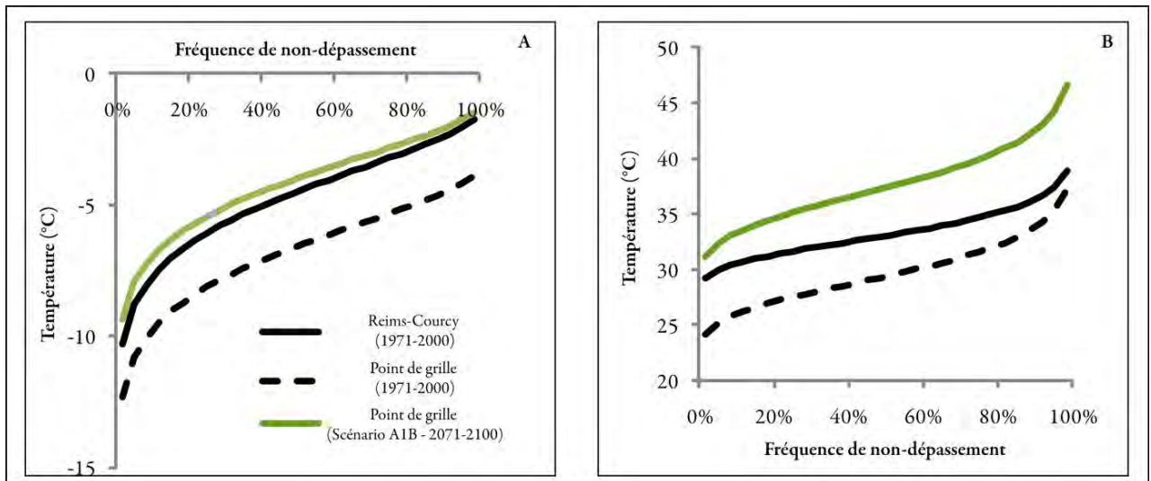
Figure 9.5 : Comparaison entre la station Reims-Courcy et le point de grille du modèle ARPEGE-Climat (RETIC) pour les températures minimales journalières (A) au printemps (mars-avril) et maximales journalières (B) estivales (juin, juillet et août) pour des périodes de retour d'un jour (Données : Météo-France – CNRM, CIVC).
