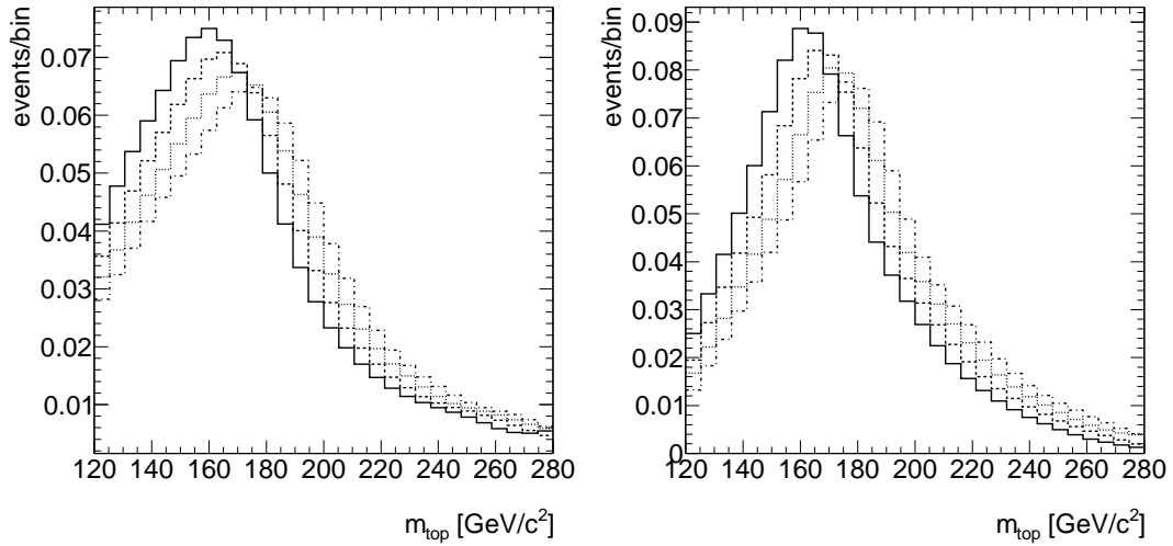
FIG. 10.3 – Distributions de m_{top} pour différentes hypothèses de masse du quark top, à gauche pour le top leptonique entre 145 \text{GeV}/c^2 et 200 \text{GeV}/c^2 et à droite pour le top hadronique entre 160 \text{GeV}/c^2 et 190 \text{GeV}/c^2 , après stabilisation.
