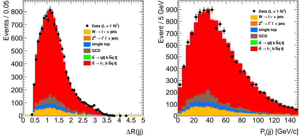
FIG. 6.8 – A gauche : Distance angulaire entre les deux jets reconstruisant le boson W après sélection de la meilleure combinaison par la fonction de séparation. A droite : Impulsion transverse du boson W hadronique reconstruit après sélection de la meilleure combinaison par la fonction de séparation.
