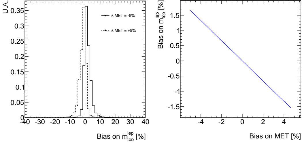
FIG. 5.6 – Biais sur la masse du top induit par une variation de E_{\text{T}}^{\text{miss}} de -5\% et +5\% (gauche). Propagation de la décalibration de E_{\text{T}}^{\text{miss}} à la masse du top leptonique pour des événements t\bar{t} semileptoniques (droite).
