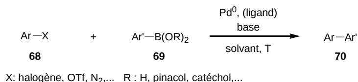
Schéma 13 : couplage de Suzuki-Miyaura
