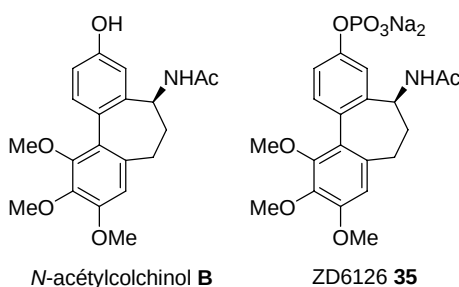
Figure 23 : les dérivés du N-acétylcolchinol B
