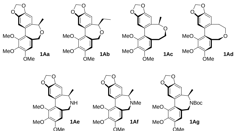
Figure 32 : analogues hydribes stéganes/allocolchicinoïdes
