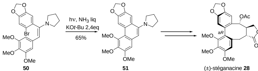
Schéma 4 : synthèse de la (±)- stéganacine 28 par Raphael et coll.
