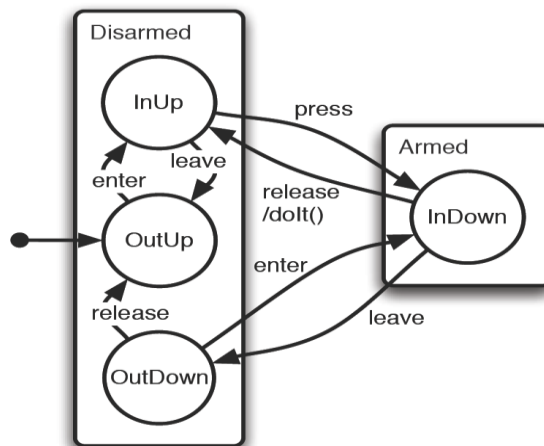
Figure II.7 modélisation du comportement d'un bouton en Hierarchical state machine
