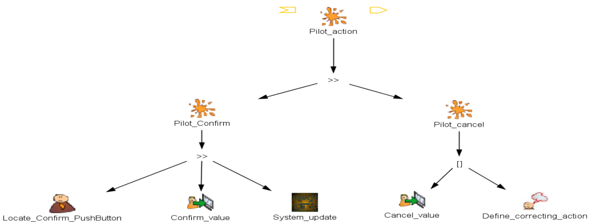
Figure V.21 Modèle de tâche de l'interaction en entrée de l'approche mixte (2)
