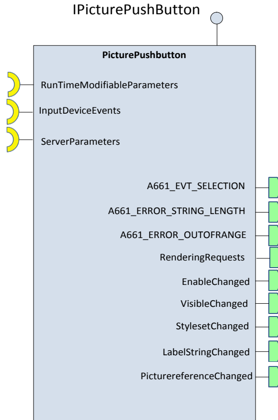
Figure IV.9 Modèle ICompoNet du PicturePushButton
