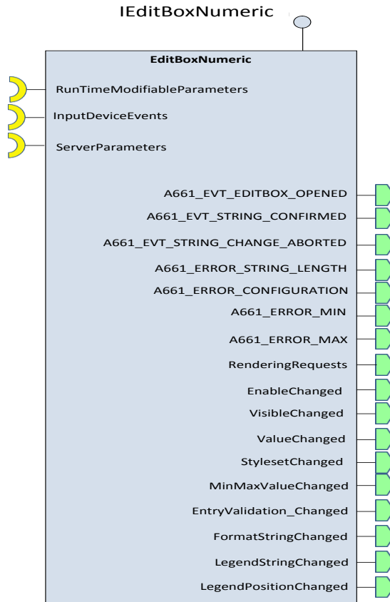
Figure IV.21 Modèle ICompoNet de l'EditBoxNumeric
