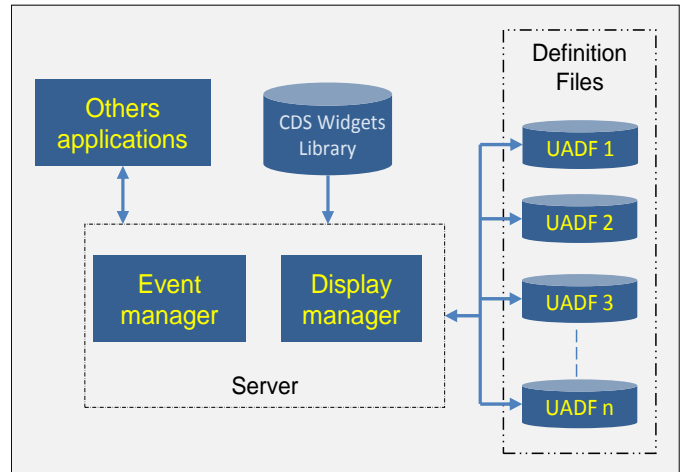
b) Architecture logicielle DU
