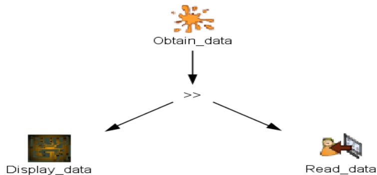
Figure IV.35 Modèle de tâche de l'interaction en sortie cas zéro défaut
