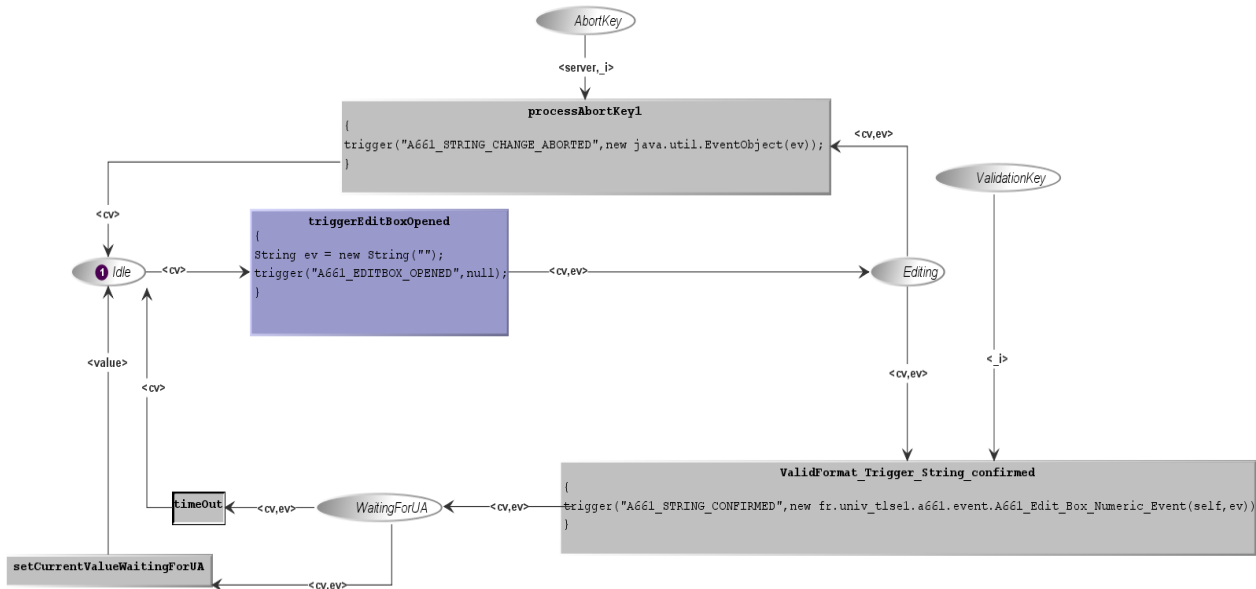
Figure IV.23 Etat editing de l'EditBoxNumeric
