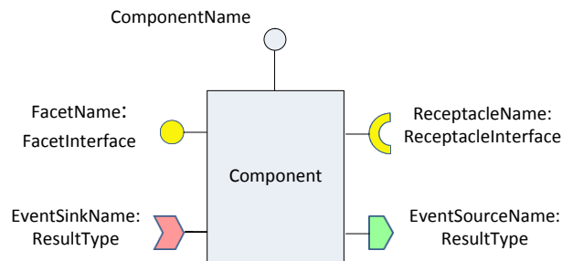
Figure II.24 Syntaxe graphique des CompoNets
