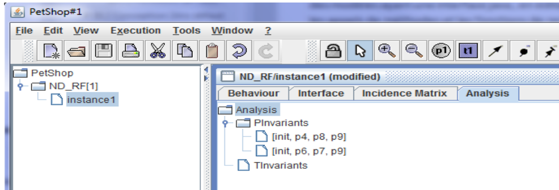
Figure II.30 Analyse d'invariants dans PetShop
