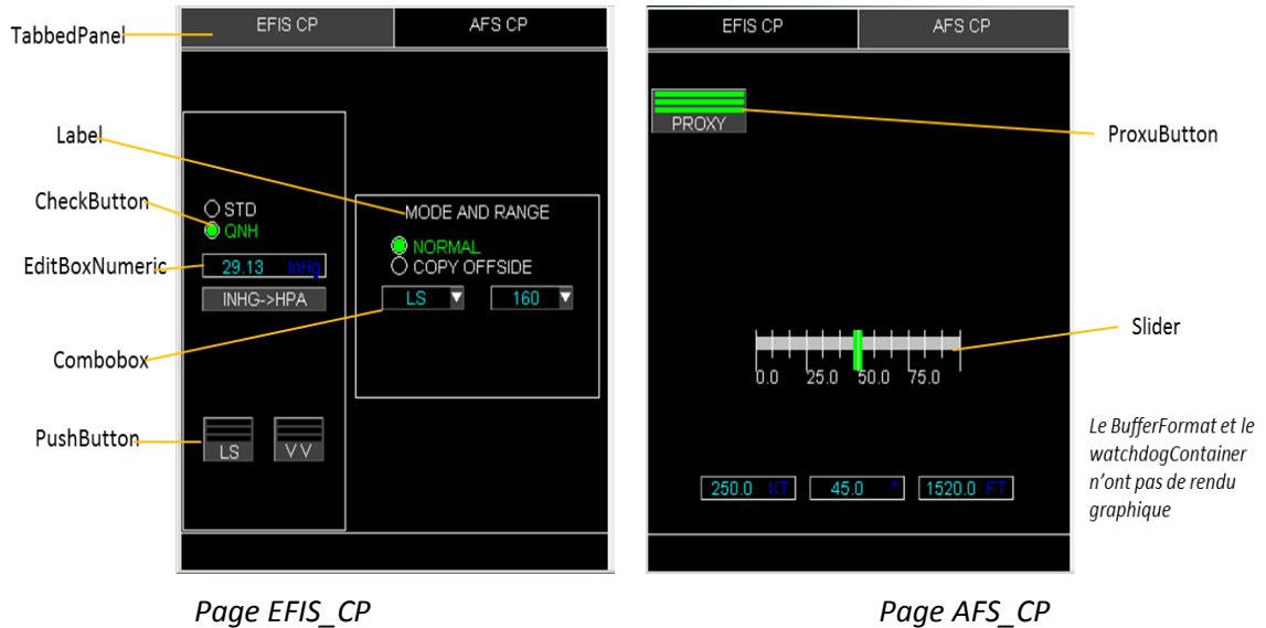
Figure IV.4 Interface de l'étude de cas FCU
