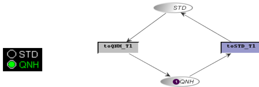
Figure IV.27 Gestion du couple de CheckButton (SDT/QNH) par l'UA FCU
