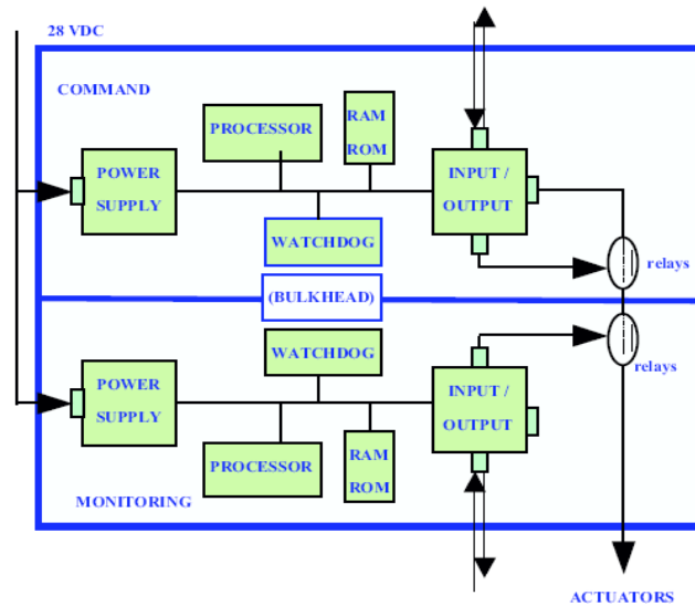
Figure II.35 Schéma simplifié du matériel d'un calculateur de commande de vol Airbus
