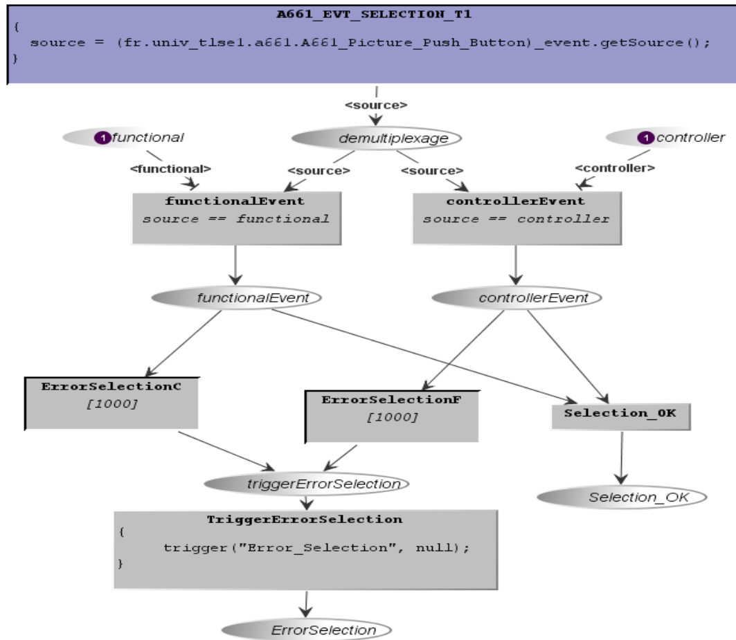
Figure V.15 Comparaison de l'A661_EVT_SELECTION
