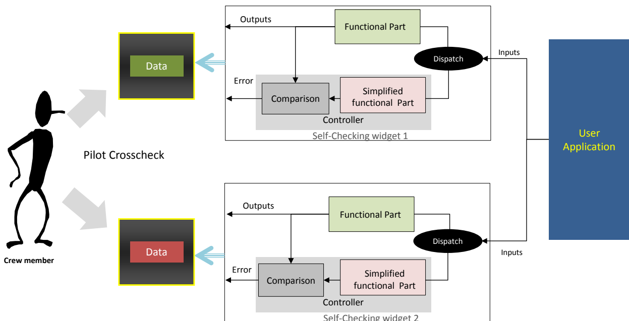
Figure V.18 Architecture du flot d'affichage de l'approche mixte de tolérance aux fautes
