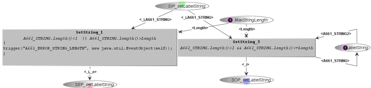
Figure IV.13 Gestion du paramètre LabelString
