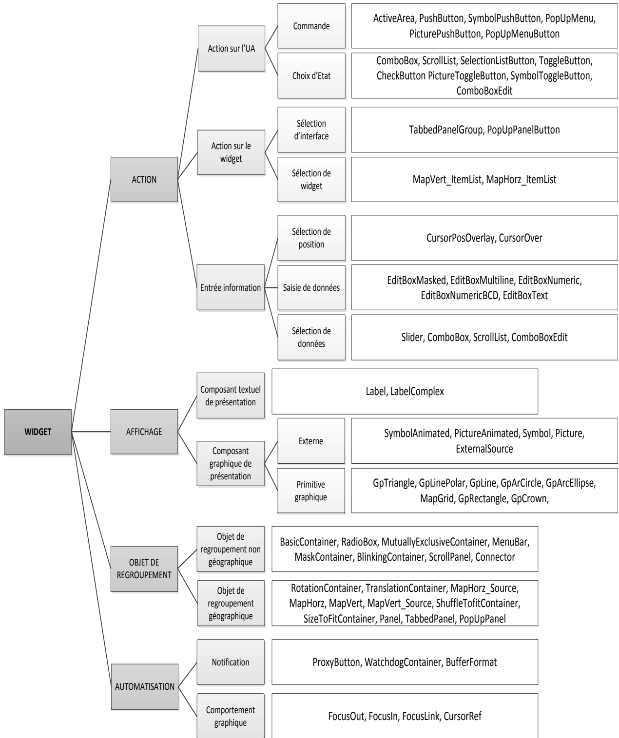
Figure III.11 Typologie des widgets du standard ARINC 661 supplément 3
