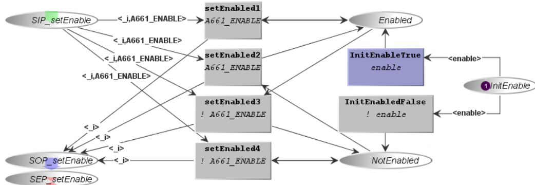
Figure IV.12 Gestion du paramètre Enable
