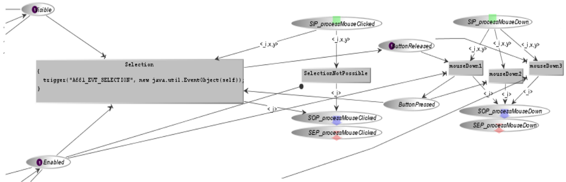
Figure IV.17 Gestion de l'envoi de l'Event du PicturePushButton
