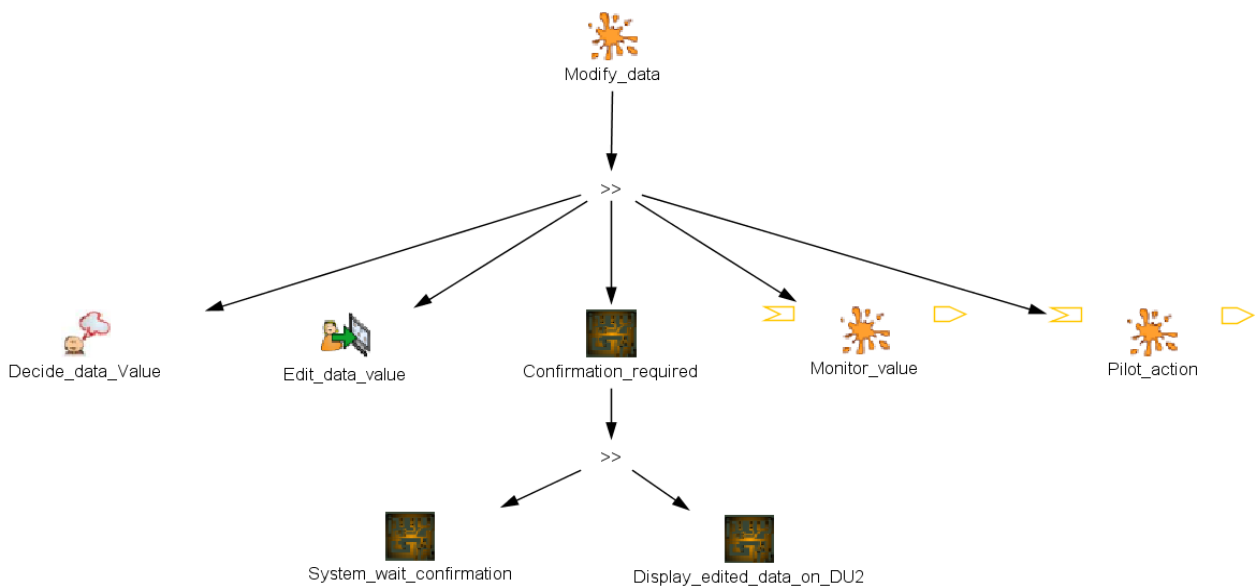
Figure V.20 Modèle de tâche de l'interaction en entrée de l'approche mixte (1)
