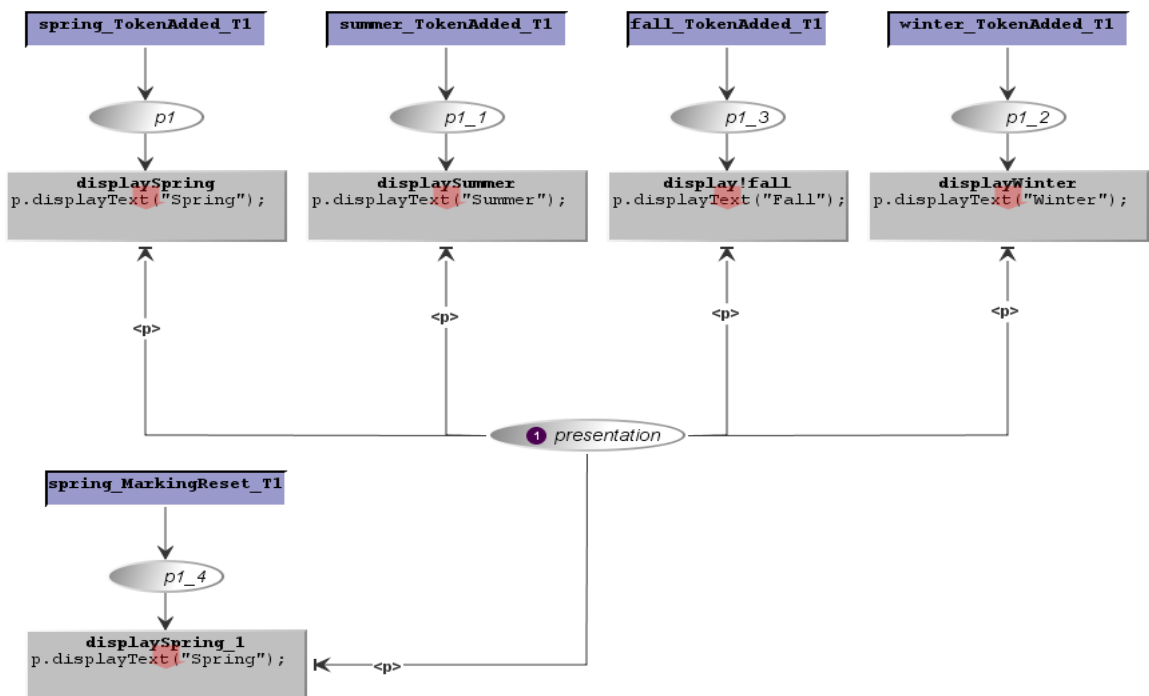
Figure II.22 Réseau de Petri de la fonction de rendu
