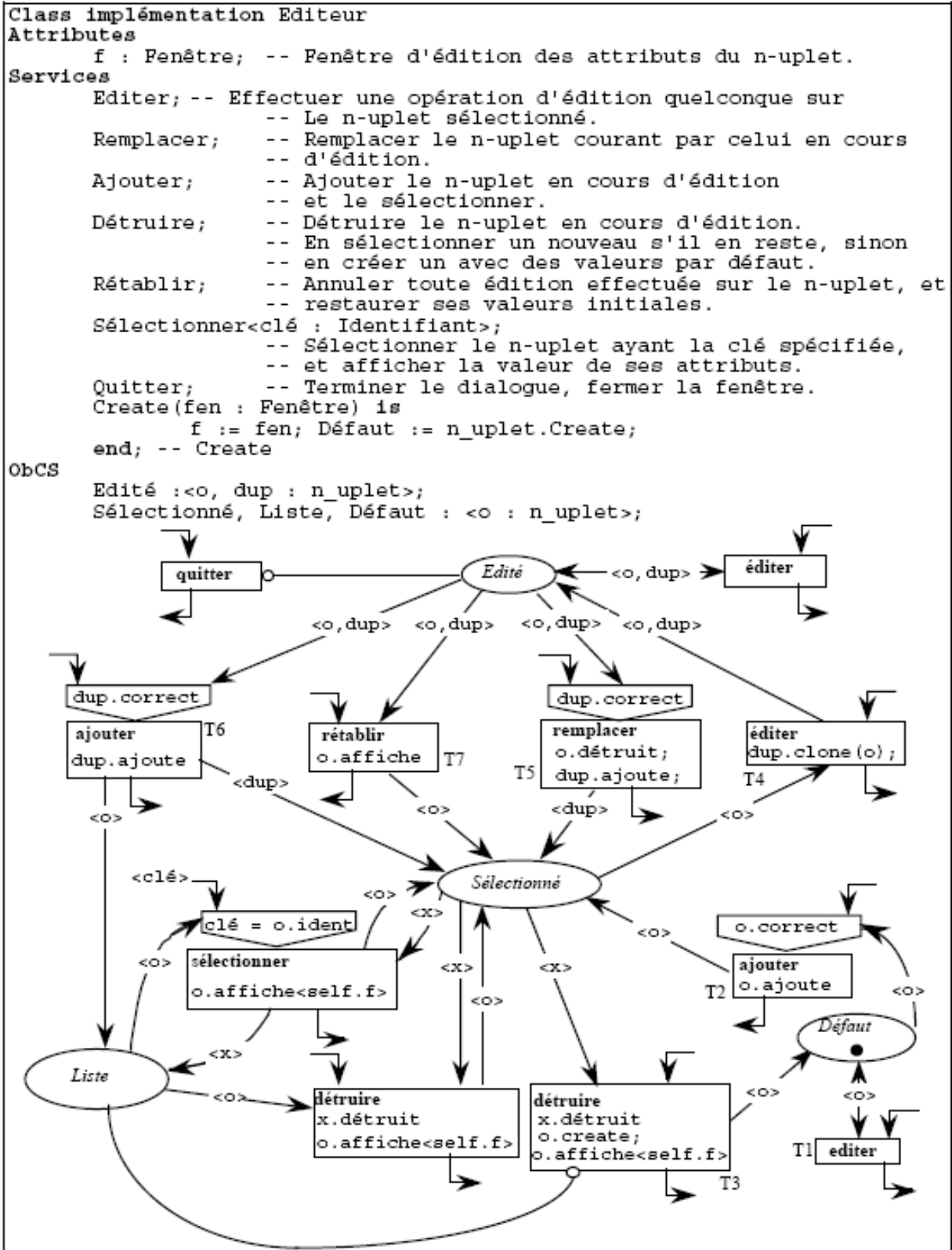
Figure II.10 Implémentation classe Editeur du composant dialogue (Bastide, 1992)
