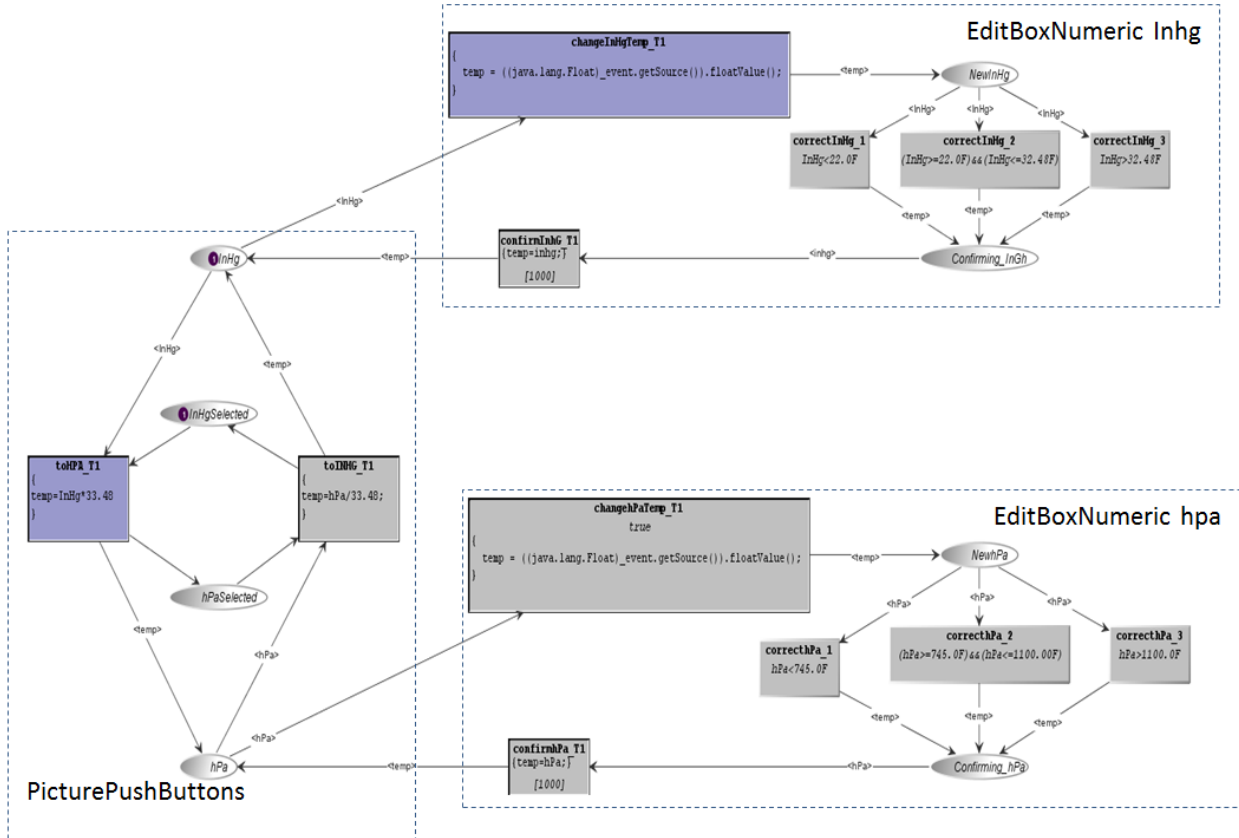
Figure IV.31 Modèle de conversion EditTextNumeric/Pushbutton
