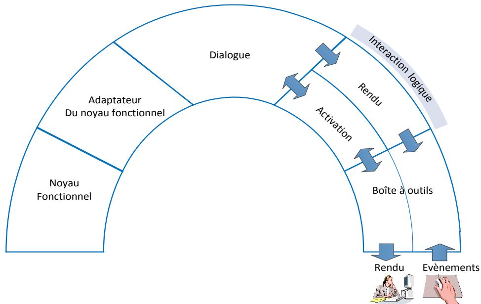
Figure II.19 Représentation sur ARCH des éléments d'ICO
