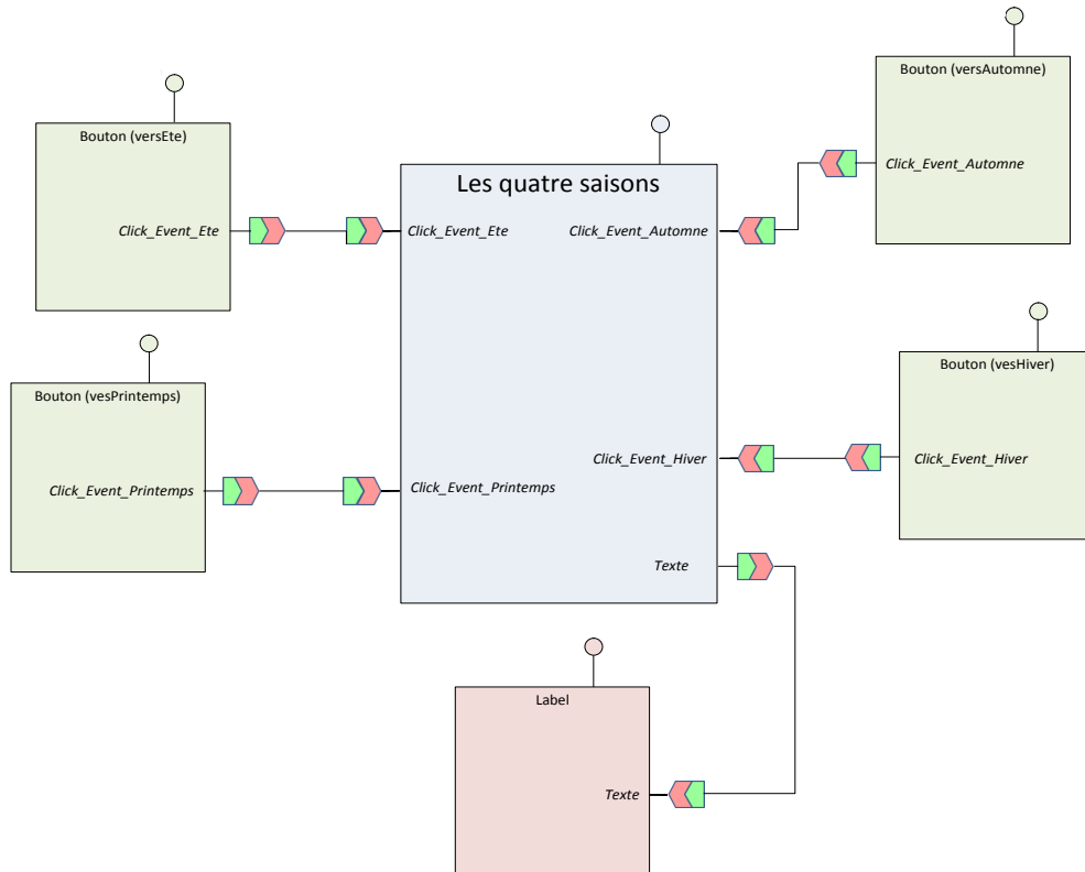
Figure II.26 Assemblage ICompoNet décrivant les 4 saisons
