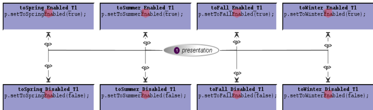
Figure II.23 Réseau de Petri de la fonction d'activation
