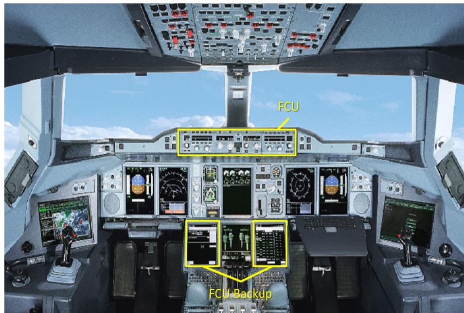
Figure IV.3 Position du FCU et du FCU Backup dans l'environnement du cockpit A380
