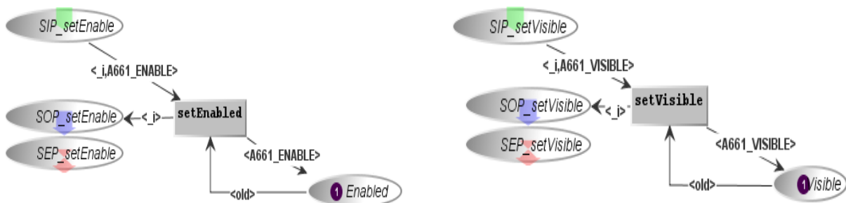
Figure V.12 Gestion des paramètres visible et Enable dans le modèle de la fonction simplifiée
