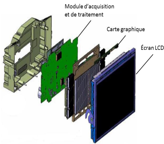
a) Architecture matérielle DU
