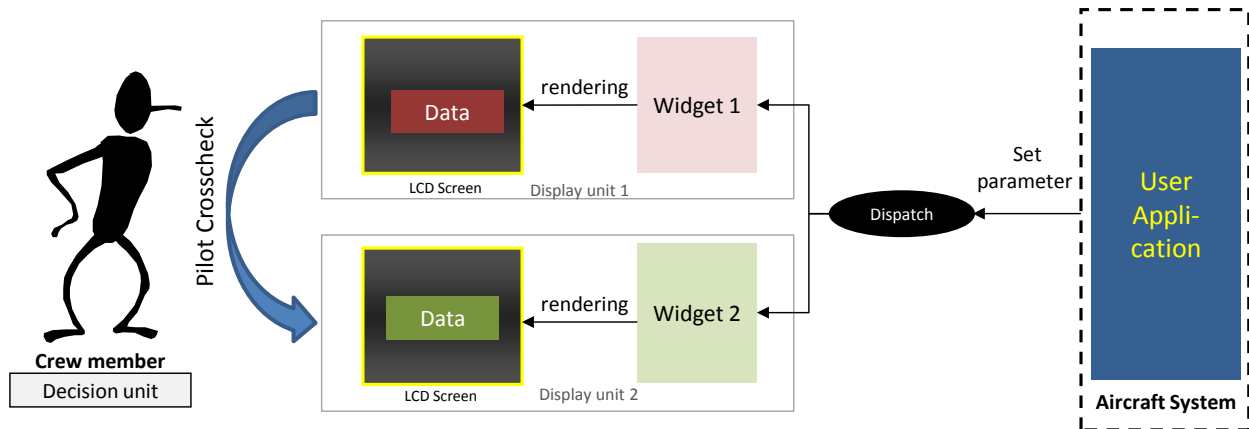
Figure V.1 Architecture de tolérance aux fautes du flot d'affichage reposant sur utilisateur
