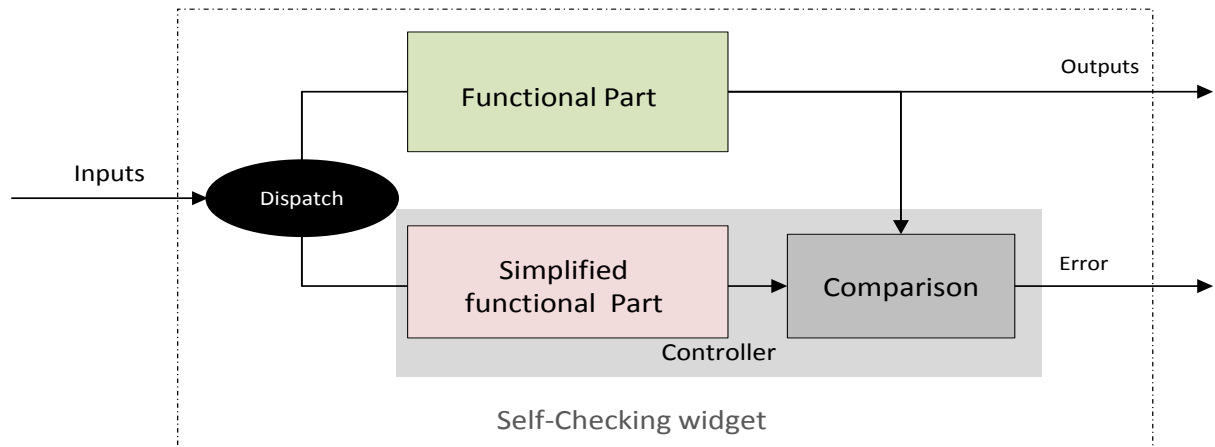
Figure III.19 : modèle de widget autotestable
