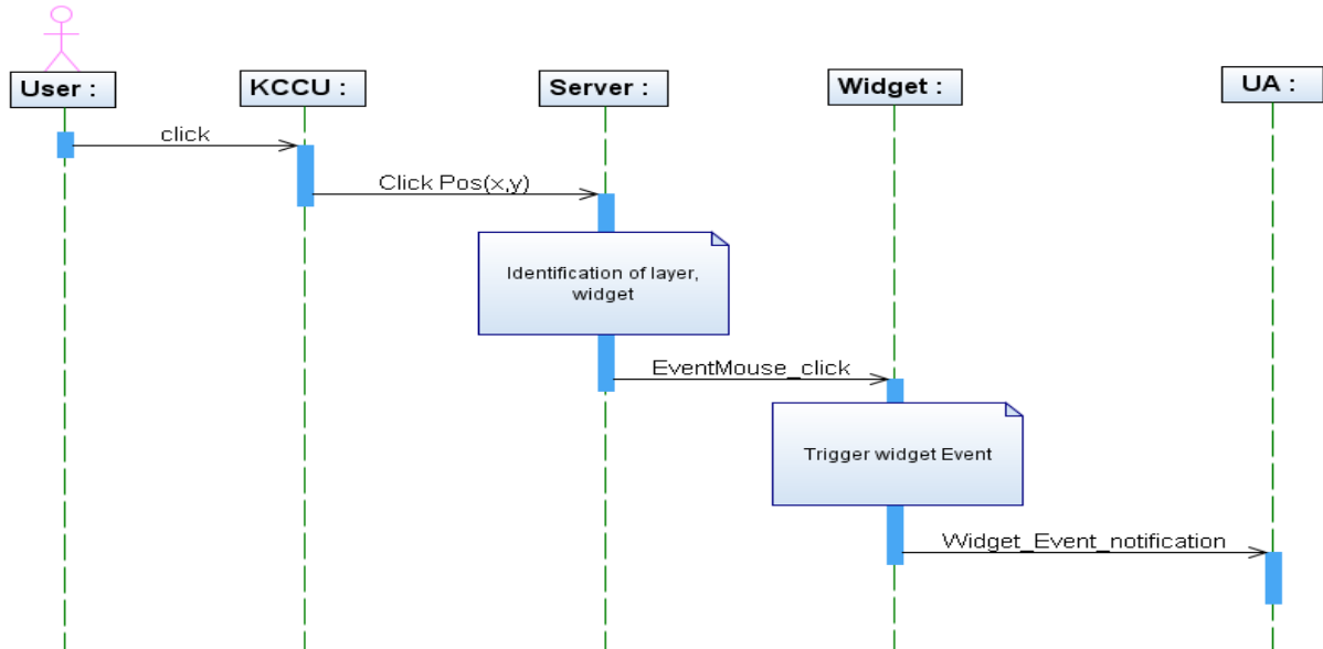
Figure III.4 Diagramme de séquence du flot d'évènements allant du CDS à UA
