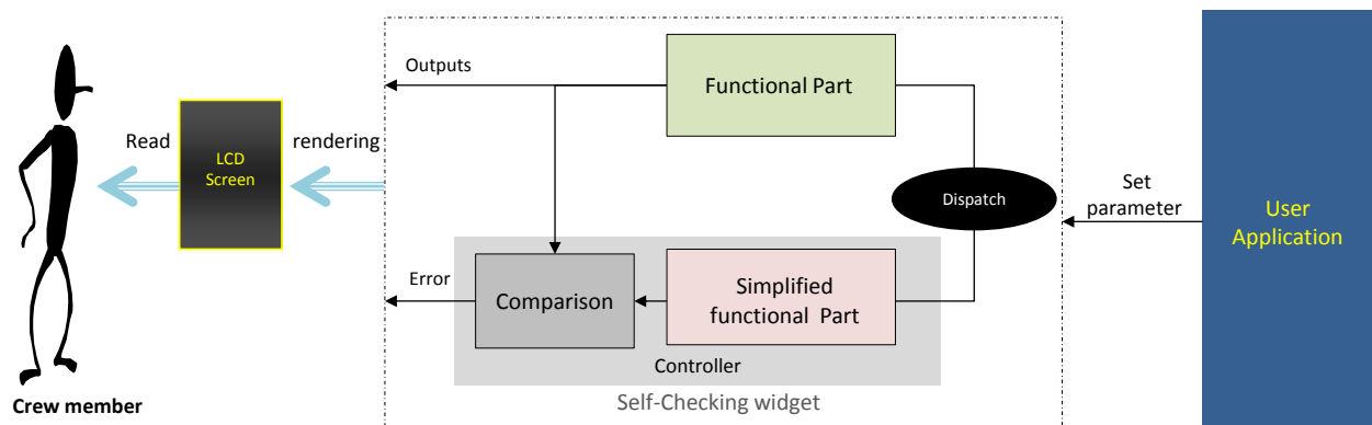
Figure III.21 : Architecture de traitement du flot d'affichage par un widget autotestable
