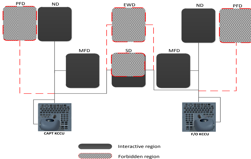
Figure III.7 Zone interactive et non interactive sur le CDS A380
