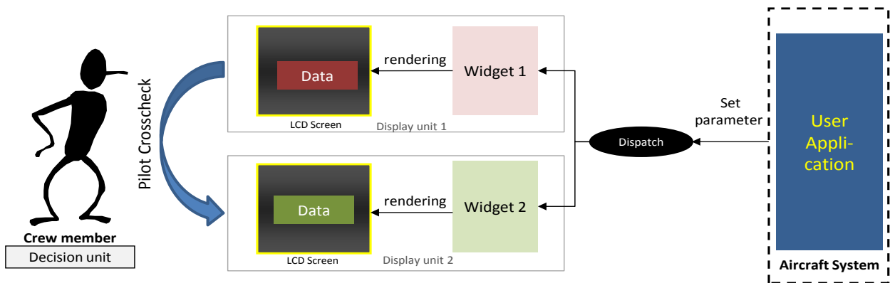
Figure III.18 Intégrité flot d’affichage avec utilisateur
