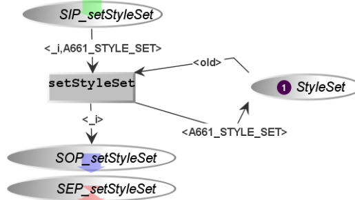
Figure IV.14 Gestion du paramètre Styleset
