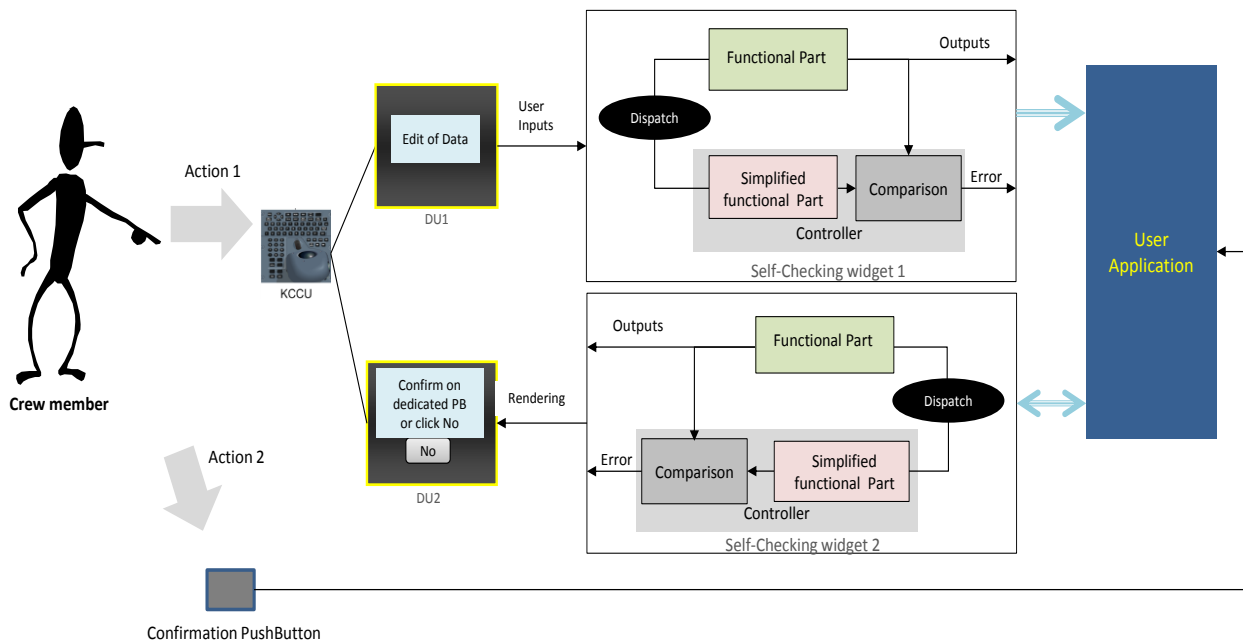
Figure V.19 Architecture du flot de contrôle de l'approche mixte de tolérance aux fautes
