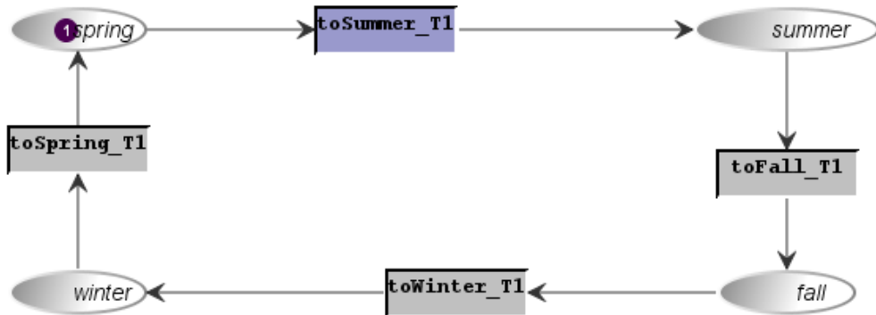
Figure II.21 Réseau de Petri représentant le cycle des saisons
