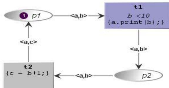
Figure II.12 Réseau de Petri à objets
