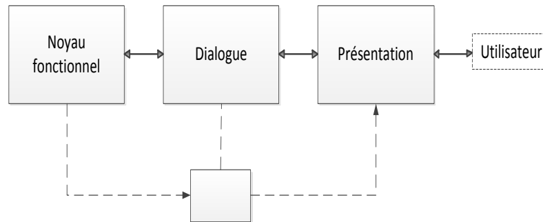
Figure II.2 Modèle d'architecture de seeheim
