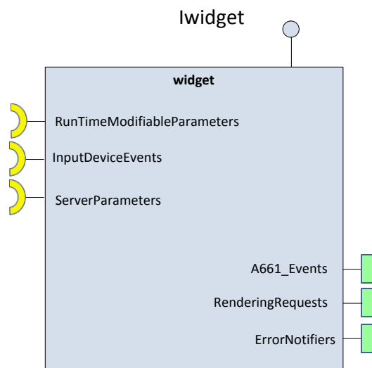
Figure IV.7 Modèle Composant d'un Widget
