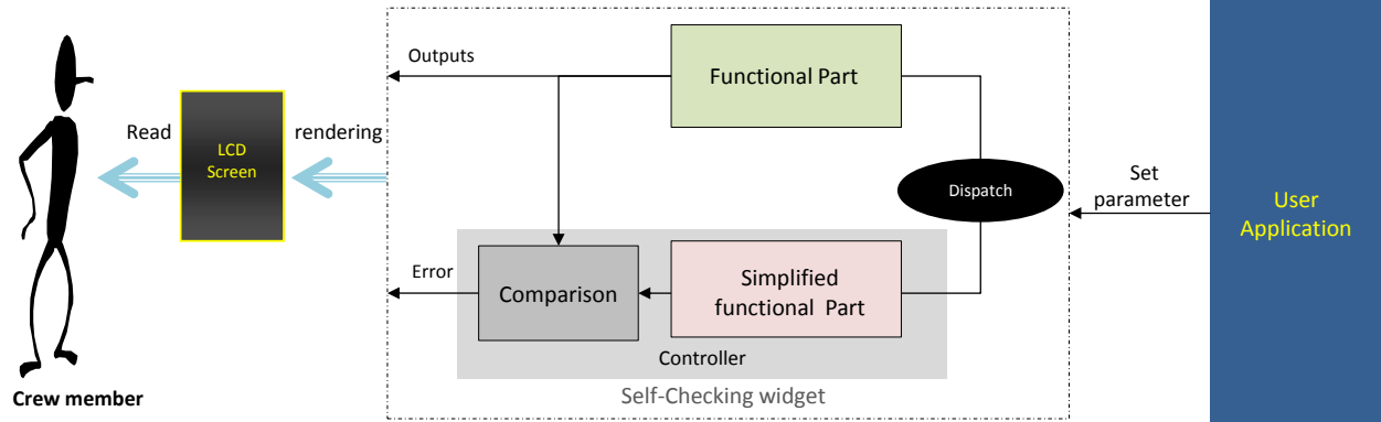
Figure V.10 : Traitement du flot d'affichage par un widget autotestable
