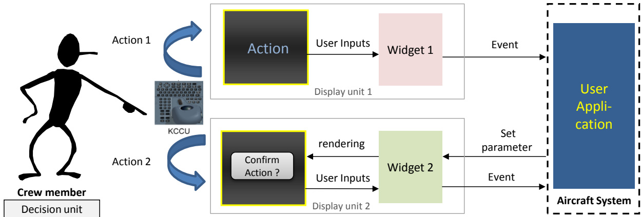
Figure III.17 Intégrité du flot de contrôle
