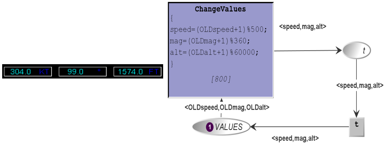
Figure IV.32 Modèle BufferFormat
