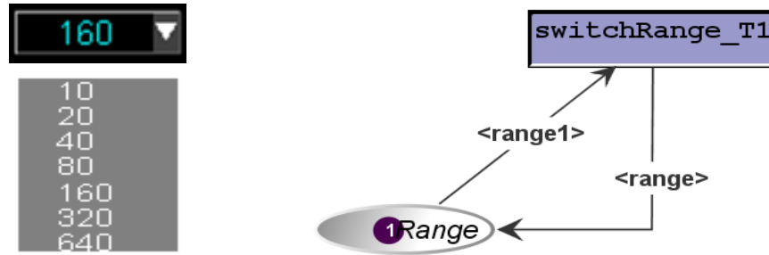
Figure IV.29 Modèle ComboBox
