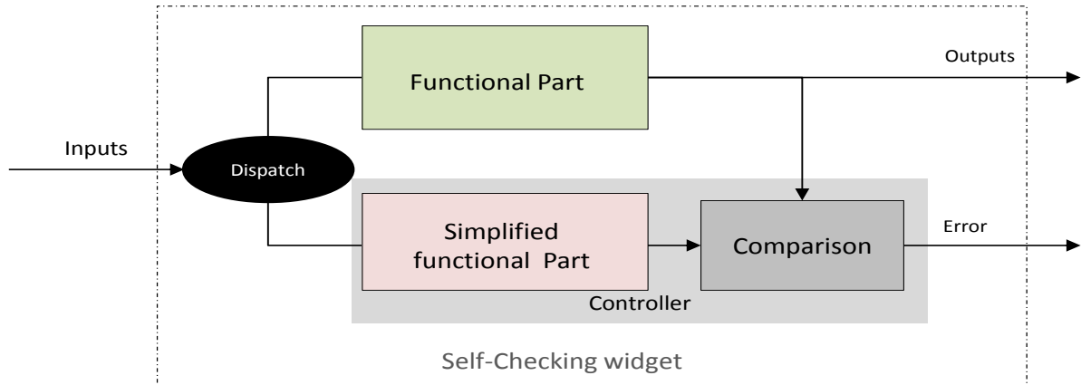
Figure V.8 : Architecture d'un widget autotestable
