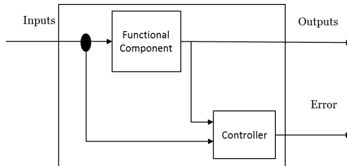
Figure II.34 Structure générale d'un composant autotestable
