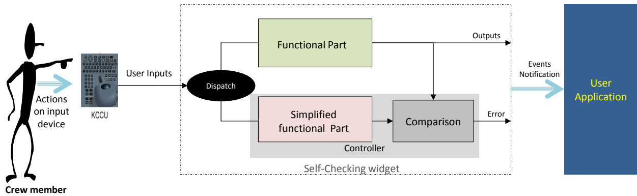
Figure III.20 : Architecture de traitement du flot de contrôle par un widget autotestable
