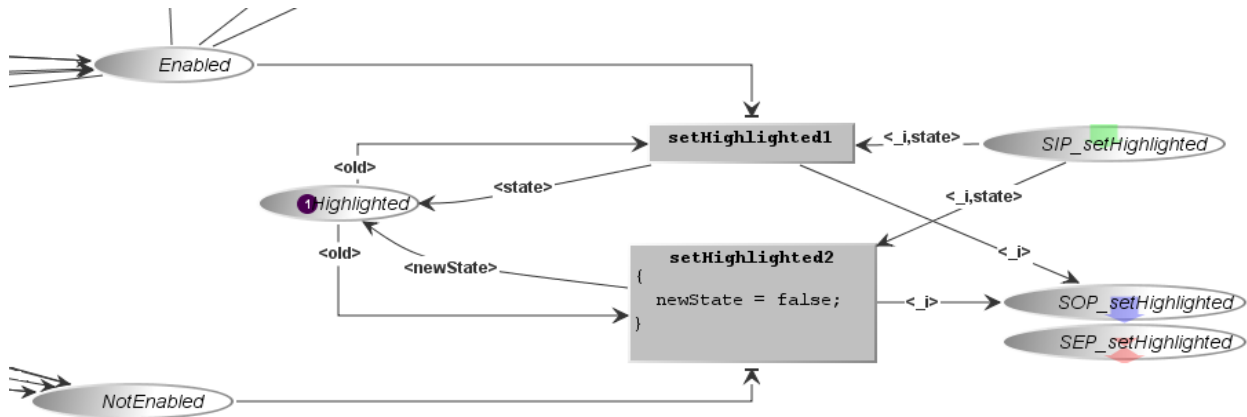
Figure IV.16 Gestion de l'état highlighted en fonction de l'Enable
