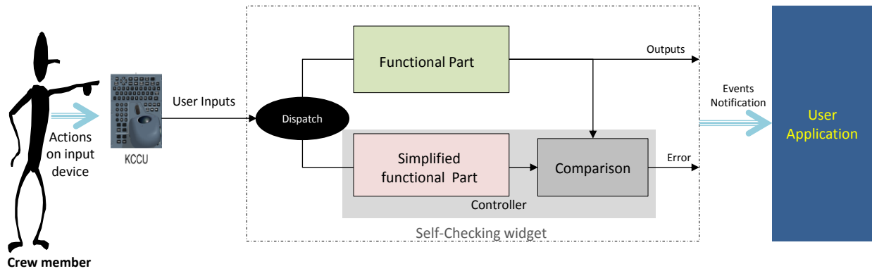
Figure V.9 : Traitement du flot de contrôle par un widget autotestable
