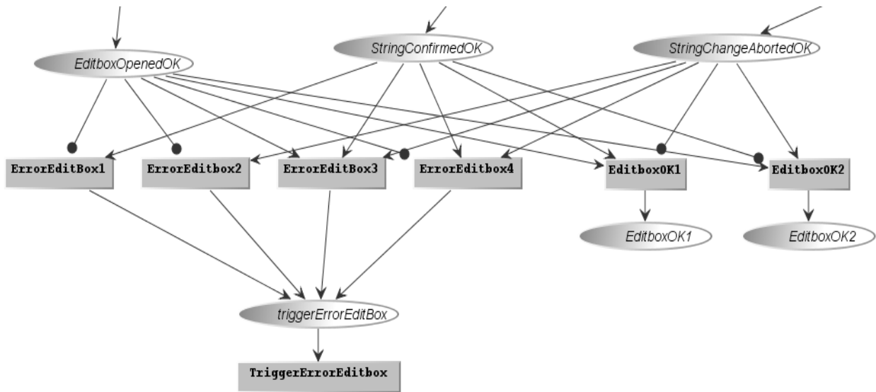
Figure V.17 Comparaison de la séquence des évènements de l'EditBoxNumeric
