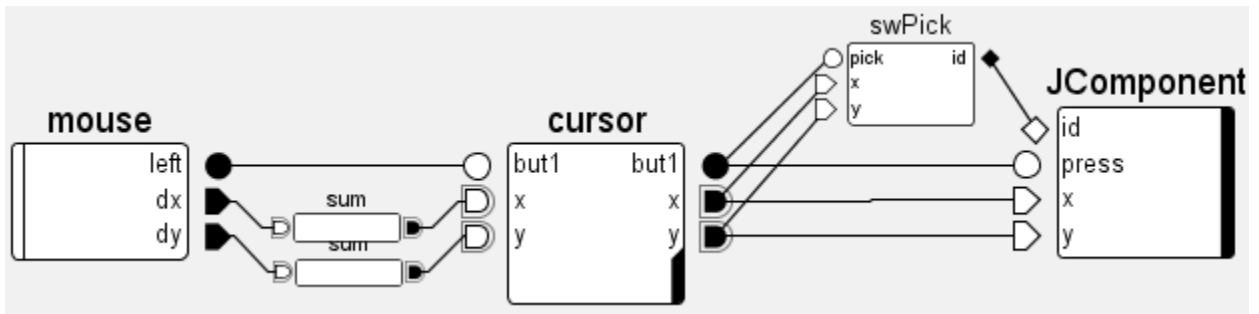
Figure II.6 Contrôle positionnel standard des composants Swing
