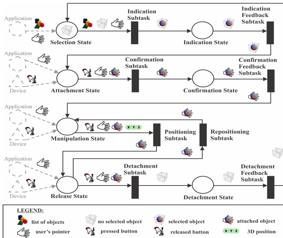
Figure II.9 Réseau de Petri coloré d'un processus d'interaction (Rieder, et al., 2010)
