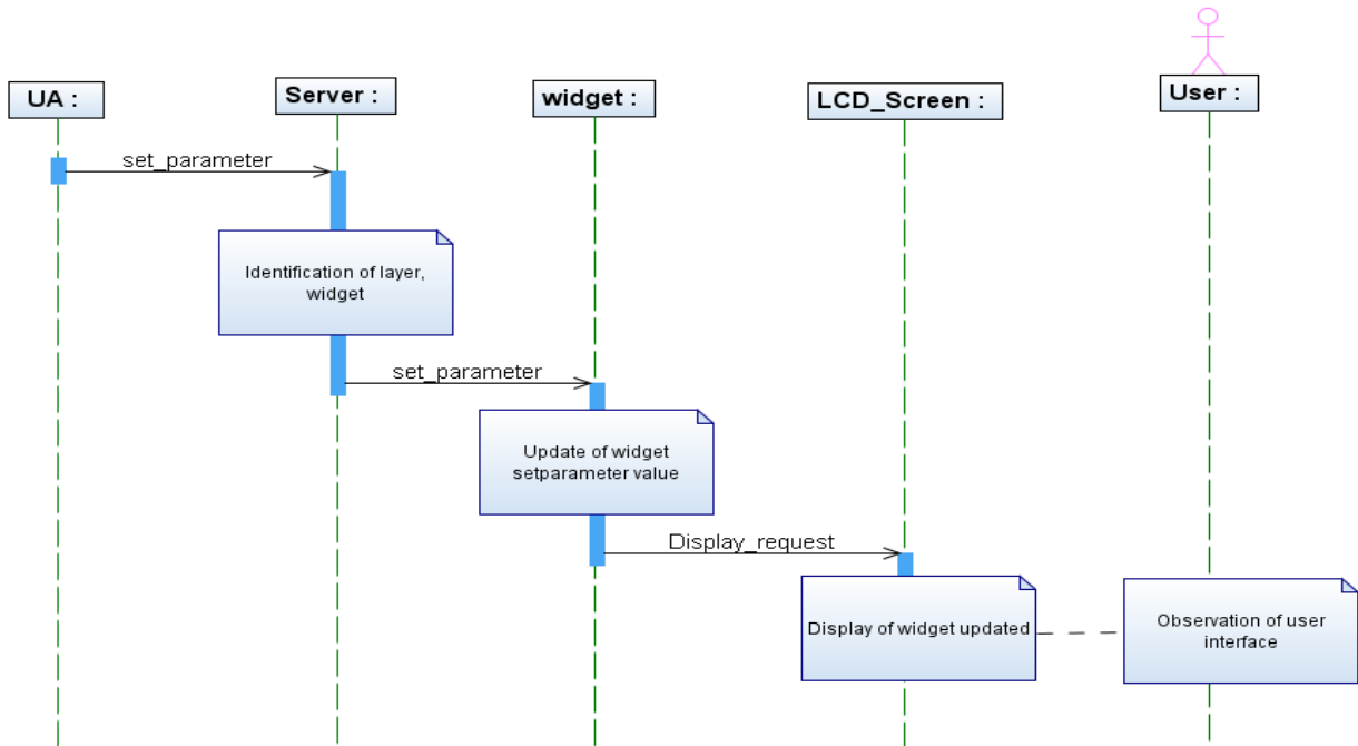
Figure III.5 Diagramme de séquence du flot de données allant de l'UA au CDS
