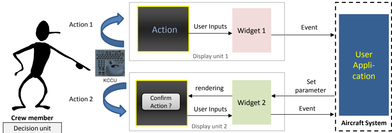
Figure V.3 Architecture de tolérance aux fautes du flot de contrôle reposant sur utilisateur
