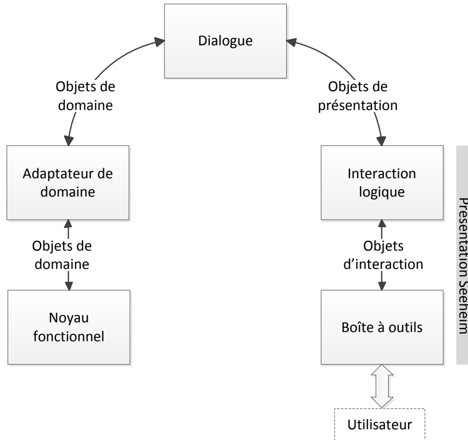
Figure II.3 modèle ARCH/Slinky
