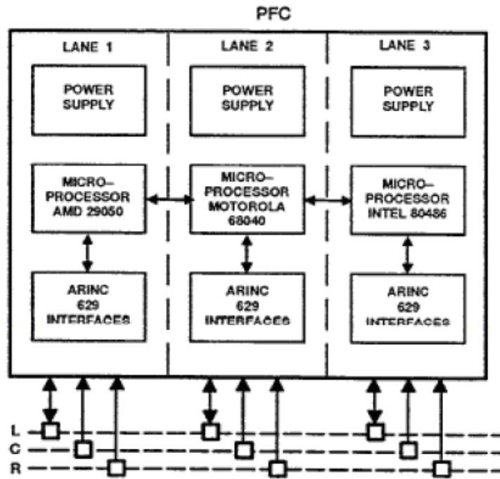
Figure II.36 Schéma simplifié du matériel d'un calculateur de commande de vol Boeing
