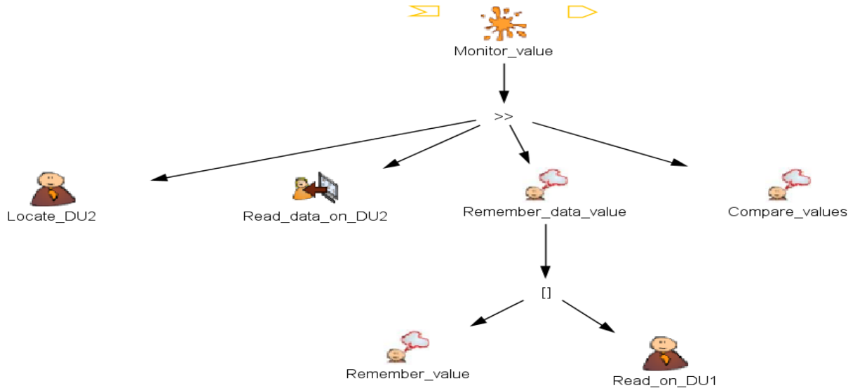
Figure V.5 Modèle de tâche de l'interaction en sortie pour la tolérance aux fautes reposant sur l'utilisateur (2)
