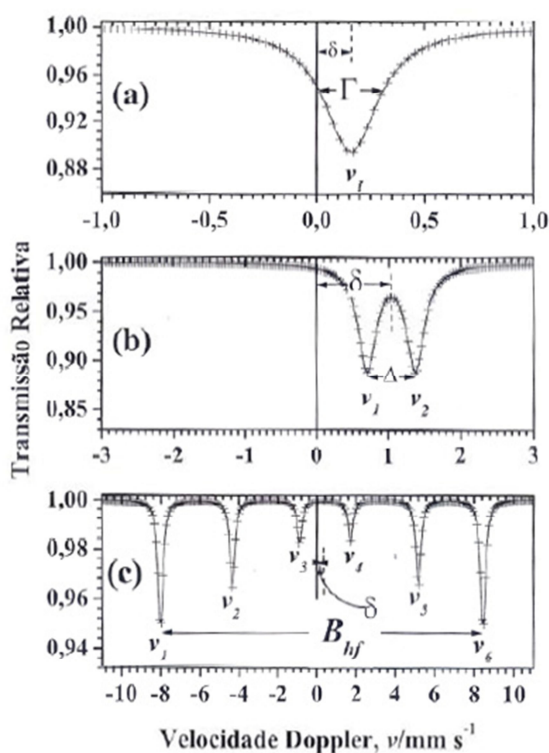
Figura 3.5 Exemplo de espectros Mössbauer para \text{Fe}^{57} (a) apenas o deslocamento isomérico (b) espectro com desdobramento quadrupolar (c) um espectro de uma amostra em estado ordenado com as 6 linhas do campo hiperfino magnético.
