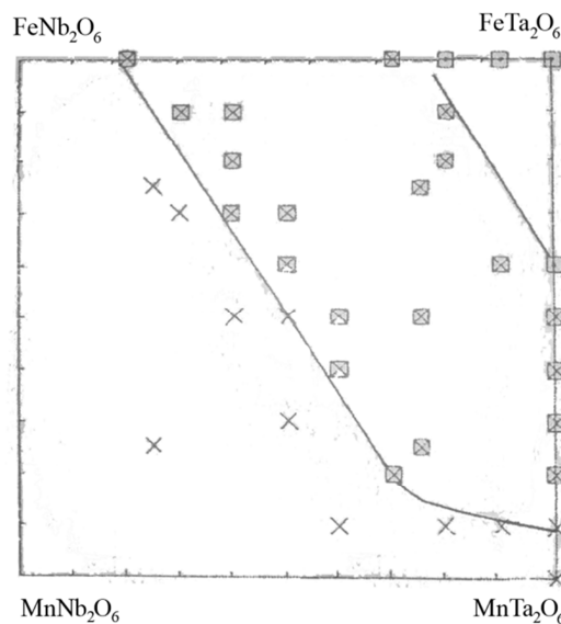
Figura 2.3: Diagrama de fases de amostras sintéticas por Moreau e Tramasure [28]. Os símbolos e X representam tapiolita e columbita, respectivamente.
