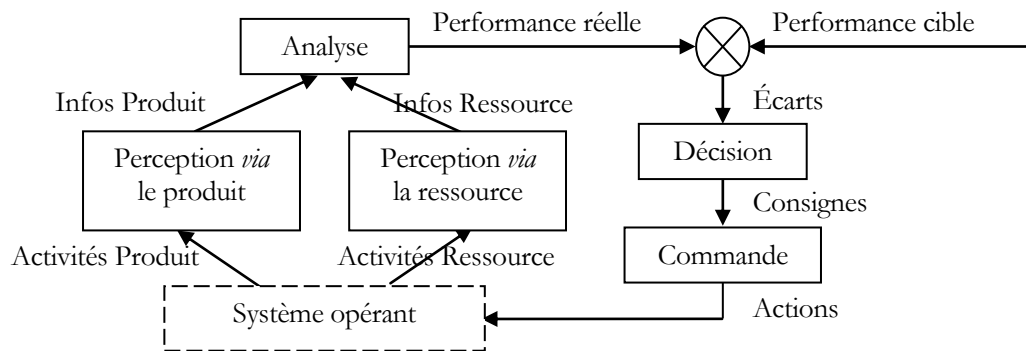
Figure 28. Boucle proprioceptive intégrant le produit intelligent (d'après (McFarlane et al. 2002)).
