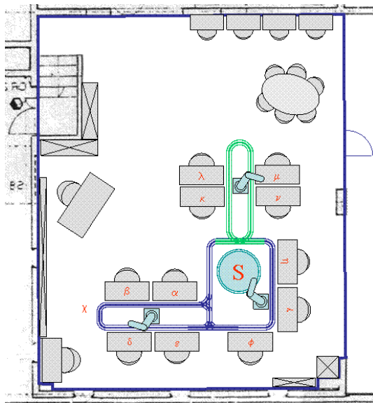
Figure 101 : Plan d'ensemble de la Plateforme Polyvalente de Production et vue d'une boucle de transitique Montrac
