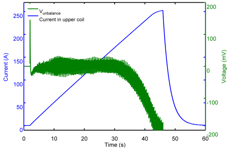
Figure 4-8 : Courant maximal sur la bobine supérieure, avec seuil de transition réglé à 200 mV
