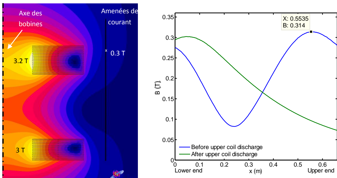
Figure 3-5 : A gauche, Induction magnétique créée par les bobines au courant nominal. A droite, induction magnétique vue par les aménées de courant.
