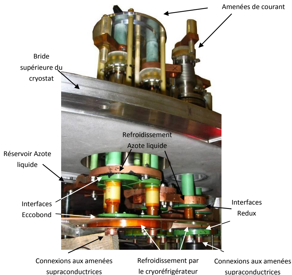
Figure 4-4 : Système d'amenée de courant résistif
