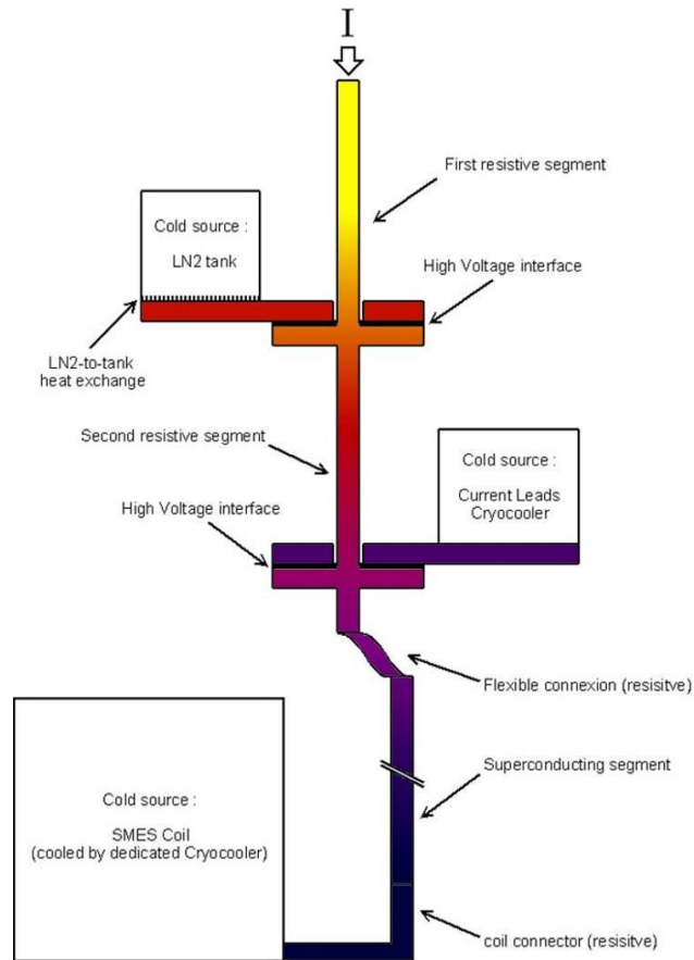
Figure 3-4 : Schéma de principe des Aménées de courant
