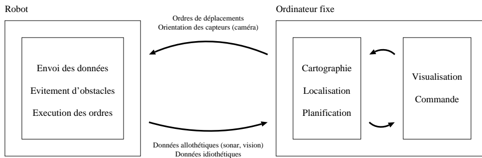
FIG. 6.5: L'architecture que nous avons utilisée pour notre robot est une architecture hybride classique. Un ensemble de comportements réactifs de bas niveau fonctionnant sur le robot permet d'assurer l'exécution des ordres provenant du système de navigation, tout en évitant les obstacles imprévus. Un second niveau fonctionnant sur un autre ordinateur effectue les opérations de cartographie, localisation et planification à partir des données reçues du bas niveau. Un second module fonctionnant sur ce même ordinateur permet de visualiser la carte et de choisir des buts pour le robot.
