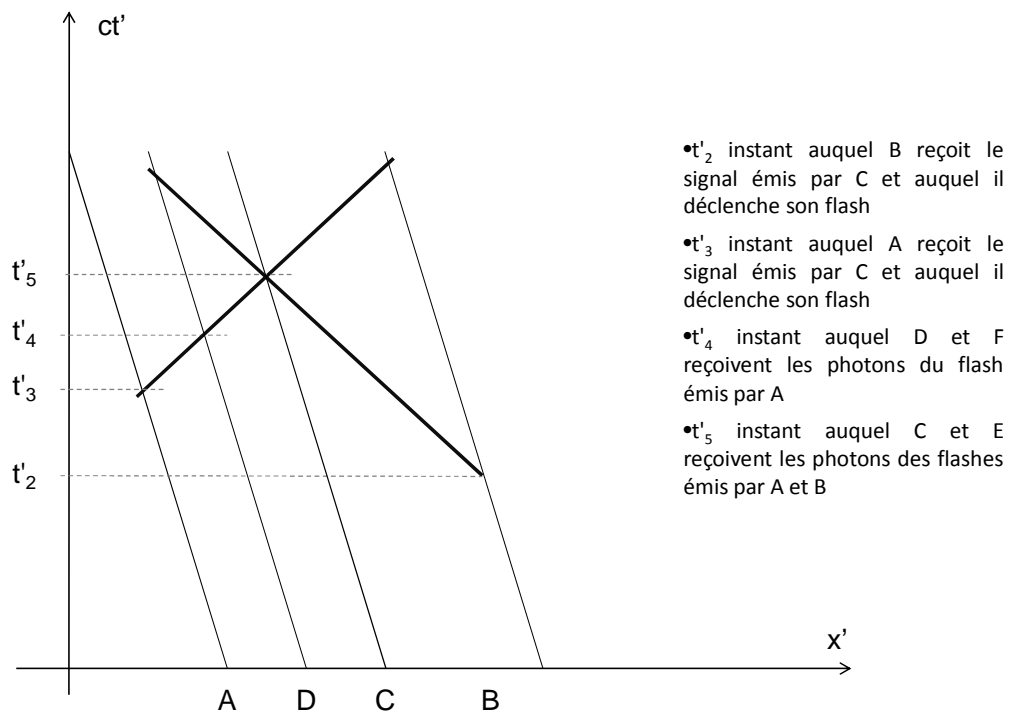
Diagramme d'espace-temps représentant la série des événements E1, E2, E3, E4 et E5 et permettant de répondre aux items I2.5, I2.6, I2.7 et I2.8. Les traits épais représentent les lignes d'univers des photons, les lignes fines représentent les lignes d'univers de A, B, C et D dans le référentiel de E et F.
