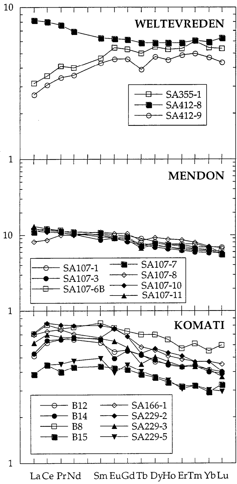
Figure 6: Spectres de Terres Rares normalisés aux chondrites (Evensen et al., 1978) représentant les roches totales des komatiïtes des trois formations.
