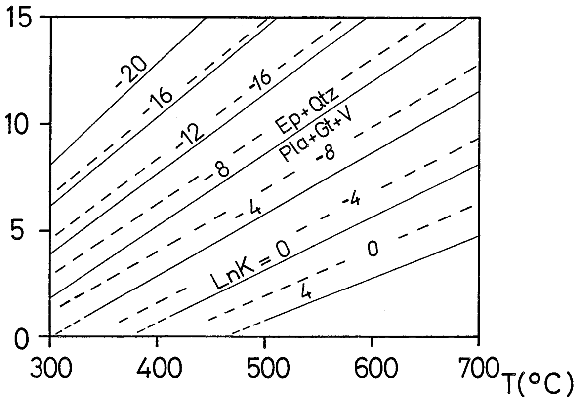
Fig. 76 : Contours d'iso-LnK de l'équilibre R15 calculés en utilisant les paramètres thermodynamiques des pôles purs de Powell et Holland (1985) (trait continu) et d'Helgeson et al. (1978) (trait discontinu).
