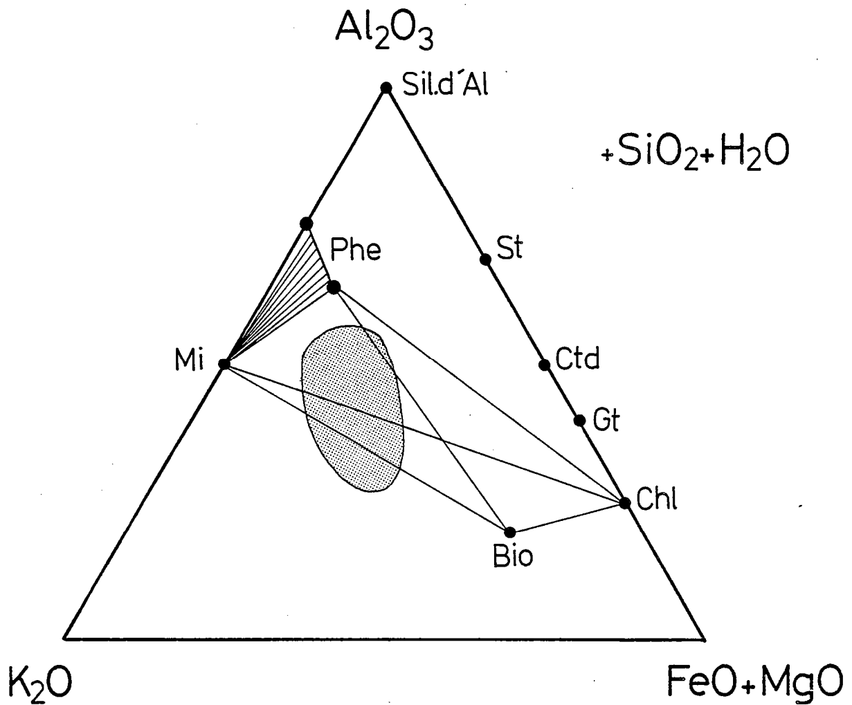
Fig. 2 : Projection dans le diagramme AKF des phases phengite, microcline, biotite, chlorite, grenat, cordiérite, chloritoïde, staurotide, silicate d'alumine. H_2O et Qtz sont en excès. Le champ en grisé représente dans ce diagramme, la position des roches de composition granitique et granodioritique.
