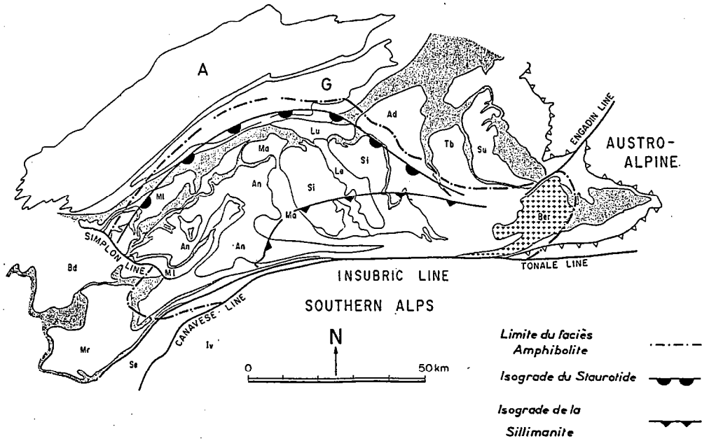
Fig. 24 : Carte géologique simplifiée des Alpes centrales montrant la répartition des isogrades du staurotide et de la sillimanite dans les Alpes centrales d'après Niggli (1970). Dans le domaine pennique, les roches de couverture (domaine grisé) sont intercalées avec des nappes de socle (Ad: Adula, An: Antigorio, Le: Leventina, Lu: Lucomagno, Ma: Maggia, Mi: Monte Leone, Mr: Mont Rose, Se: Sesia, Su: Suretta, Tb: Tambo). Au Nord du dôme lépontin, sont représentés les massifs cristallins externes de l'Aar (A) et du Gotthard (G). Au Sud, les lignes insubrienne et du Canavese séparent la zone pennique du domaine austroalpin comprenant la zone d'Ivrea (Iv). L'intrusion de Bergell (Ber) est également figurée. Modifié d'après Merle et al. (1988).
