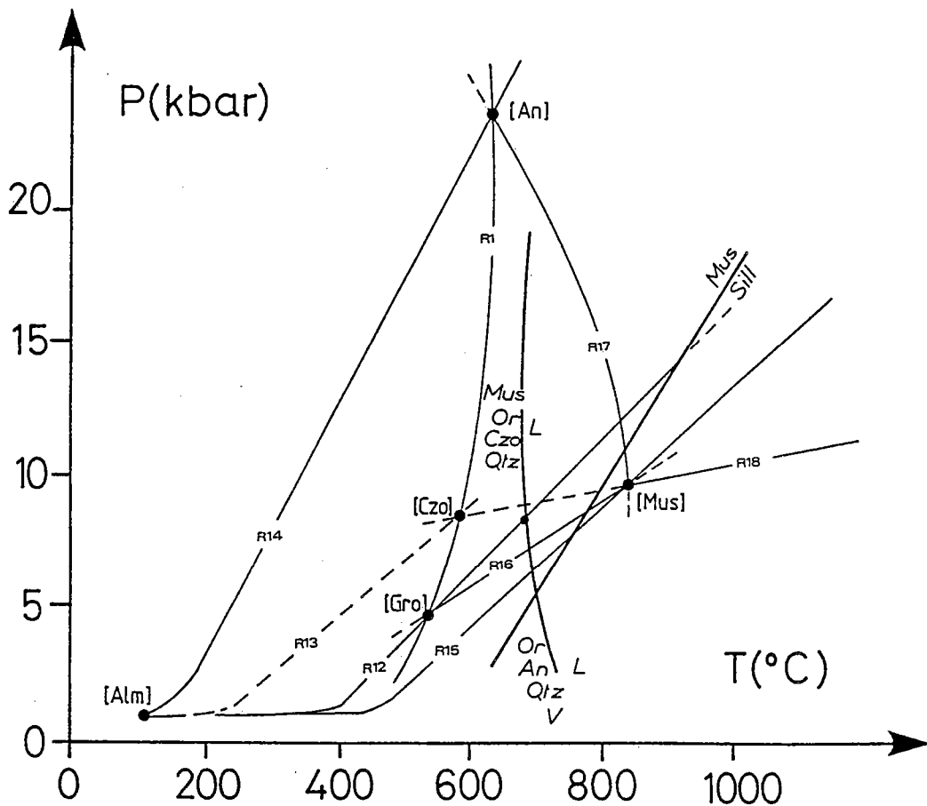
Fig. 50 : Courbes de fusion partielle dans le système \text{Na}_2\text{O}-\text{K}_2\text{O}-\text{CaO}-\text{Al}_2\text{O}_3-\text{SiO}_2-\text{H}_2\text{O} d'après Johannes (1984). Les courbes de fusion \text{Pl} + \text{Or} + \text{Qtz} + \text{V} = \text{L} sont fonction de la composition du plagioclase. A basse pression, la courbe de fusion partielle se déplace d'environ 70^\circ\text{C} vers les hautes températures d'un plagioclase de composition albitique à une anorthite pure.
