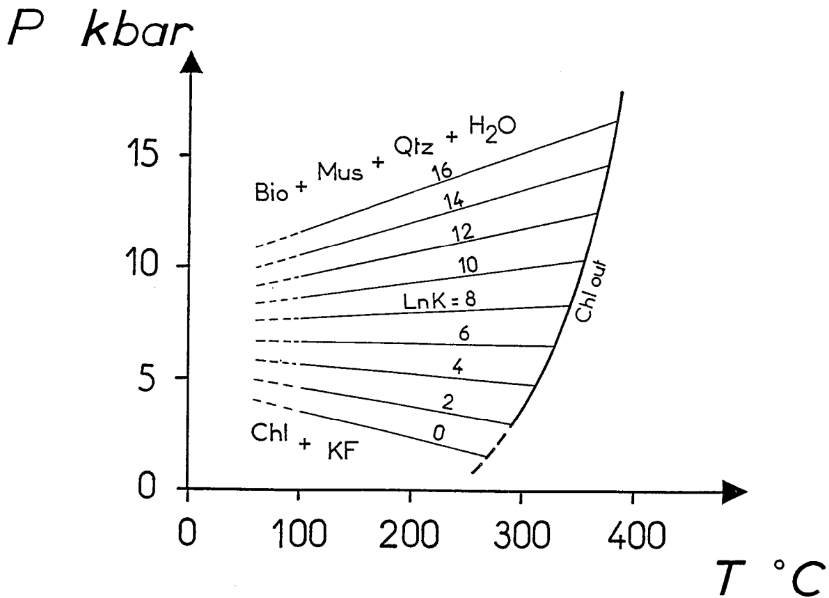
Fig. 71 : Contours d'iso- \text{Ln}K de l'équilibre R_{22}: 3\text{Clin} + 8\text{FK} = 3\text{Mus} + 5\text{Phl} + 9\text{Qtz} + 4\text{H}_2\text{O} , calculés en utilisant les paramètres thermodynamiques des pôles purs de Powell et Holland (1985). La courbe Chl déterminée expérimentalement par Massonne et Schreyer (1987) représente l'équilibre R_6 pour différentes valeurs de la substitution phengitique.
