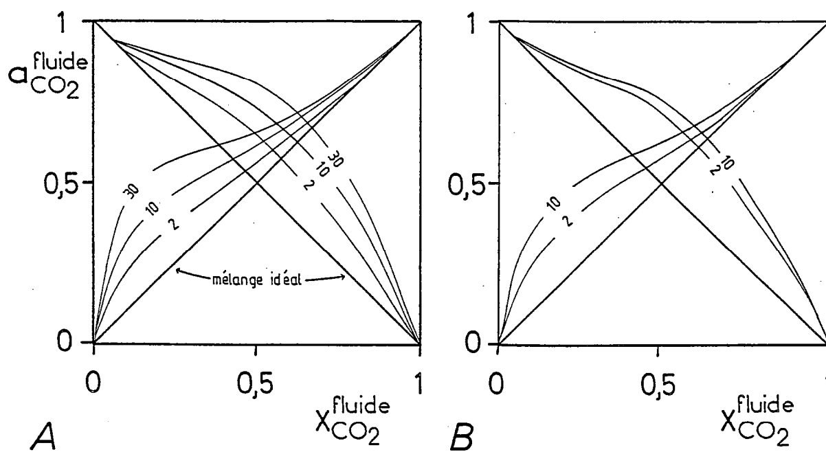
Fig. 15 : Diagramme a_{\text{H}_2\text{O}}-X_{\text{H}_2\text{O}} calculé à 500°C et 2, 10, 30 kbar d'après Kerrich et Jacobs (1981) (A) et Powell et Holland (1985) (B) montrant la non-idéalité de la solution \text{CO}_2\text{-H}_2\text{O} .
