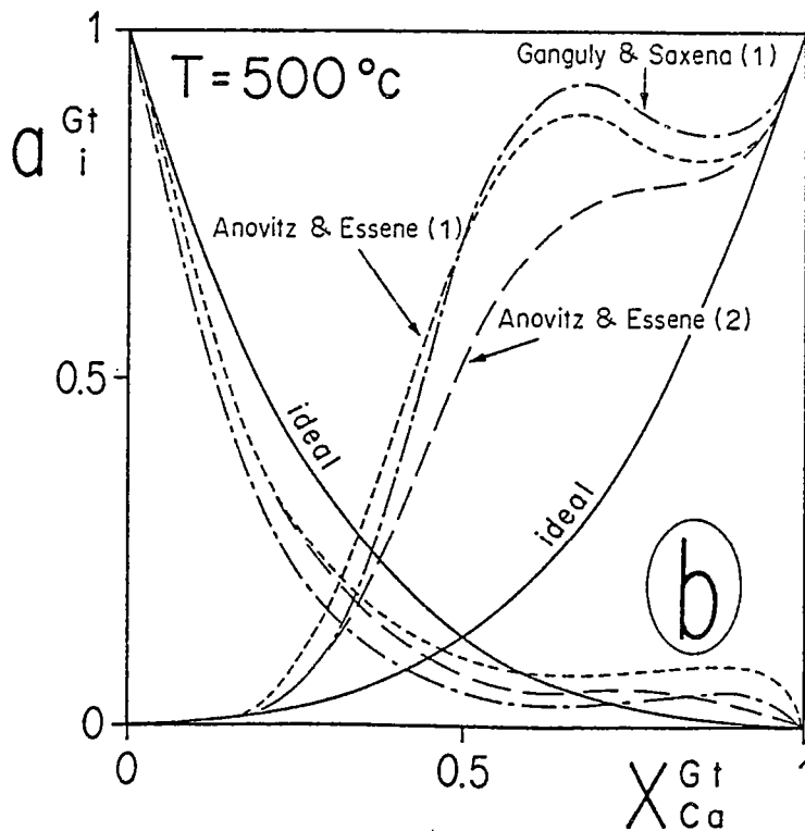
Fig. 7 : Diagramme a_i-X_i dans le grenat ( i = \text{Ca-Fe} ) calculé à 500^\circ\text{C} d'après les modèles pour lesquels W_s = 0 modèles de Geiger et al. (1967) et Ganguly et Saxena (1964, 2 d modèle) (A) et d'après les modèles pour lesquels W_s = 0 , modèles de Ganguly et Saxena (1964, 1 er modèle) et Anovitz et Essene (1967, modèles 1 et 2) (B).
