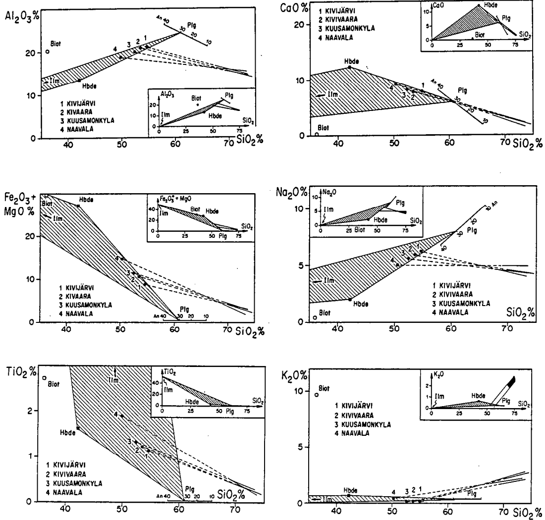
Fig. 10-16 : Diagrammes oxyde = f(\text{SiO}_2) pour \text{Al}_2\text{O}_3 (a) ; (\text{Fe}_2\text{O}_3 + \text{MgO}) (b) ; \text{TiO}_2 (c) ; \text{CaO} (d) ; \text{Na}_2\text{O} (e) et \text{K}_2\text{O} (f). La composition des minéraux constituant le cumulat a été figurée : Biot = biotite; Hbde = hornblende; Plg = plagioclase; Ilm = ilménite. Les droites représentent les lignes de différenciation des massifs de TTG et les points noirs, la composition calculée des cumulats (1 = Kivijärvi; 2 = Kivivaara; 3 = Kuusamonkylä; 4 = Naavala).
