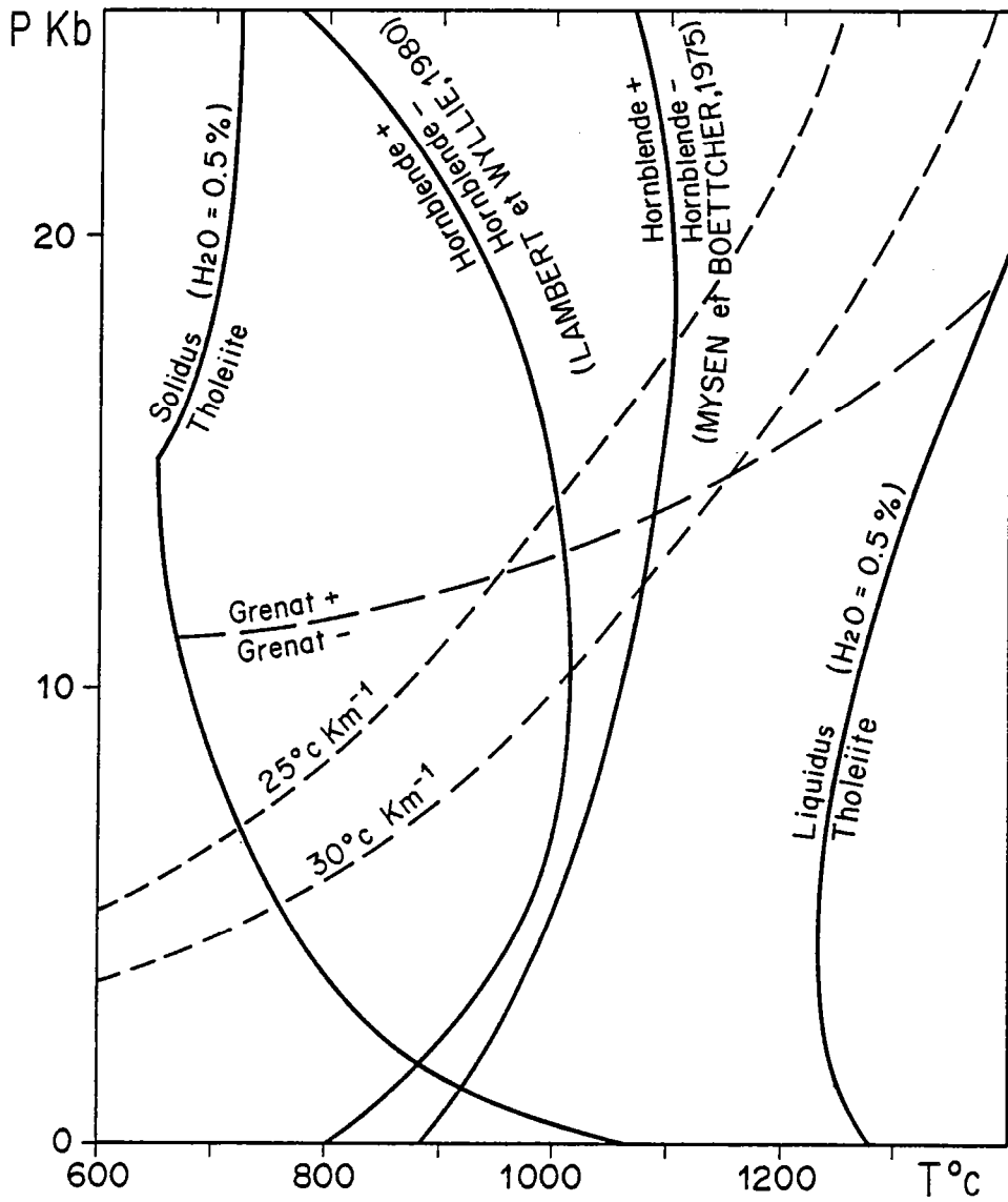
Fig.15-1 : Diagramme P = f (T) dans lequel ont été représentés le solidus et les liquidus d'une tholéiite hydratée (Wyllie, 1971 ; Stern et al., 1975) ainsi que les domaines de stabilité du grenat et de la hornblende. Les gradients géothermiques de 25°C km -1 et 30°C km -1 ont aussi été figurés, seuls des gradients inférieurs à 30°C km -1 peuvent permettre la fusion d'une tholéiite alors que le grenat et la hornblende sont présents au résidu.
