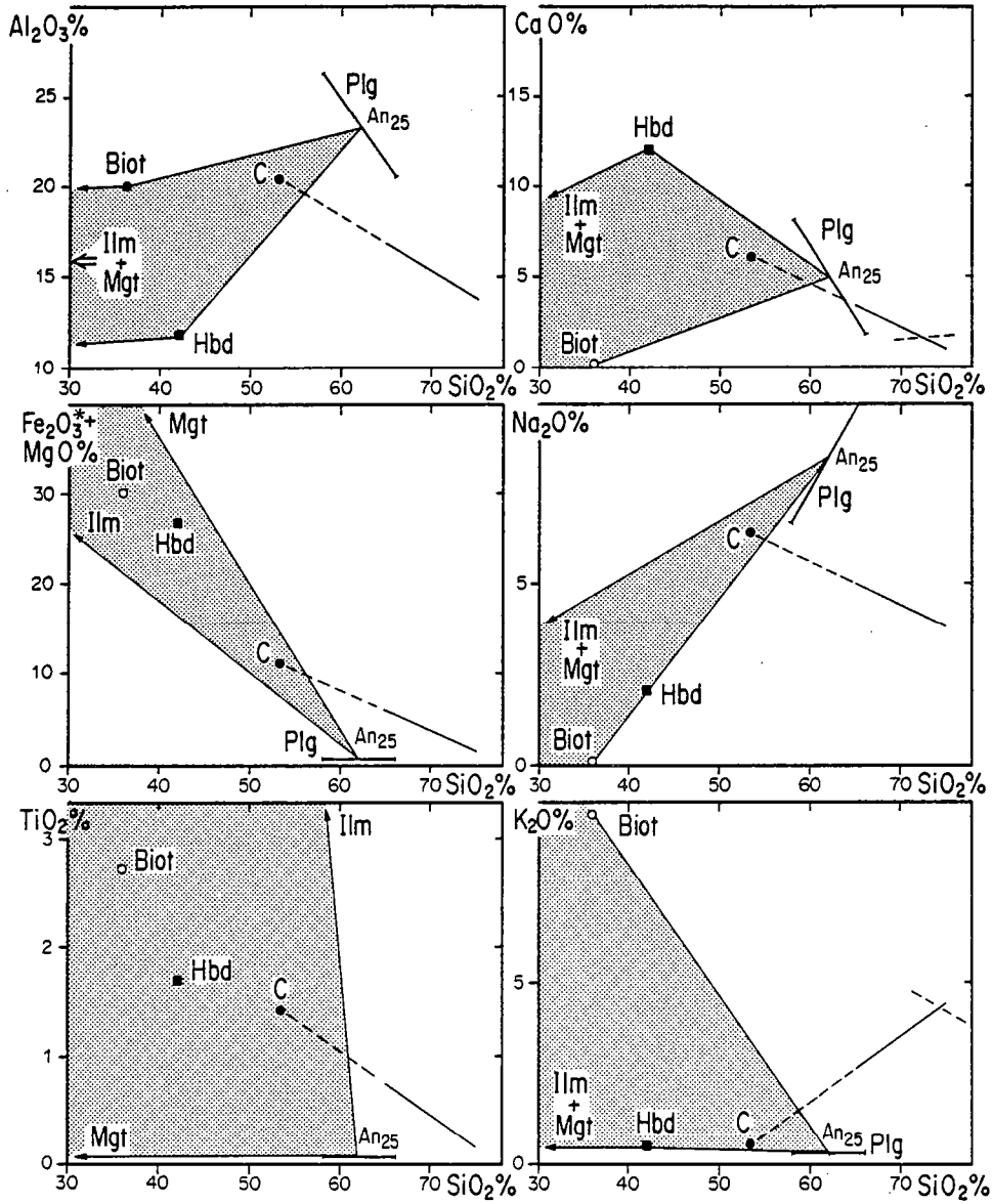
Fig. 12-16 : Diagrammes Oxyde = f ( SiO_2 ) dans lesquels la composition des minéraux constituant le cumulat (c) a été figurée : Biot = biotite ; Hbd = hornblende Plg = Plagioclase ; Ilm = ilménite ; Mgt = magnétite. Le segment de droite représente la lignée de différenciation des granodiorites et des granites gris.
