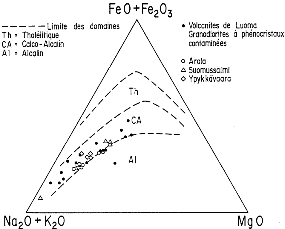
Fig. 13-2 : Diagramme A-F-M (Kuno, 1968) montrant le caractère calco-alcalin des volcanites acides de Luoma et leur ressemblance avec les granodiorites à phénocristaux contaminées.
