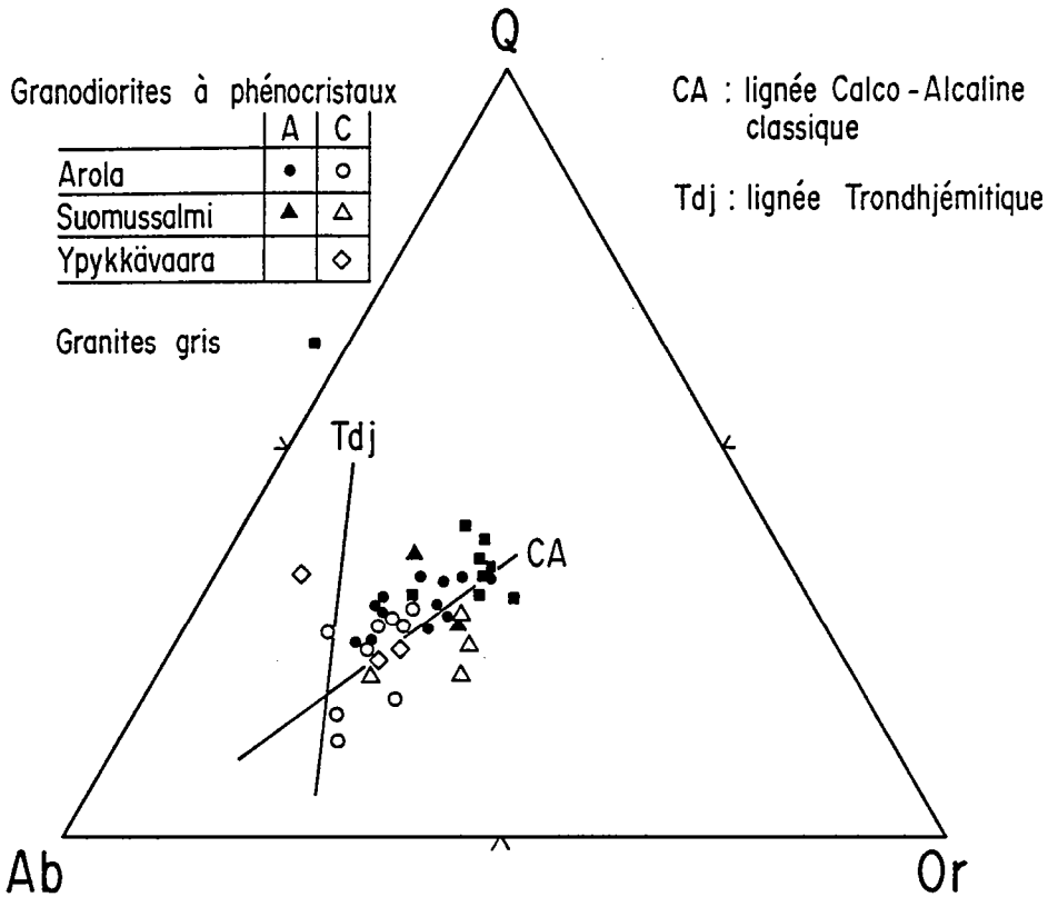
Fig. 12-5 : Diagramme Q - Ab -Or d'après Barker et Arth (1976) permettant de distinguer les lignées trondhjémétiques des lignées calco-alcalines classiques.
