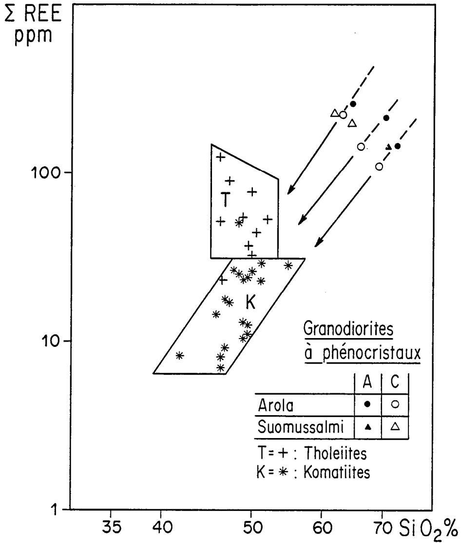
Fig. 12-12 : Diagramme Log ( \Sigma REE) = f (Log (SiO 2 )) montrant l'influence de l'assimilation de komatiites sur la composition des magmas granodioritiques.
