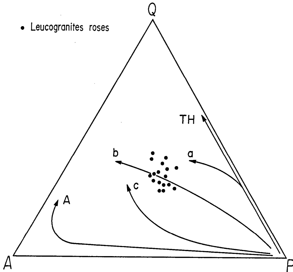
Fig. 5-5 : Diagramme modal Q-A-P dans lequel est reportée l'évolution de séries magmatiques typiques (Laméyre et Bowden, 1982) : Séries tholéitiques (TH), séries alcalines (A), séries calco-alcalines; pauvres en K_2O (a), intermédiaires (b), riches en K_2O (c).
