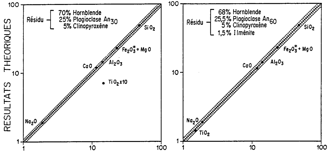
Fig.10-36 : Diagramme log (résultat théorique) = f (log (donnée analytique) ) permettant de comparer les résultats du modèle de fusion d'une amphibolite sans grenat avec les données analytiques.
