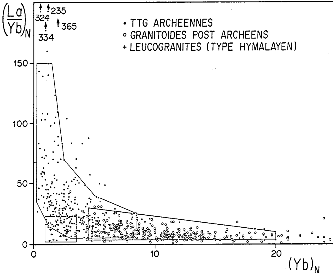
Fig. 15-7 : Diagramme (\frac{La}{Yb})_N = f (Yb)_N permettant de comparer l'allure des spectres de REE des granitoïdes archéens et modernes.
