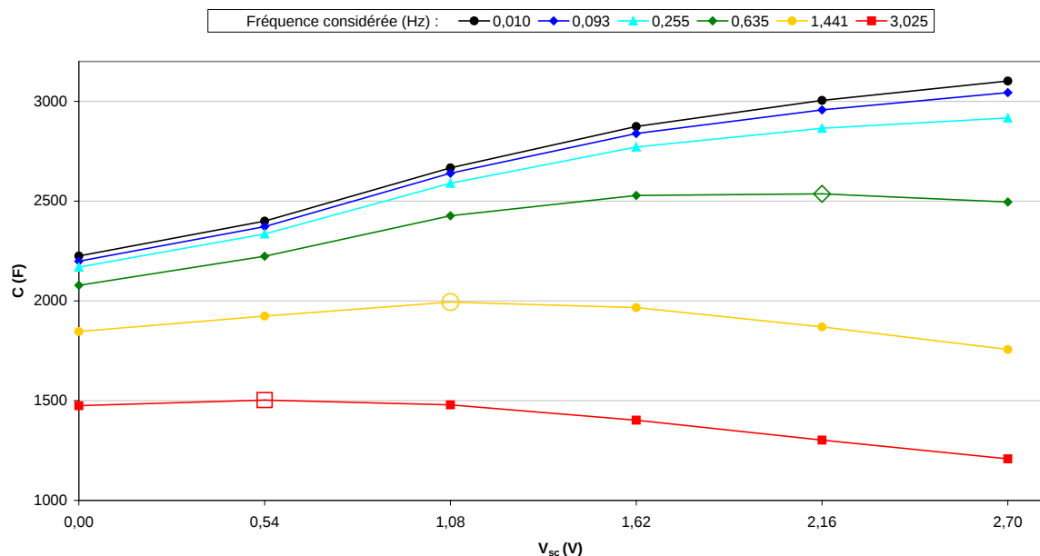
Figure 2. 22 : évolution de la capacité en fonction de la tension de polarisation pour différentes fréquences
