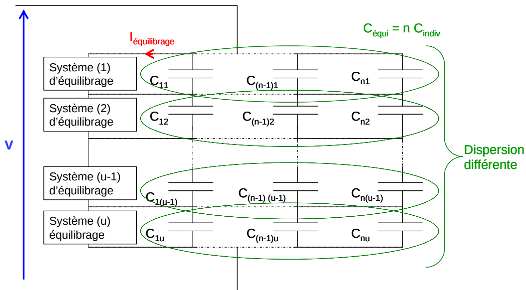
Figure 2. 29 : Représentation d'une mise en série/parallèle de (u*n) supercondensateurs avec les systèmes d'équilibrage correspondants.
