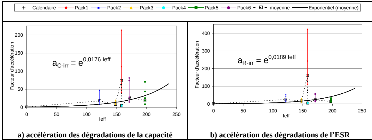
Figure 3. 48: Facteur d'accélération entre les dégradations irréversibles observées longtemps après cyclage et celles estimées par la loi calendaire en fonction du courant efficace
