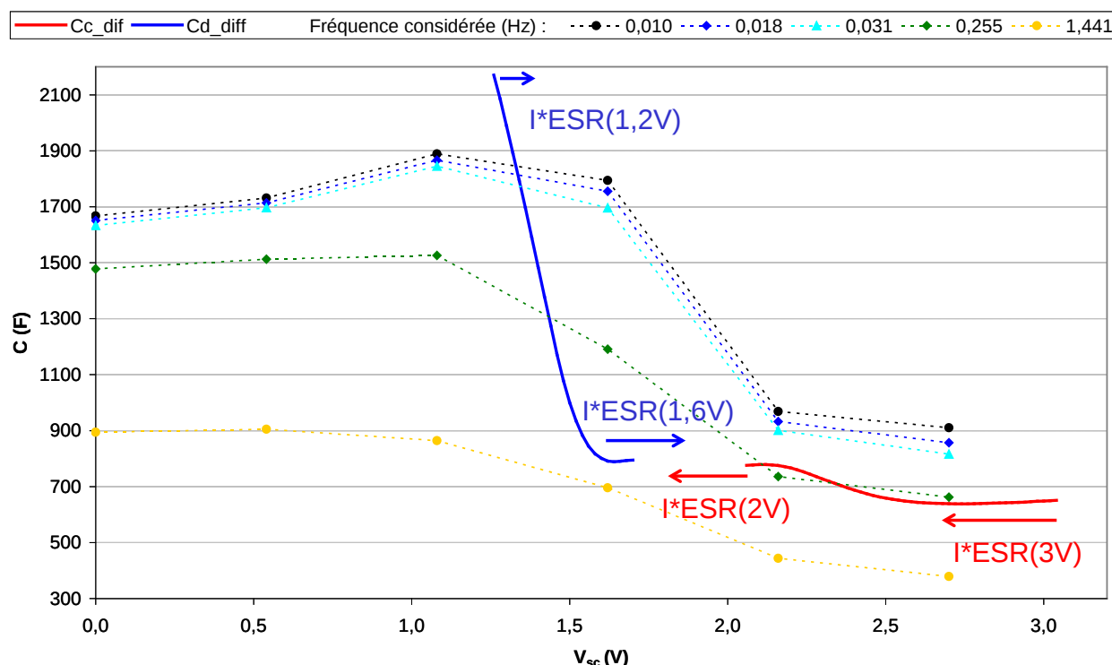
Figure 3. 35: C_{c\_diff}(V_{sc}) et C_{d\_diff}(V_{sc}) pour le dernier cycle (43000 ème ) et C(V_{sc}) capacité obtenue par spectroscopie complète 7h après l'arrêt du cyclage, et paramétré par la fréquence, le tout pour le composant P24
