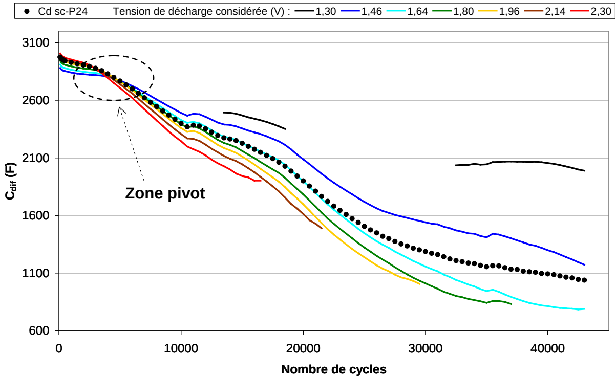
Figure 3. 31: C_{dif} décharge et C_d P24 ( I_{SC} de 300A) : Capacité différentielle obtenue pour certaines tensions de décharge et capacité constructeur en fonction du nombre de cycles
