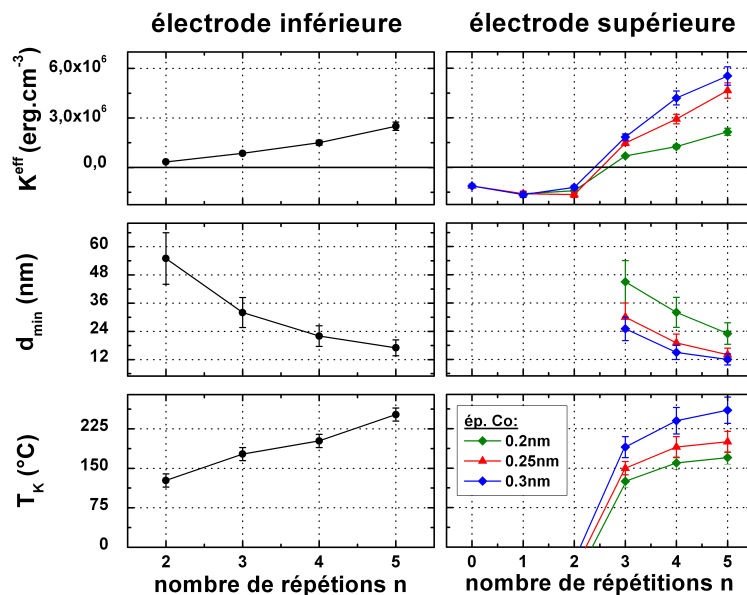
FIGURE 5.11 – Anisotropie effective (en haut), diamètre minimal de pilier pour respecter la condition KV/k_B T > 50 à température ambiante (au milieu) et température de basculement d'anisotropie (en bas) des électrodes inférieure (à gauche) et supérieure (à droite) en fonction du nombre n de répétitions de la multicouche (\text{Co}/\text{Pt})_n (électrode inférieure) ou (\text{Co}/\text{Pd})_n (électrode supérieure).
