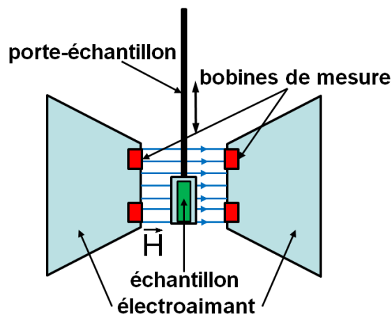
FIGURE 1.6 – Schéma de fonctionnement d'un VSM.
