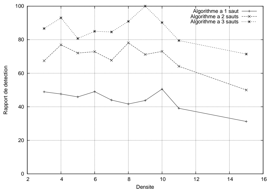
FIG. 4.16 – Rapport de détection des liens critiques.
