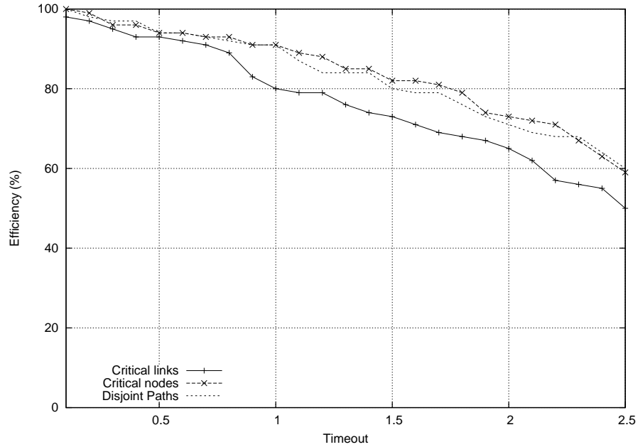
FIG. 4.19 – Efficacité des méthodes de prédiction en fonction de la valeur du timeout
