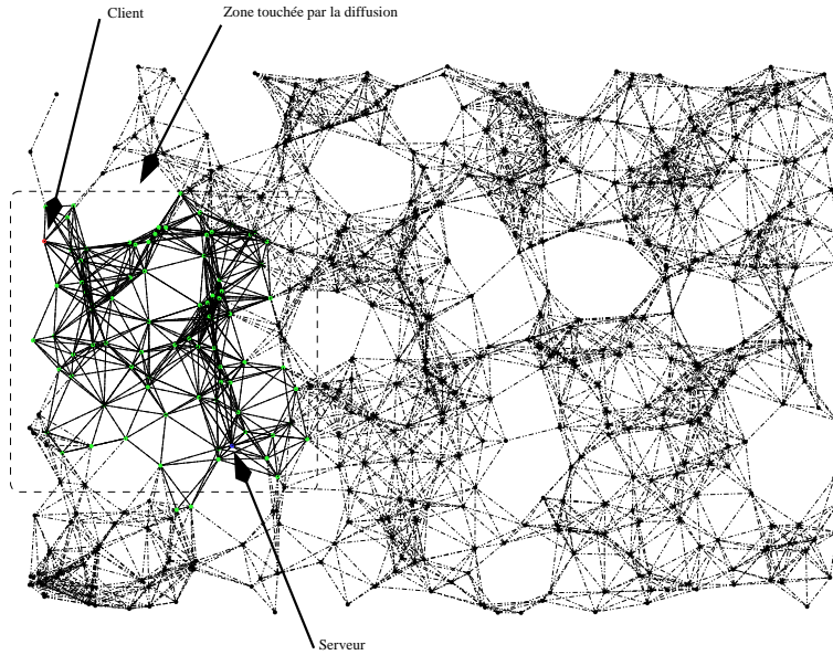
FIG. 4.7 – Diffusion confinée.
