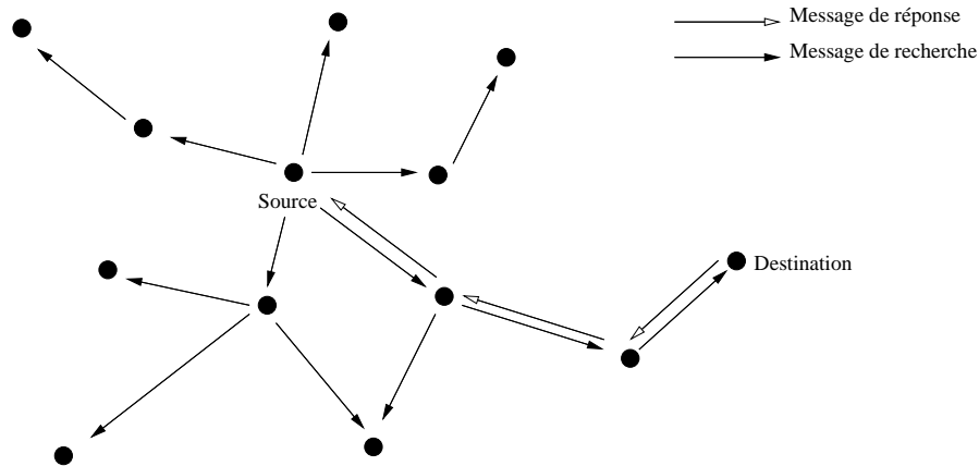
FIG. 2.8 – Recherche de route par un protocole réactif
