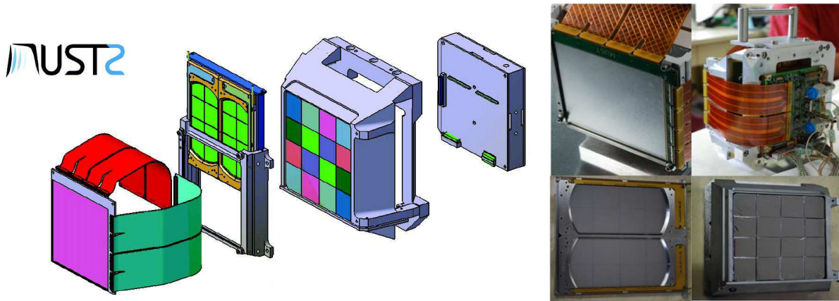
Fig. 6.7 – Vue éclatée d'un télescope MUST2 avec ses 3 étages de détection : (1) Silicium à pistes mince (128X, 128Y), (2) détecteur Si(Li) épais (16 secteurs), (3) 16 cristaux CsI; l'électronique, constituée de 2 cartes embarquées, est placée à l'arrière de part et d'autre du bloc de refroidissement dans lequel circule un mélange eau-alcool refroidi à 0°C.
