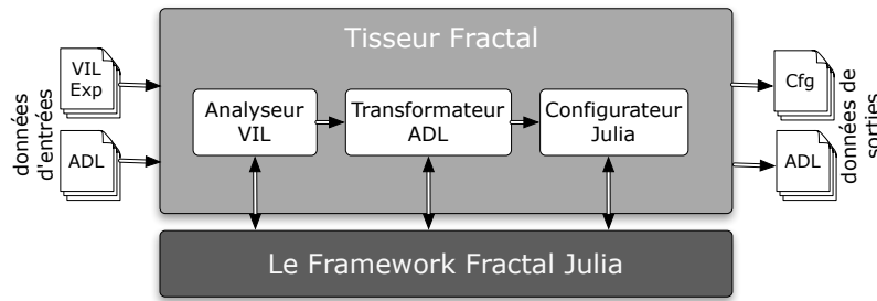
Figure A.1: L'architecture du Tisseur Fractal
