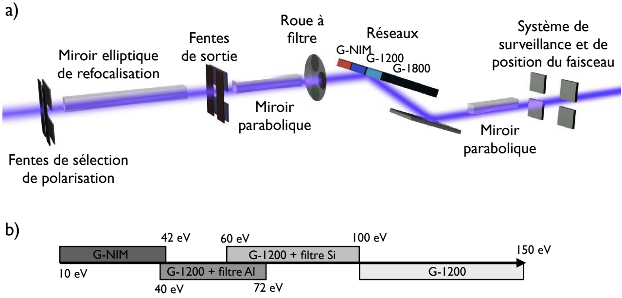
FIGURE 2.6 – Schéma de la ligne de métrologie BEAR du synchrotron italien Elettra. a) Détail des optiques constituant la ligne BEAR. b) Bandes spectrales accessibles grâce au monochromateur de la ligne composé de trois réseaux et d'une roue à filtre. Le réseau G-1800 fonctionne sur la plage 800 eV – 1400 eV.
