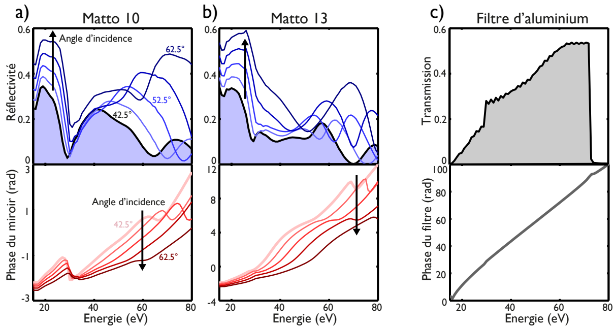
FIGURE 2.14 – Simulation de l'évolution de la réflectivité et de la phase de matto 10 et matto 13 en fonction de l'angle d'incidence. Réflectivité (courbes bleues) et phase (courbes rouges) de matto 10 (a) et matto 13 (b) entre 42.5° et 62.5° par pas de 5°. c) Transmission et phase du filtre de 250 nm d'aluminium calculées en utilisant les bases d'indices du CXRO pour les énergies supérieures à 30 eV. En dessous, Les indices du Palick sont utilisés, ce qui explique la discontinuité dans la transmission du filtre d'aluminium à 30 eV.
