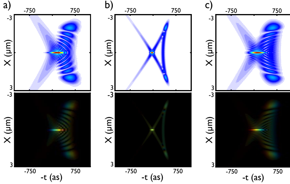
FIGURE 3.24 – Influence de l'atto-chirp sur la forme spatio-temporelle des impulsions On représente une impulsion attoseconde 75\mu m avant le foyer paraxial lorsqu'elle est focalisée par le miroir sphérique sur l'axe de la Fig. 3.11. L'impulsion initiale utilisée pour les calculs possède une GDD de +6000 as^2/rad (a), 0 as^2/rad (b), et -6000 as^2/rad (c). Le module du champ électrique (panneaux supérieurs) et la fréquence instantanée de l'impulsion (panneaux inférieurs) sont représentés dans les trois cas. L'échelle des fréquences instantanées reste inchangée par rapport aux figures précédentes.
