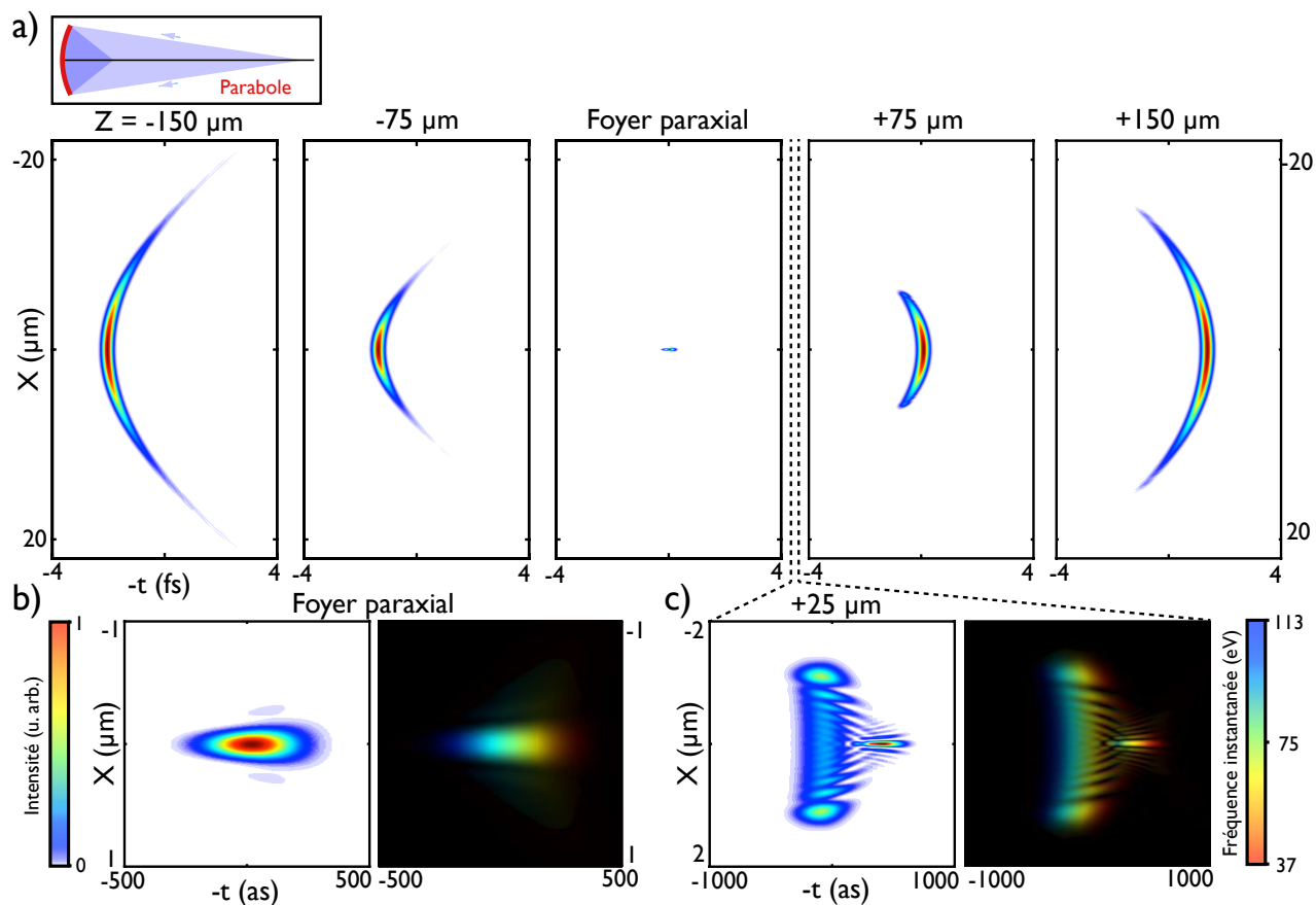
FIGURE 3.10 – Focalisation d'une impulsion attoseconde par un miroir parabolique pour une source sur l'axe. Le repère (x, y, z) choisi est le même que celui utilisé pour les Fig. 3.3 et Fig. 3.2. a) Evolution de l'intensité de l'impulsion autour du foyer paraxial. L'axe optique se trouve à la position x = 0 \mu\text{m} . b) Détail de l'évolution de l'intensité et de la fréquence instantanée de l'impulsion b) au foyer paraxial, et c) 25 \mu\text{m} après le foyer paraxial.
