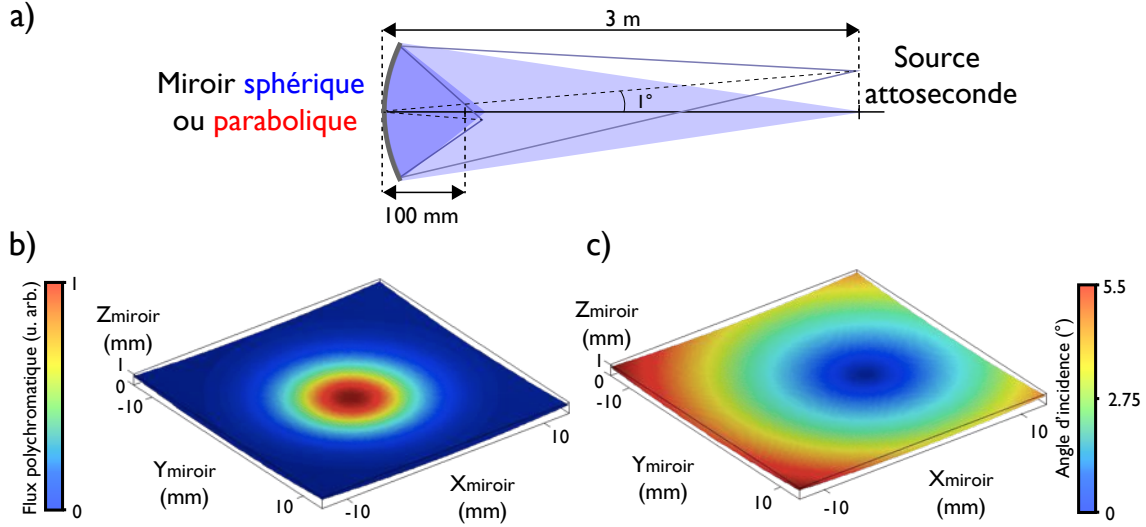
FIGURE 3.9 – Conditions des simulations pour les miroirs sphériques et paraboliques. a) Schéma des conjugaisons optiques étudiées, à savoir un miroir parabolique puis sphérique utilisé avec une source sur l'axe puis dans le champ. (b-c) Evolution du flux polychromatique (b) et de l'angle d'incidence des rayons (c) sur la surface du miroir lorsque la source est placée dans le champ sous un angle de 1^\circ .
