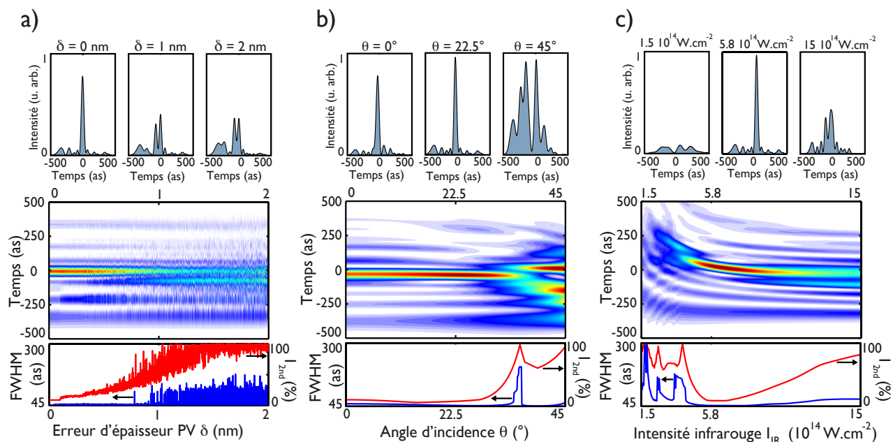
FIGURE 2.18 – Evolution de l'impulsion après réflexion sur matto 22 en fonction des conditions environnementales a) L'erreur Pic-à-Vallées sur l'épaisseur des couches déposées, b) l'angle d'incidence du faisceau XUV sur le miroir, et c) l'intensité de l'impulsion IR générant les impulsions attosecondes furent choisis comme les trois paramètres variables. Dans chaque cas, on trace l'évolution continue de l'impulsion en fonction du paramètre étudié (partie centrale), le profil d'impulsion étant détaillé pour trois valeurs du paramètre (panneaux supérieurs). L'évolution de la durée à mi-hauteur (FWHM) et de l'intensité du pic secondaire I_{2nd} (panneau inférieur) est également tracée.
