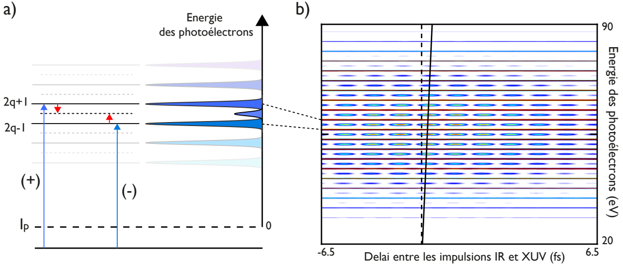
FIGURE 1.11 – Principe de la caractérisation d'un train d'impulsions attosecondes par la technique RABITT. a) Les transitions à deux-photons deux-couleurs permettent aux photoélectrons d'accéder à des niveaux d'énergies intermédiaires entre les harmoniques. b) L'étude de la synchronisation de ces pics satellites entre eux donnent directement le profil du retard de groupe des impulsions attosecondes.
