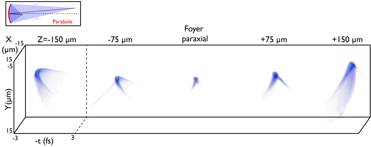
FIGURE 3.13 – Focalisation d’une impulsion attoseconde par un miroir parabolique utilisé dans le champ. Pour chaque position le long de l’axe de propagation, on représente l’intensité de l’impulsion en fonction des variables (x, y, t) . L’aberration de coma est responsable de l’apparition d’un double front d’impulsion, donnant une forme caractéristique en “V” inversé à l’impulsion attoseconde.
