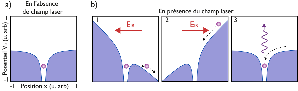
FIGURE 1.5 – Modèle semi-classique de la génération d'harmoniques d'ordre élevé. a) En l'absence de champ laser, l'électron est maintenu dans son niveau fondamental. b) Un champ laser intense abaisse la barrière de potentiel, que l'électron franchit par effet tunnel. Une fois dans le continuum, l'électron acquiert de l'énergie cinétique (1). Une demi-période infrarouge plus tard, la barrière de potentiel s'inverse (2). L'électron retourne alors dans son niveau fondamental et libère l'énergie acquise sous forme d'un photon XUV (3).
