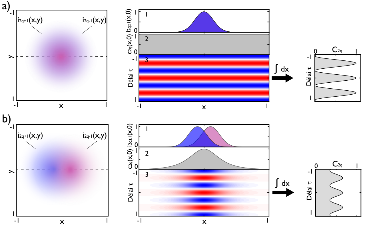
FIGURE 5.10 – Perte de contraste des pics satellites d'une trace RABITT due à un couplage en amplitude. Construction du profil du pic satellite mesuré (panneaux de droite) en l'absence (a) et en présence (b) de couplage en amplitude. Dans les deux cas, on trace les profils spatiaux i_{2q±1}(x, y) des deux harmoniques consécutives (panneaux de gauche). On représente également (1) une coupe de ces profils i_{2q±1}(x, 0) , (2) le contraste cohérent c_{2q}(x, 0) en chaque point, et (3) l'impact sur l'oscillation du pic satellite produit en chaque point. Tous les axes sont en unités arbitraires.
