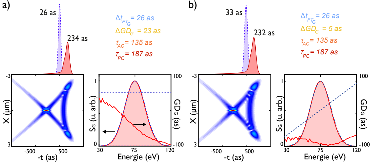
FIGURE 4.8 – Exemple de minimisation de la durée globale d’une impulsion aberrante. Impulsion avant (a) et après (b) minimisation de la durée globale. Dans les deux cas, une coupe radiale du module du champ électrique de l’impulsion spatio-temporelle (panneaux inférieurs gauches), ainsi que l’impulsion initiale (courbe pointillée bleue) et l’impulsion globale (courbe continue rouge) sont tracées (panneaux supérieurs gauches). Sur les panneaux inférieurs droits, le spectre initial et le retard de groupe initial (courbes pointillées bleues) sont tracés avec le spectre global et le retard de groupe global de l’impulsion finale (courbes rouges). Enfin, la décomposition de la durée globale dans les deux cas est également détaillée sur les panneaux supérieurs droits.
