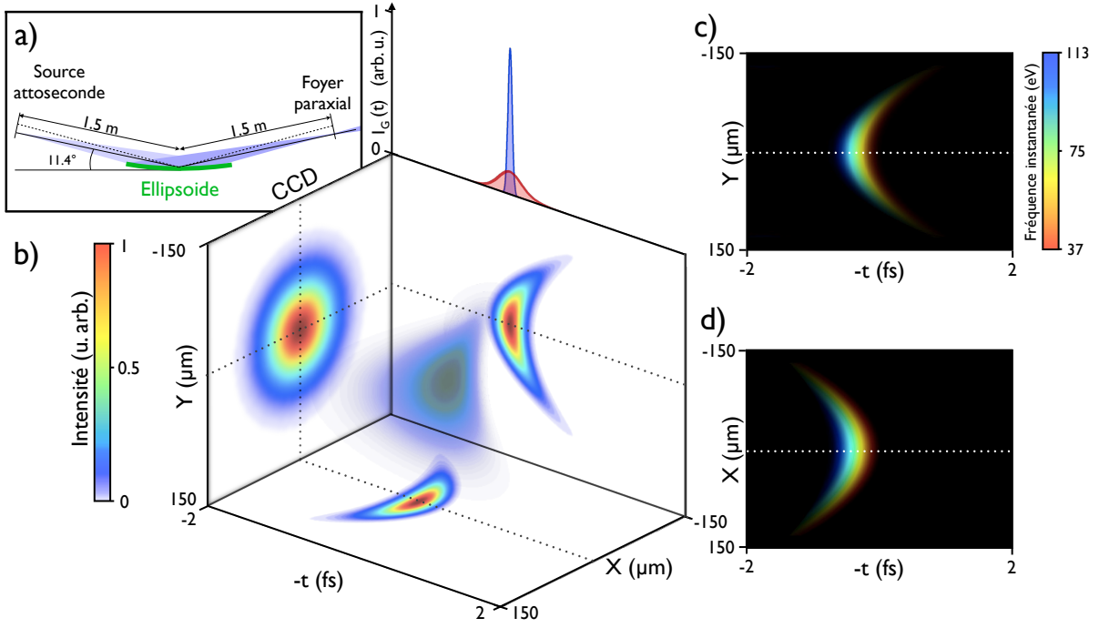
FIGURE 4.5 – Simulation du champ électrique spatio-temporel d’une impulsion attoseconde en présence d’aberrations. a) L’impulsion attoseconde est focalisée par un miroir ellipsoïdal en incidence rasante, dont l’angle de rasance optimal vaut 11.5^\circ . Le miroir est réglé pour un angle de rasance de 11.4^\circ pour ajouter de l’astigmatisme sur l’impulsion. b) Intensité spatio-temporelle de l’impulsion au foyer paraxial. L’impulsion globale I_G(t) colorée en rouge et la limite de Fourier globale I_{TFG}(t) en bleu sont représentées au-dessus de la boîte. c) (resp. d)) Evolution de la fréquence instantanée de l’impulsion au niveau de la coupe correspondante en b) projetée dans le plan (y, t) (resp. (x, t) ). L’astigmatisme provoque l’inversion de la courbure des fronts de l’impulsion entre les deux coupes. L’atto-chirp quant à lui fait varier linéairement la fréquence instantanée de l’impulsion dans son enveloppe.
