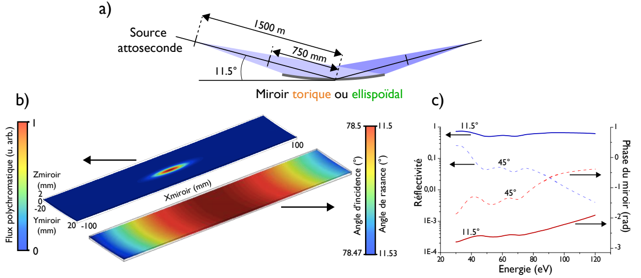
FIGURE 3.17 – Conditions des simulations pour les miroirs torique et ellipsoïdal. a) Conjugaison 2f - 2f étudiée. b) Evolution du flux polychromatique et de l'incidence des rayons à la surface du miroir torique en conjugaison 2f - 2f . c) Evolution de la réflectivité et de la phase spectrale d'un miroir en platine pour des angles de rasance de 11.5^\circ et de 45^\circ
