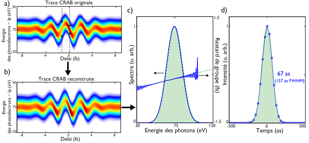
FIGURE 5.4 – Reconstruction d'une impulsion en l'absence de couplage par la technique CRAB.
