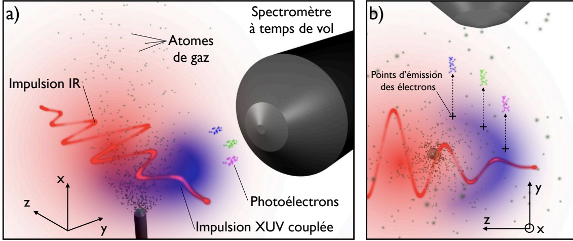
FIGURE 5.1 – Caractérisation d'une impulsion attoseconde en présence de couplages spatio-temporels. a) Vue générale de l'interaction entre les champs IR et XUV et les atomes de gaz. b) Vue de dessus. En présence de couplages sur l'impulsion XUV, chaque point de l'impulsion génèrera un paquet d'électrons copiant les propriétés de l'impulsion XUV en ce point. Les photoélectrons bleus sont émis en avance par rapport aux photoélectrons verts et roses, traduisant le fait que l'instant d'arrivée de l'impulsion XUV n'est pas le même en chaque point.
