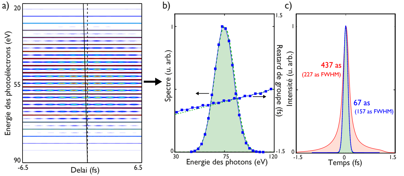
FIGURE 5.6 – Reconstruction d'une impulsion en présence de couplages par la technique RABITT. a) Trace RABITT obtenue en intégrant les spectres de photoélectrons générés par chaque point du train d'impulsions. On observe un brouillage des oscillations des pics satellites dû à la structure spatio-temporelle du train d'impulsions. Malgré tout, la désynchronisation linéaire des sidebands due à l'atto-chirp reste visible. b) Enveloppe du spectre harmonique et retard de groupe mesurés directement sur la trace RABITT en a) (carrés bleus), et comparés aux spectre et retard de groupe initiaux (courbes vertes pointillées). c) Comparaison du profil d'une impulsion attoseconde du train reconstruit à partir des mesures faites sur la trace RABITT (courbe bleue), et de celui d'une impulsion du train émis par la source (courbe pointillée verte), avec l'impulsion globale (courbe continue rouge) associée à l'impulsion spatio-temporelle de la Fig. 5.5 b). Les durées RMS et à mi-hauteur sont indiquées.
