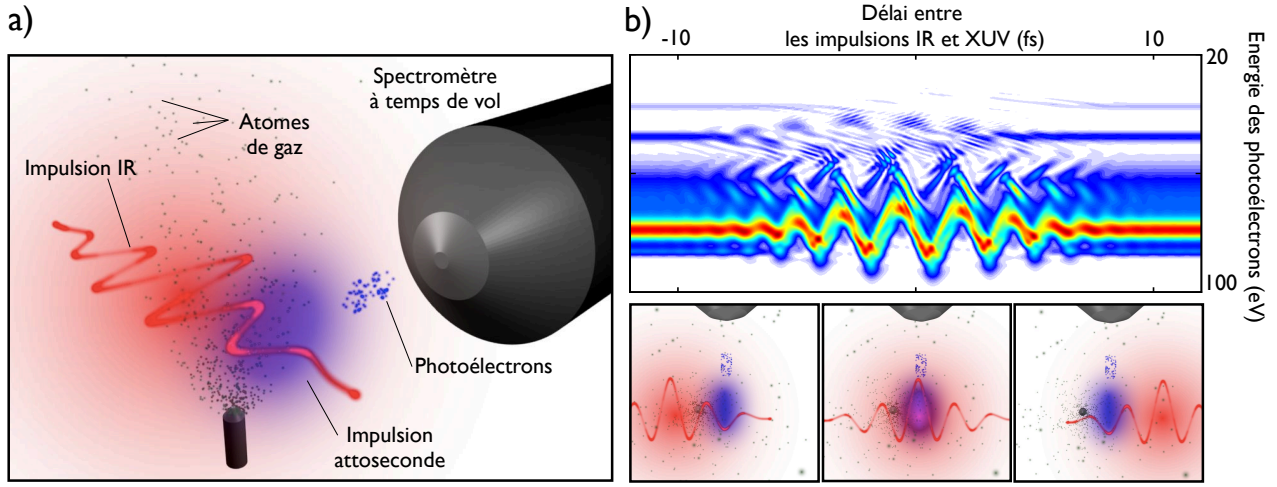
FIGURE 1.9 – Principe général de la caractérisation d'une impulsion attoseconde. a) On procède par la mesure de spectres de photoélectrons en fonction du retard \tau avec le champ d'habillage IR. b) Pour des retard \tau grands devant la durée de l'impulsion IR, les spectres de photoélectrons représentent directement le spectre de l'impulsion attoseconde. Pour les délais intermédiaires, les deux impulsions se recouvrent et les spectres varient significativement, ces variations étant représentatives de la phase spectrale de l'impulsion attoseconde.
