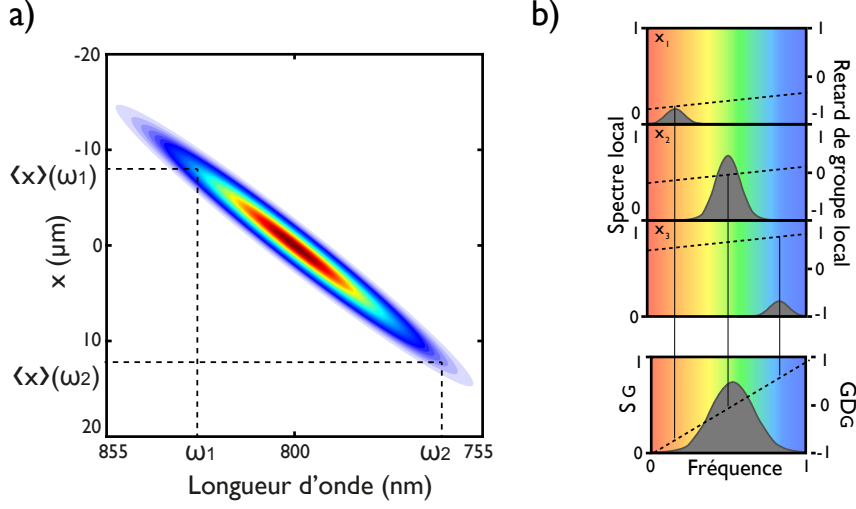
FIGURE 4.4 – Calcul des grandeurs globales. a) Evolution de l'intensité spatio-spectrale, c'est à dire du spectre local, de l'impulsion de la Fig. 4.3 a) en sortie du système optique. Le chirp spatial est responsable d'un décalage linéaire du spectre local. b) Déduction du spectre global S_G et du retard de groupe global GD_G à partir des grandeurs locales représentées en trois points. Les axes sont en unités arbitraires. Le décalage entre les trois spectres locaux provient du chirp spatial, la pente commune aux trois retards de groupes locaux est due à la GDD, et le décalage vertical entre ces retards de groupe est engendré par le retard linéaire de pente \gamma . Pour déterminer la quantité GD_G , on calcule la moyenne du retard de groupe local pondérée par le spectre local. Mais du fait du chirp spatial et du retard linéaire \gamma , la pente du retard de groupe global est bien supérieure à la GDD induite par le système optique.
