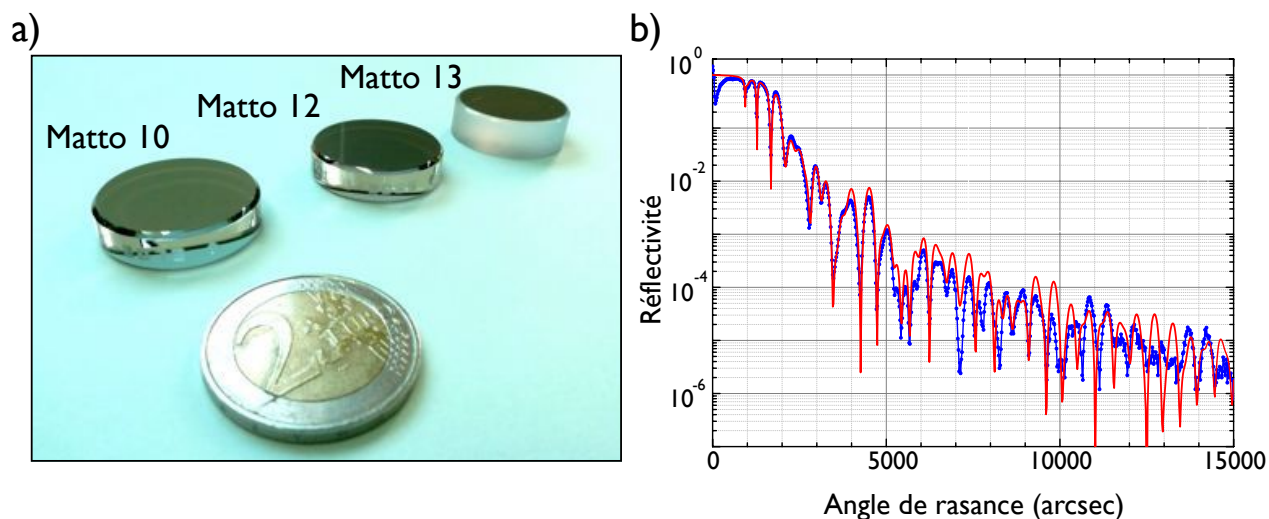
FIGURE 2.9 – Résultat de la fabrication des miroirs. a) Photo des trois miroirs. b) Mesure de la réflectivité (courbe bleue) de matto 12 à 0.154\text{ nm} obtenue par réflectométrie en X-rasants. La courbe rouge est le résultat de la simulation.
