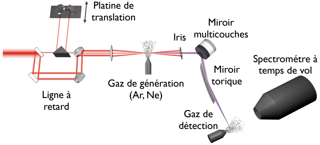
FIGURE 2.7 – Schéma de la source d'impulsions attosecondes basé sur le laser LUCA du CEA-Saclay. A partir de la lentille de focalisation du faisceau IR, la ligne est placée sous vide.
