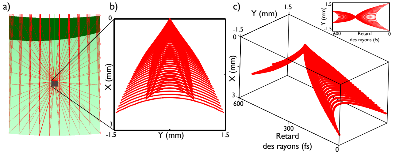
FIGURE 3.3 – Principe des spot diagrams 2D et 3D. a) Vue de dessus de la tache focale obtenue sur la Fig 3.2 avec la réflexion des rayons sur le miroir en arrière plan. Un plan noir a été placé au niveau du foyer paraxial. b) Le spot diagram 2D est obtenu en traçant l'intersection d'une matrice de 100 \times 100 rayons réfléchis par le miroir avec le plan noir précédent. Le point de coordonnées (0; 0) correspond au point d'impact sur le plan du spot diagram 2D du rayon réfléchi par le sommet du miroir. La forme en aigrette de la tache focale obtenue est caractéristique de la présence de coma. c) Le spot diagram 3D est obtenu en rajoutant l'information sur le retard du chemin optique dans la profondeur du spot diagram 2D. L'origine de l'axe des retards est prise au niveau du rayon arrivant le premier sur le plan noir paraxial. Insert : Vue de dessus du spot diagram 3D.
