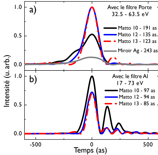
FIGURE 2.13 – Reconstruction temporelle des impulsions attosecondes obtenues après réflexion sur les miroirs attosecondes et le miroir en argent. On applique numériquement a) un filtre porte ne conservant que la plage 32.5 – 63.5 eV, et b) un filtre de 250 nm d'aluminium. La durée à mi-hauteur (FWHM) est indiquée pour chaque impulsion.
