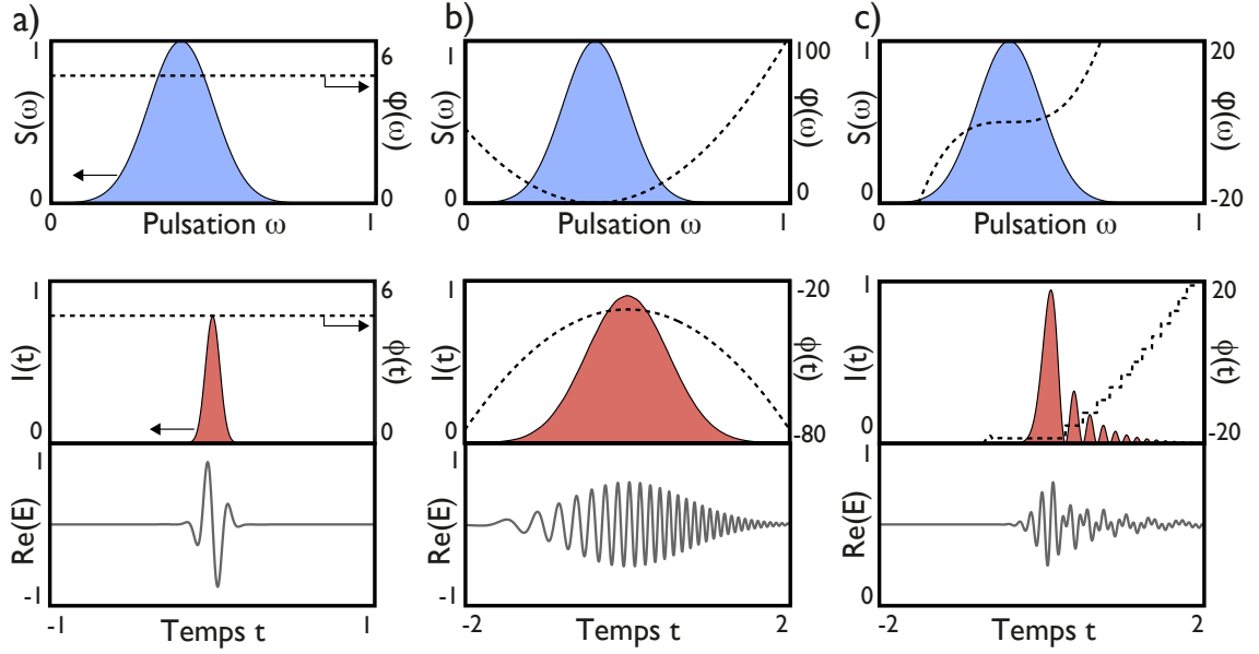
FIGURE 1.4 – Influence de la phase spectrale sur l'impulsion. Pour un spectre donné S(\omega) , on représente l'effet de la phase spectrale \varphi(\omega) sur le profil temporel I(t) et la phase temporelle \phi(t) de l'impulsion, ainsi que sur le champ électrique réel. Cas d'un déphasage constant (a), d'une phase spectrale parabolique (b) et du troisième ordre (c). Les valeurs des phases sont en radians, les autres grandeurs sont en unités arbitraires.
