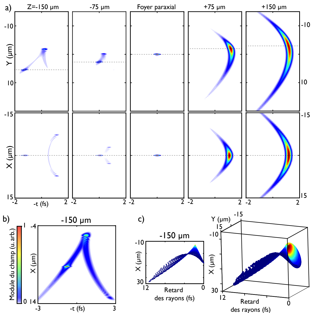
FIGURE 3.16 – Focalisation d'une impulsion attoseconde par un miroir sphérique utilisé dans le champ. a) Coupes représentant l'évolution de l'intensité de l'impulsion autour du foyer paraxial. Les lignes pointillées indiquent la position du plan orthogonal associé. b) Evolution du module du champ électrique dans le plan (y, t) 150 \mu\text{m} avant le foyer paraxial. c) Spot diagram 3D de l'impulsion 150 \mu\text{m} avant le foyer paraxial. L'échelle de couleur représente le flux polychromatique porté par chaque rayon. Seuls les rayons transportant un flux supérieur à 1 % du flux maximum sont pris en compte.
