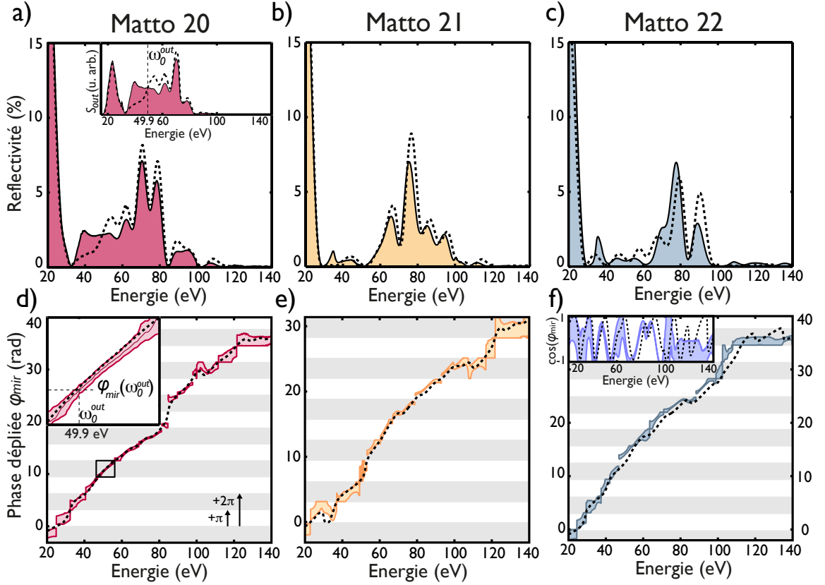
FIGURE 2.20 – Mesure de la réflectivité (a-c) et de la phase (d-f) des trois miroirs. Les réflectivités et les phases simulées (lignes pointillées) sont superposées aux mesures (courbes colorées). En a), l'insert représente le spectre S_{out}(\omega) réfléchi par matto 20 et déduit de S_{in} et des réflectivités mesurée (courbe colorée) et simulée (courbe pointillée). On peut ainsi déduire expérimentalement la fréquence porteuse moyenne \omega_0^{out, xp} de l'impulsion réfléchie. L'insert en d) correspond à un agrandissement de la phase sur la plage spectrale 47 – 56 eV sur laquelle la phase \phi_{mir}(\omega_0^{out, xp}) peut être précisément mesurée. La ligne continue au centre de la zone colorée correspond à la phase reconstruite en considérant que \cos(\phi_{ref}) vaut 0. En f), l'insert représente le \cos(\phi_{mir}) simulé (ligne pointillée) et celui reconstruit à partir de l'échantillon de référence de 20 nm (courbe colorée en bleu). Les réflectivités simulées tiennent compte de la polarisation (80; 20) de la ligne synchrotron.
