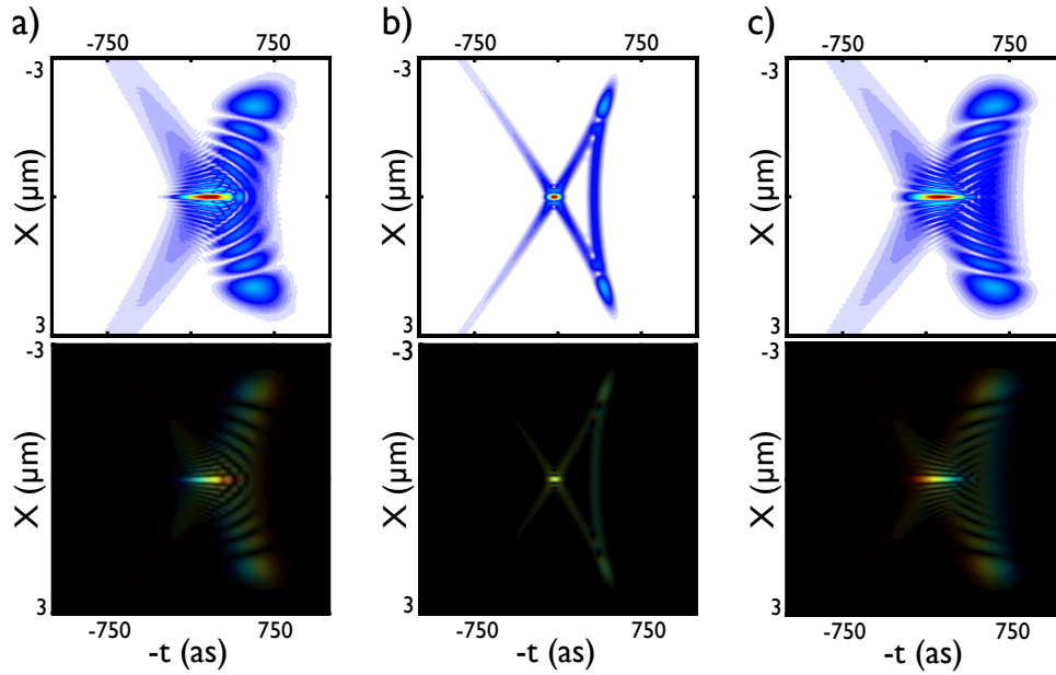
FIGURE 3.24 – Influence de l’atto-chirp sur la forme spatio-temporelle des impulsions On représente une impulsion attoseconde 75 \mu\text{m} avant le foyer paraxial lorsqu’elle est focalisée par le miroir sphérique sur l’axe de la Fig. 3.11. L’impulsion initiale utilisée pour les calculs possède une GDD de +6000 \text{ as}^2/\text{rad} (a), 0 \text{ as}^2/\text{rad} (b), et -6000 \text{ as}^2/\text{rad} (c). Le module du champ électrique (panneaux supérieurs) et la fréquence instantanée de l’impulsion (panneaux inférieurs) sont représentés dans les trois cas. L’échelle des fréquences instantanées reste inchangée par rapport aux figures précédentes.
