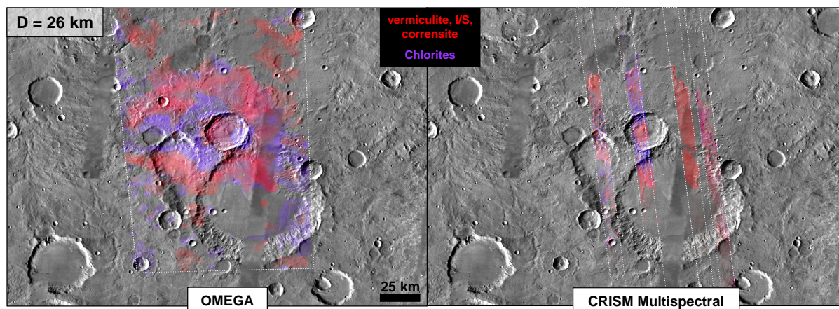
FIGURE 4.9 – Cratères et diversité minérale (3). Cratère de 26 km de diamètre dans Tyrrhena Terra entièrement couvert par OMEGA. La totalité de l'éjecta lobé est hydraté. Les smectites/vermiculites Fe/Mg se concentrent à l'intérieur du cratère et dans la partie distale des éjectas, la chlorite se concentre dans la partie proximale. Les résultats sont similaires avec OMEGA ou CRISM (MSP).
