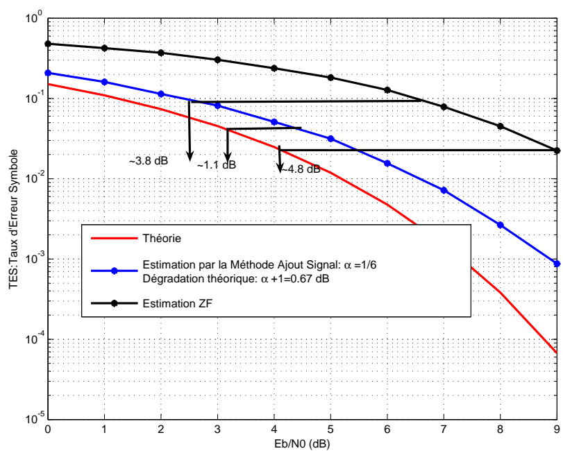
FIGURE 4.10 – Taux d’Erreur Symbole : Canal Pedestrian A , Egaliseur type ZF
