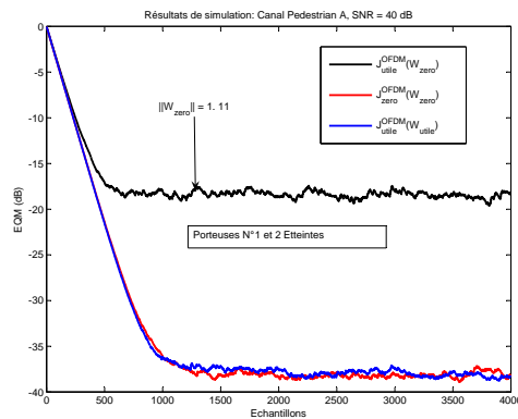
(d) Porteuse N°1 et 2 éteintes, \|W_{zero}\| = 1.11
