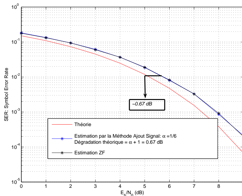
FIGURE 4.8 – Taux d'Erreur Symbole : Canal Gaussien
