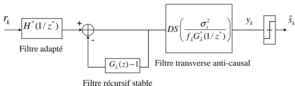
FIGURE 2.15 – Structure de l'Égaliseur Linéaire Récuratif ELR
