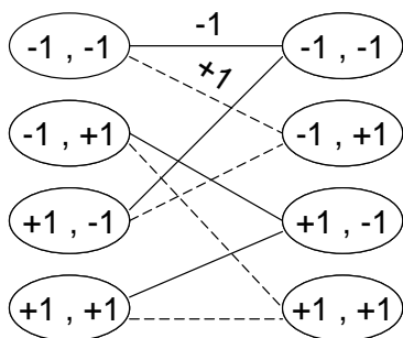
FIGURE 2.20 – Structure d'une section du Treillis pour une constellation BPSK
