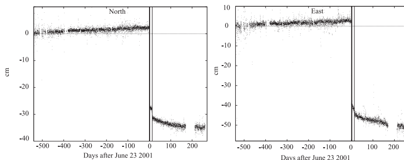
FIGURE 1.4: Série temporelle GPS (2 ans) de la station d'Arequipa (Pérou) montrant clairement les déplacements cosismiques liée au séisme de 2001, M_w 8.4 (ligne noire verticale) et d'une réplique majeure ( M_w 7.5, ligne verticale grise), ainsi que les déplacements liées à la déformation postsismique. D'après Melbourne et al. [2002]
