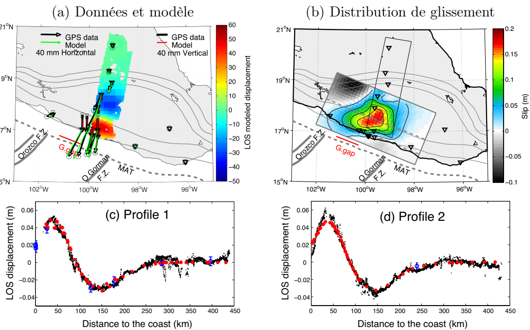
B. Inversion avec les données InSAR seules ( w_{GPS} = 1 et w_{SAR} = 100 )
