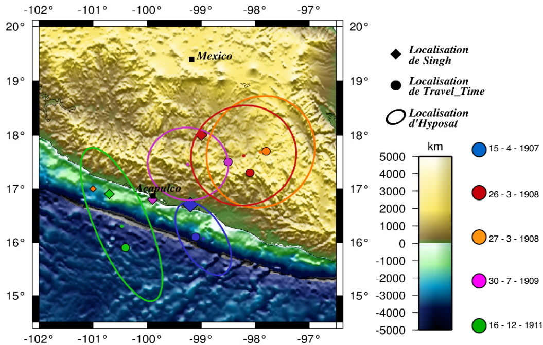
FIGURE 1.16: Localisation probable des séismes s'étant produits dans la lacune da Guerrero de 1907 à 1911. Les épïcêtres estimés par différentes techniques sont présentés. Les couleurs représentent différents séismes. (Luis Rivera, communication personnelle)
