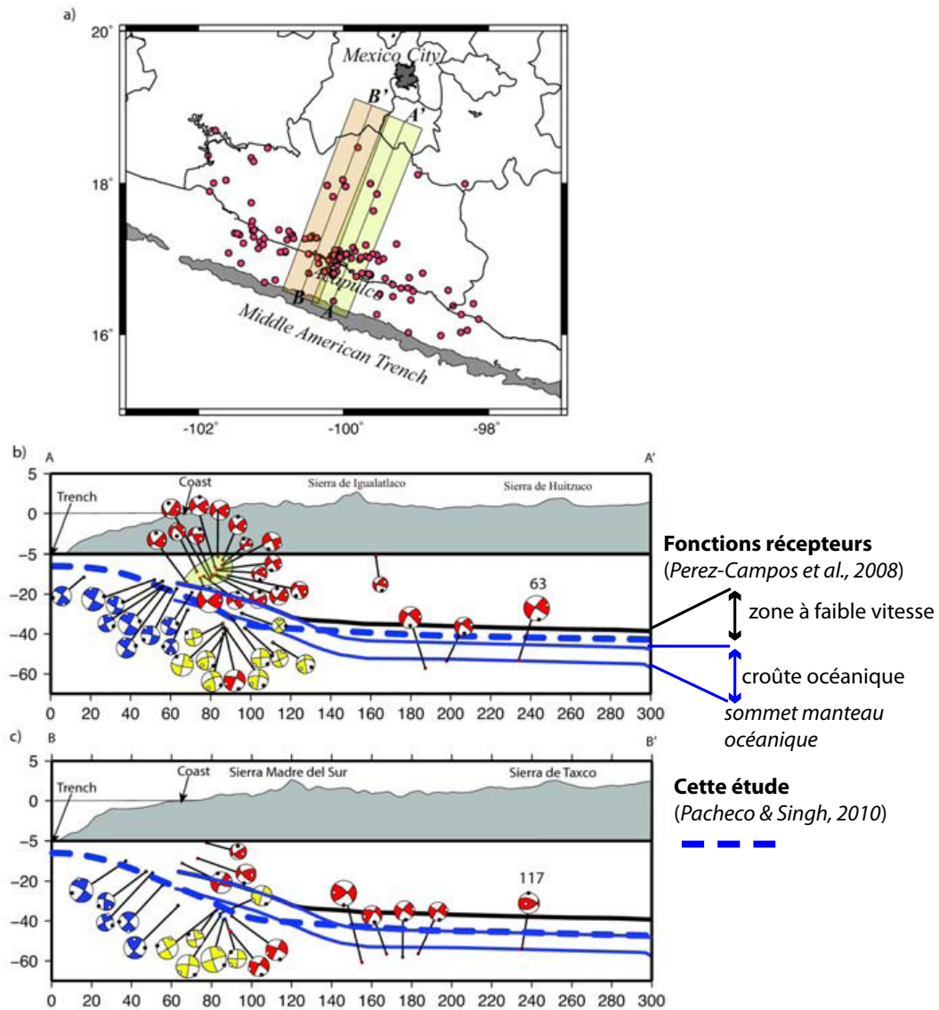
FIGURE 1.13: Localisation de la sismicité et géométrie de la subduction, d'après Pacheco and Singh [2010] . (a) Carte de la région montrant les epicentres des 132 séismes régionaux analysés ( M_w 3.3 à 6.7, entre 1995 et 2008). Les séismes situés dans les zones rectangulaires colorées sont projetés sur les coupes AA' et BB'. (b) Coupe au niveau de la ligne AA', avec projection des hypocentres. (c) Coupe au niveau de la ligne BB'. Les mécanismes au foyer en bleu, jaune, rouge, correspondent respectivement aux séismes superficiels de compression, aux séismes profonds de compressions, et aux séismes d'extension. L'interface de subduction proposée dans cette étude est présentée en pointillés bleus, elle est comparé à celle proposée par Pérez-Campos et al. [2008] à partir des fonctions récepteurs.
