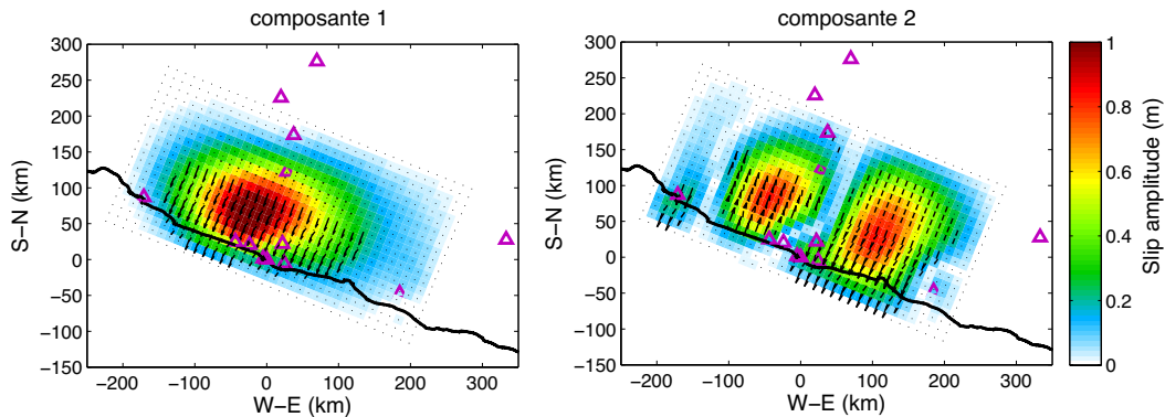
(b) Distributions de glissement associées aux deux premières composantes ( L_1 et L_2 )
