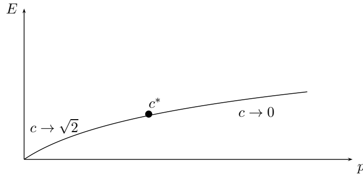
Figure 1.2 – Courbe de l'énergie E en fonction du moment p dans le cas N = 2 .
