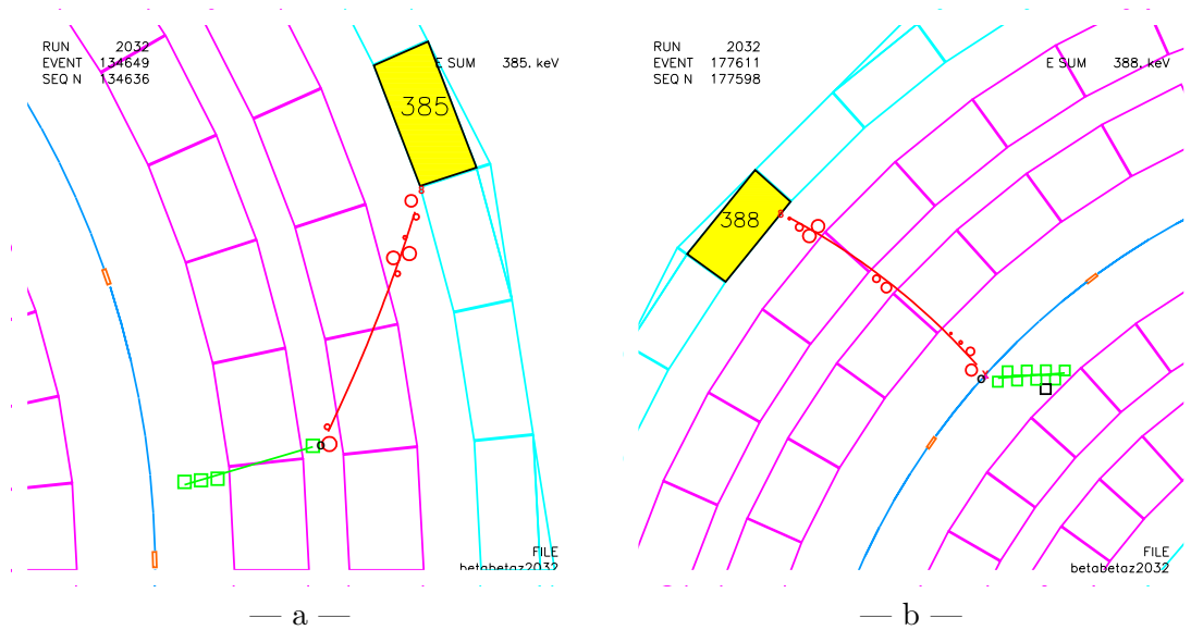
FIGURE 2.9 – Décroissance BiPo observée par NEMO 3 sur un fil d'une cellule Geiger (a) et sur/dans une des feuilles source de ^{100}\text{Mo} (b). La trace de l'électron est indiquée par les cercles rouges et celle de la particule \alpha retardée avec les carrés verts.
