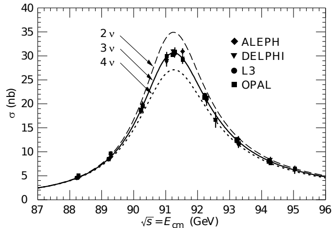
FIGURE 1.1 – Largeur invisible du Z^0 mesurée et comparée aux prédictions théoriques pour 2, 3 et 4 familles de neutrinos légers.
