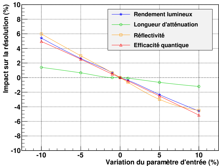
FIGURE 3.30 – Propagation de l'incertitude des paramètres d'entrée sur la résolution en énergie donnée par la simulation. La réciprocité des erreurs est estimée pour une configuration de compteur à scintillation SuperNEMO.
