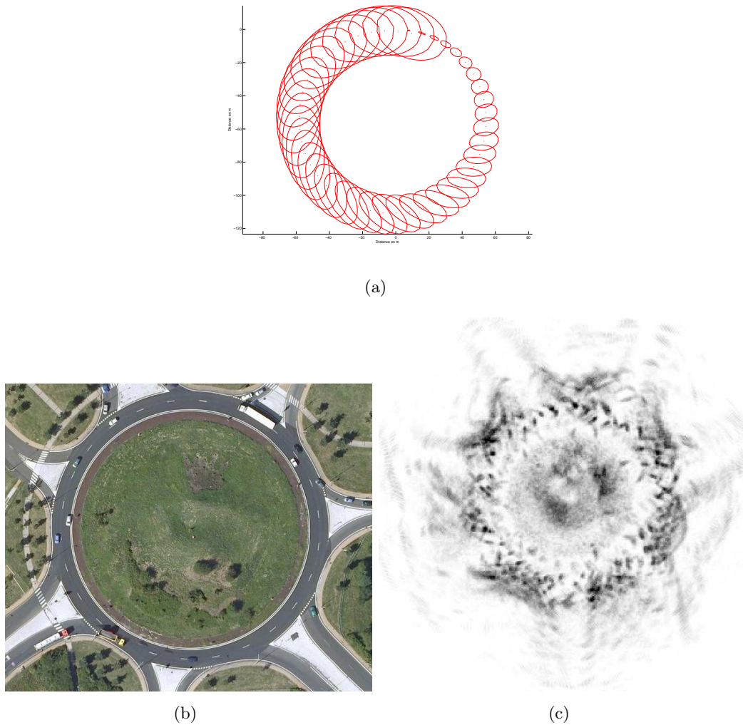
FIGURE 3.14 – Odométrie radar en environnement dynamique : (a) poses successives estimées par la navigation à l'estime utilisant l'analyse de la distorsion avec leurs incertitudes à 3\sigma . (b) vue aérienne de la zone d'expérimentation. (c) reconstruction de la cartographie.
