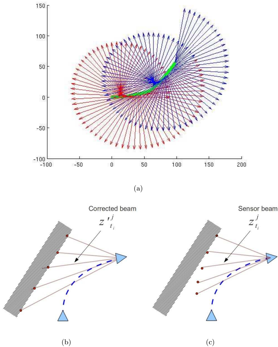
FIGURE 3.1 – (a) Phénomène de distorsion : lorsque le véhicule se déplace selon la trajectoire verte, le capteur est en train d’effectuer une acquisition. Chaque faisceau du capteur est représenté en rouge et en bleu pour, respectivement, la première et la seconde acquisition. Le premier et le dernier faisceau de chaque acquisition ne mesurent pas la même chose. Chaque scan est distordu par le mouvement. (b) représente l’acquisition souhaitée depuis la seconde position (ou dans le cas d’une approche « stop & scan » avec les faisceaux corrigés z_{t_i}^j du scan j pris au temps t_i . (c) montre l’acquisition obtenue sans prendre en compte le mouvement c’est-à-dire en considérant les faisceaux non corrigés z_{t_i}^j .
