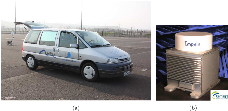
FIGURE 4.25 – (a) Véhicule expérimental du LASMEA : Véloc, (b) Vue générale du capteur radar IMPALA.
