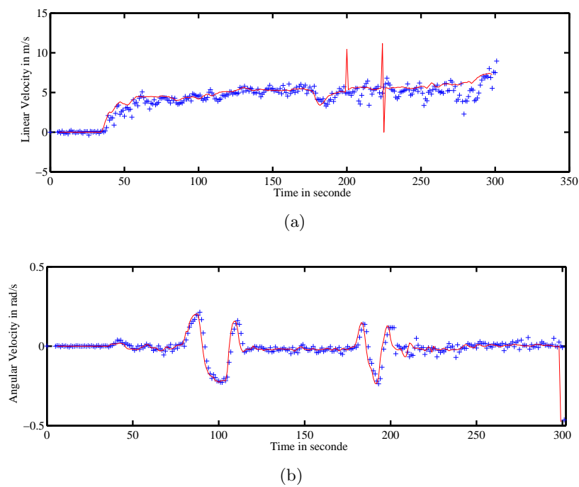
FIGURE 4.14 – Estimation de vitesses basée sur Odométrie IMPALA : (a) vitesse linéaire, (b) vitesse angulaire. En rouge la vérité terrain, en bleu l'estimation donnée par la méthode.
