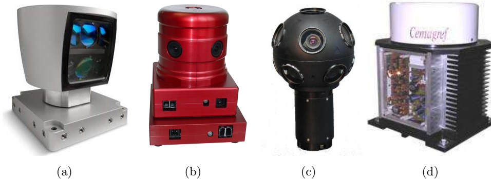
FIGURE 1.3 – Exemples de capteurs panoramiques : (a) HDL-64E (Velodyne), (b) cameras Lady Bug (Point Grey), (c) Dodeca camera (Immersive Media), (d) radar FMCW K2Pi (Cemagref).
