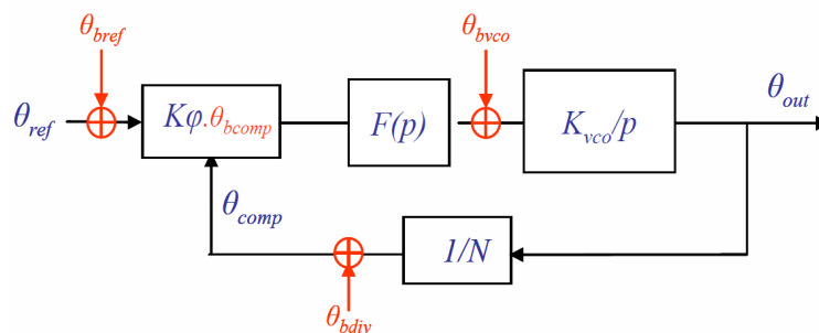
Fig. 23. Illustration d'une PLL
