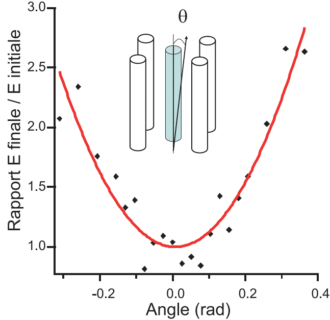
FIGURE 3.10 – Energie relachée dans le nuage par 40 ms de relaxation dipolaire rapportée à l'énergie du système sans relaxation dipolaire, en fonction de l'angle \theta entre l'axe des tubes et le champ magnétique \vec{B} .
