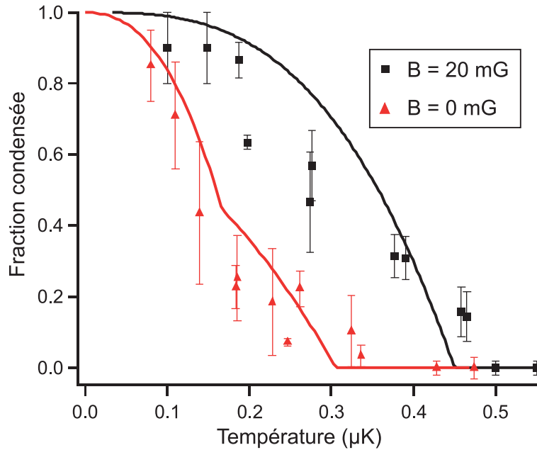
FIGURE 4.15 – Fraction condensée du nuage, en fonction de la température. Les données représentées par des carrés noirs sont mesurées après 200 ms passées à un champ magnétique (20 mG) supérieur au champ critique B_c , suffisant ne pas observer de dépolarisation, même provenant du gaz thermique. Les triangles rouges représentent des données similaires, mais prises à un champ (quasi-nul) inférieur à B_c . Les courbes en traits pleins correspondent à des ajustements par des fonctions donnant la (les) température(s) critique(s) dans le cas d'un nuage dans un piège harmonique du type : \frac{N_{\text{BEC}}}{N_{\text{Tot}}} = A(1 - (\frac{T}{T_c})^3) . Les barres d'erreurs proviennent de la moyenne sur 5 points.
