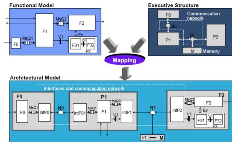
Figure 26. Illustration des modèles MCSE [73].
