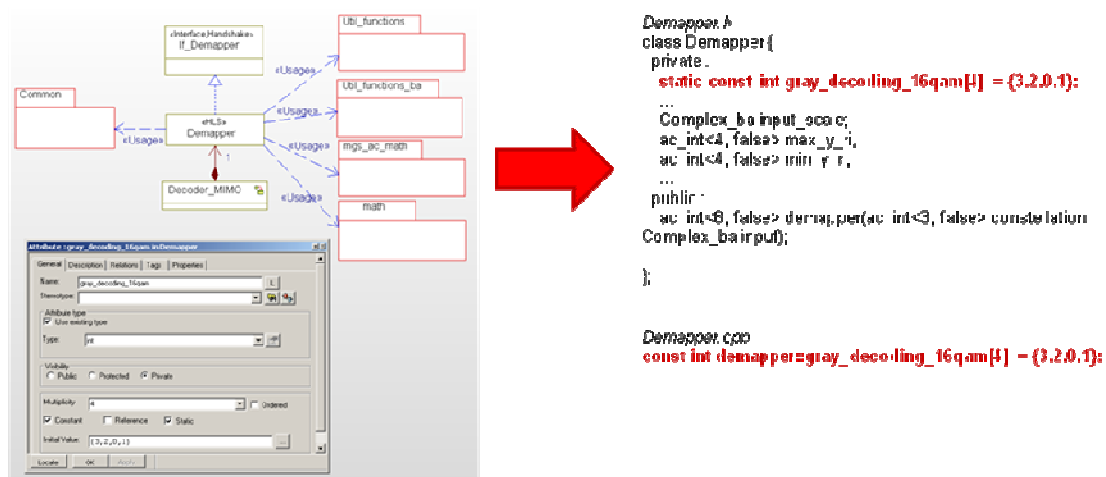
Figure 68. Exemple de génération de code de la classe « Demapper », stéréotypée « HLS », ayant entre autre un attribut de type tableau dont les valeurs initiales sont des constantes statiques.
