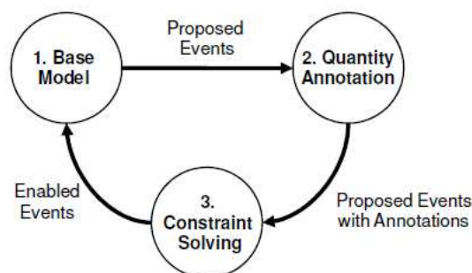
Figure 25. Illustration des 3 phases d'exécution dans Metro II, extrait de [71].
