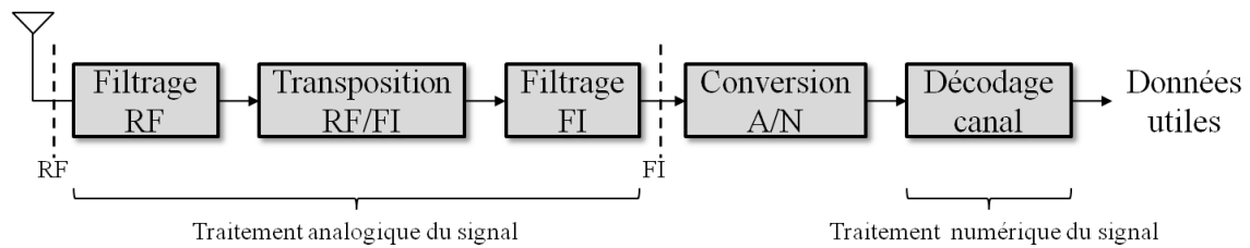
Figure 13. Architecture fonctionnelle typique d'un système de radio logicielle restreinte (RLR).
