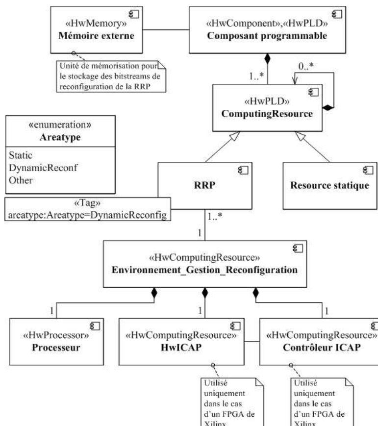
Figure 87. Méta-modèle d'une architecture matérielle reconfigurable d'un FPGA.
