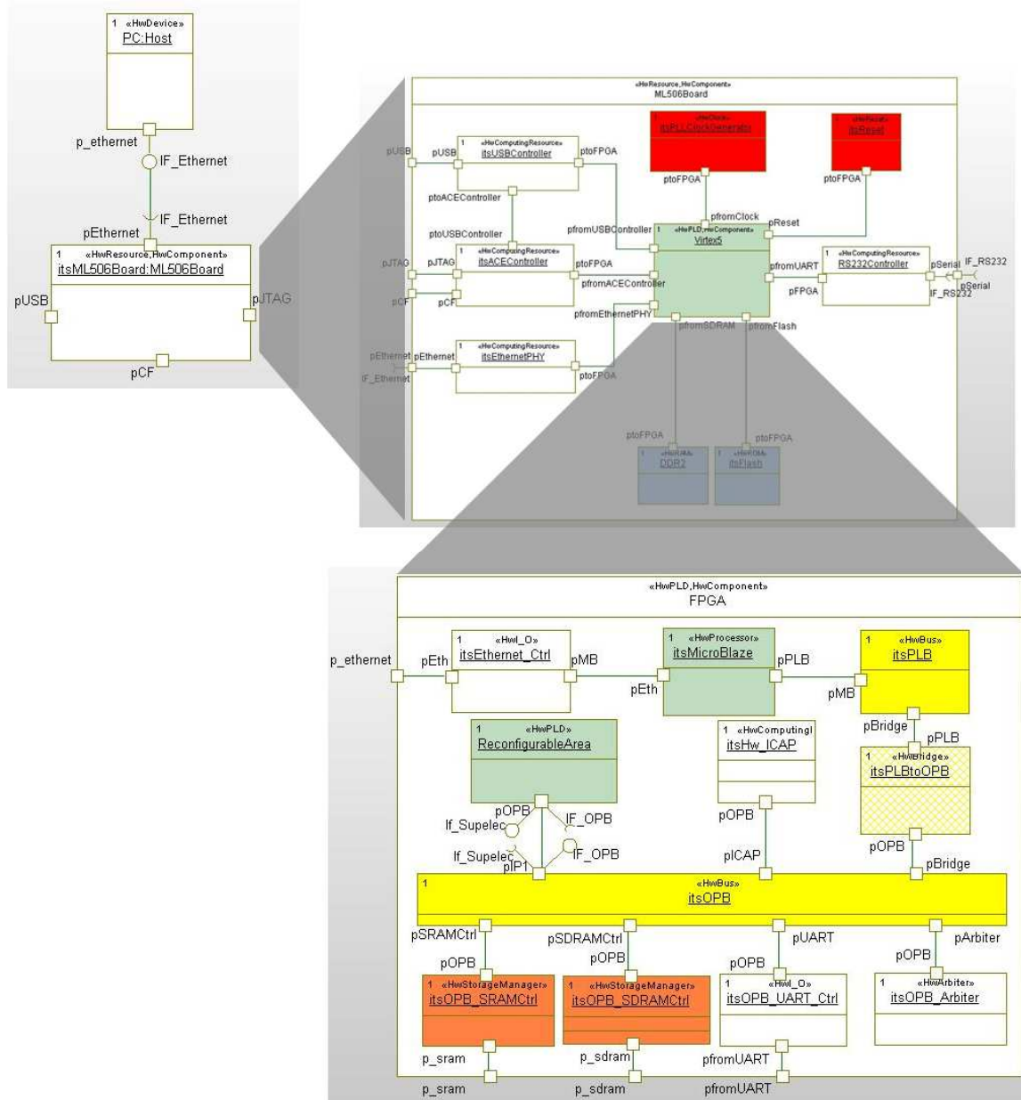
Figure 91. Extrait d'un modèle PM d'une plateforme matérielle reconfigurable basée sur un FPGA.
