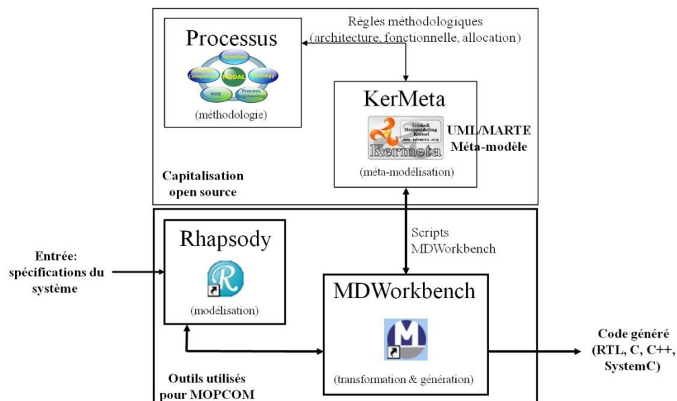
Figure 35. Environnement d'outillage de la méthodologie MOPCOM.
