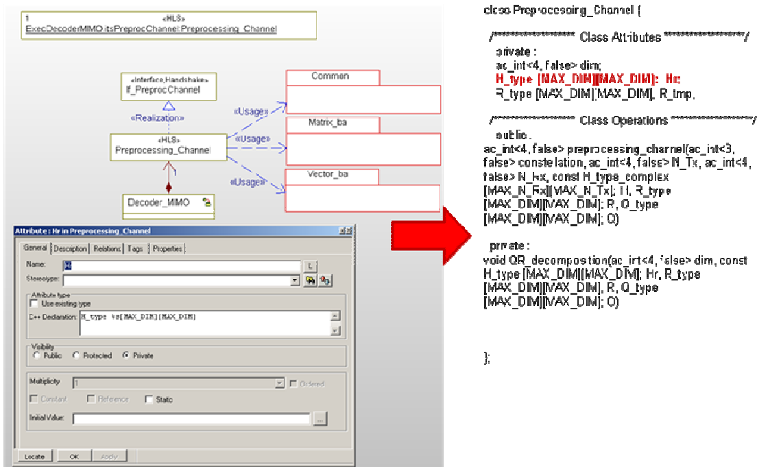
Figure 69. Exemple de génération de code de la classe « Preprocessing_Channel », stéréotypée HLS, du décodeur MIMO, ayant entre autre, un tableau à 2 dimensions comme attribut.
