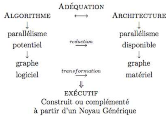
Figure 23. Illustration de la méthodologie AAA.
