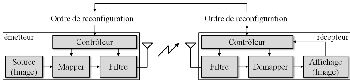
Figure 15. Synoptique du système de transmission sans-fil RLR simplifié.
