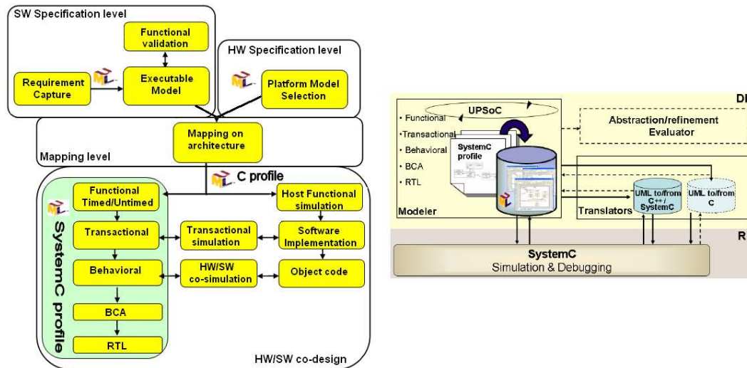
Figure 29. Méthodologie et environnement de développement UPES [81].
