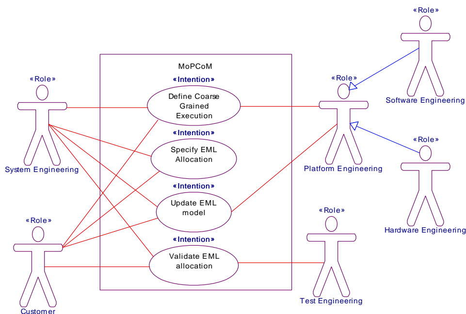
Figure 39. Diagramme de cas d'utilisation, définition des intentions du niveau EML.
