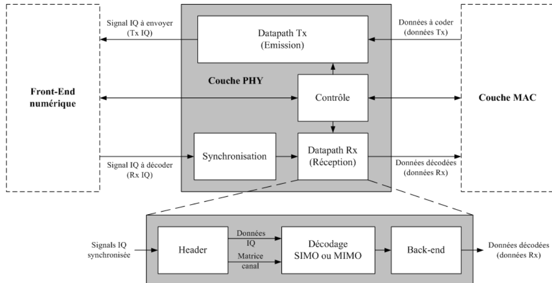
Figure 10. Synoptique de la couche PHY.
