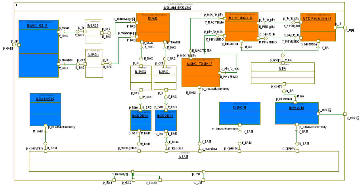
Figure 56. Diagramme de composition représentant une vue interne de l'architecture du FPGA avec les types des composants spécifiés.
