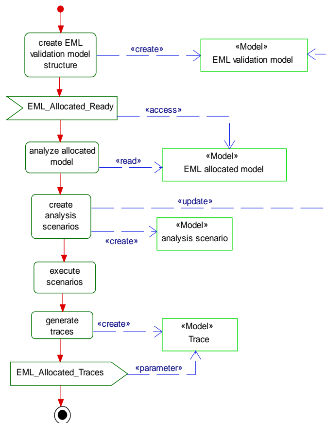
Figure 42. Diagramme d'activités illustrant la stratégie à suivre pour mettre en œuvre le cas d'utilisation « validate EML allocation ».
