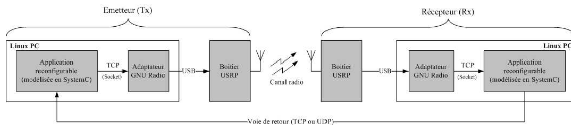
Figure 100. Synoptique du démonstrateur mettant en œuvre le système RLR présente dans le chapitre 1.
