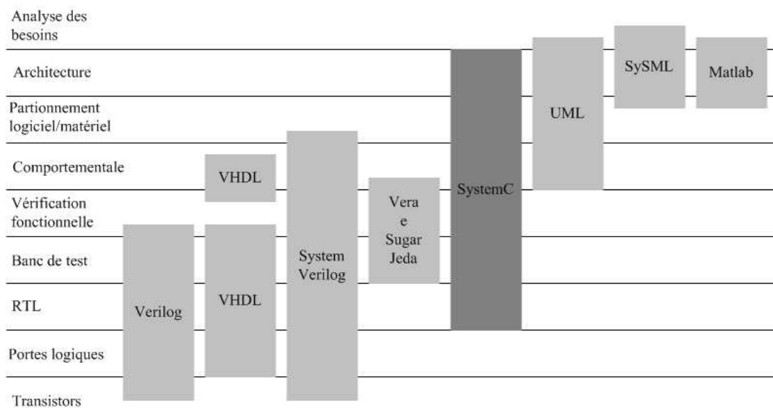
Figure 94. Positionnement du SystemC par rapport à d'autres langages utilisés dans un flot de conception de SoC Erreur ! Source du renvoi introuvable.
