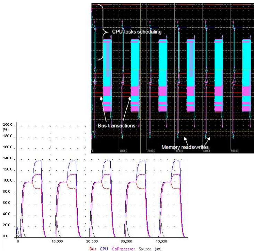
Figure 27. Extrait de résultats de simulations sous CoFluent Studio, charges des unités de calcul et analyse des transactions [75].
