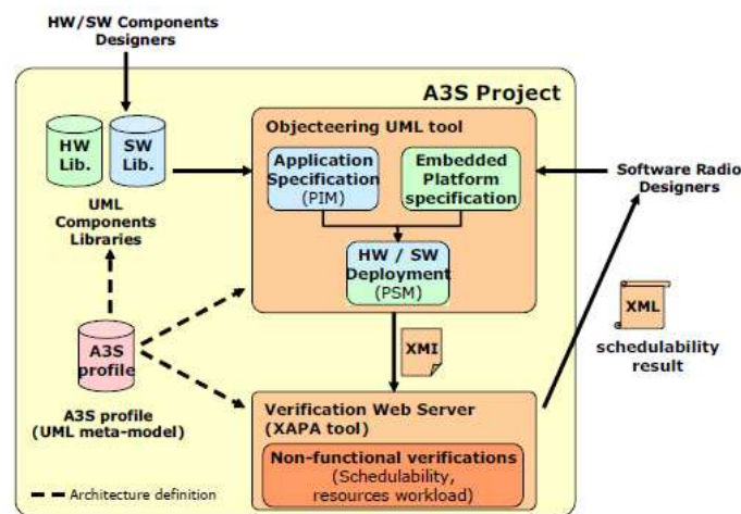
Figure 28. Environnement de modélisation du projet A3S [79].
