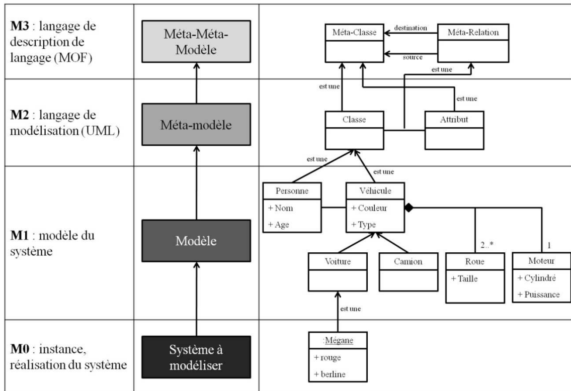
Figure 17. Représentation des couches de méta-modélisation.
