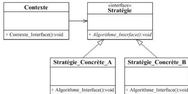
Figure 86. Méta-modèle du design pattern « Stratégie ».
