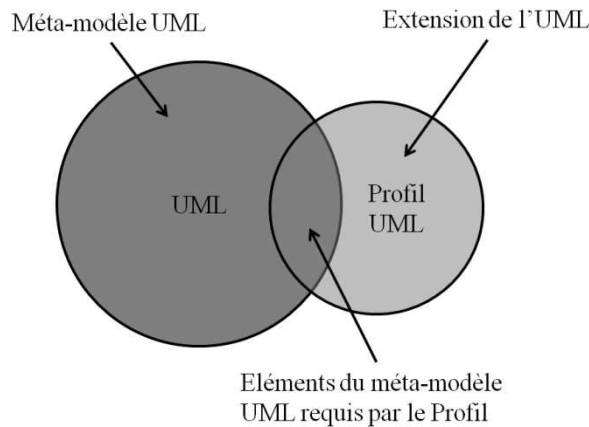
Figure 20. Extension d'UML à l'aide du mécanisme des profils.
