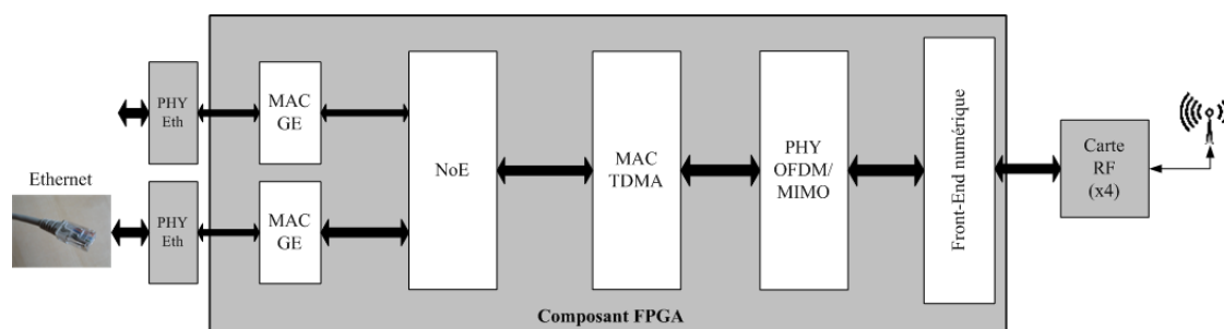
Figure 7. Nœud TxRx d'une transmission sans-fil.
