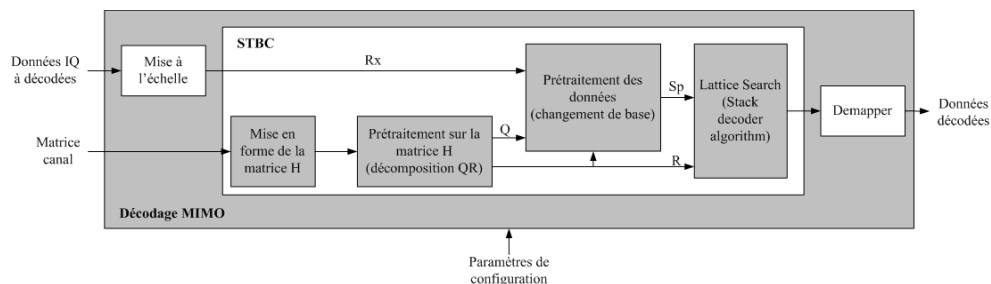
Figure 11. Architecture fonctionnelle du décodeur MIMO.
