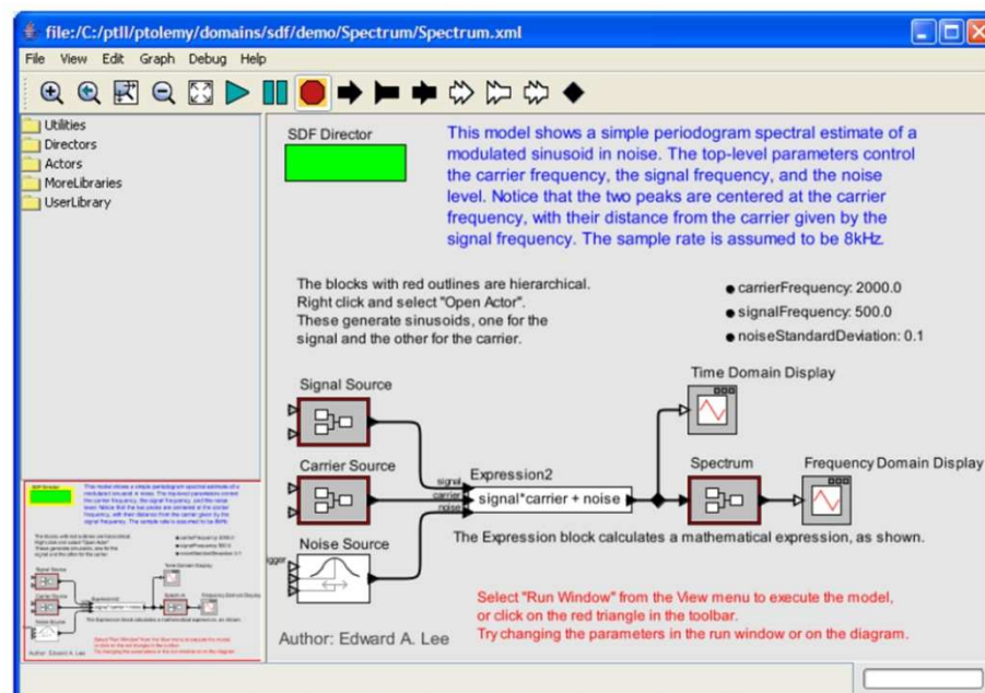
Figure 24. Vue générale de l'environnement Ptolemy.
