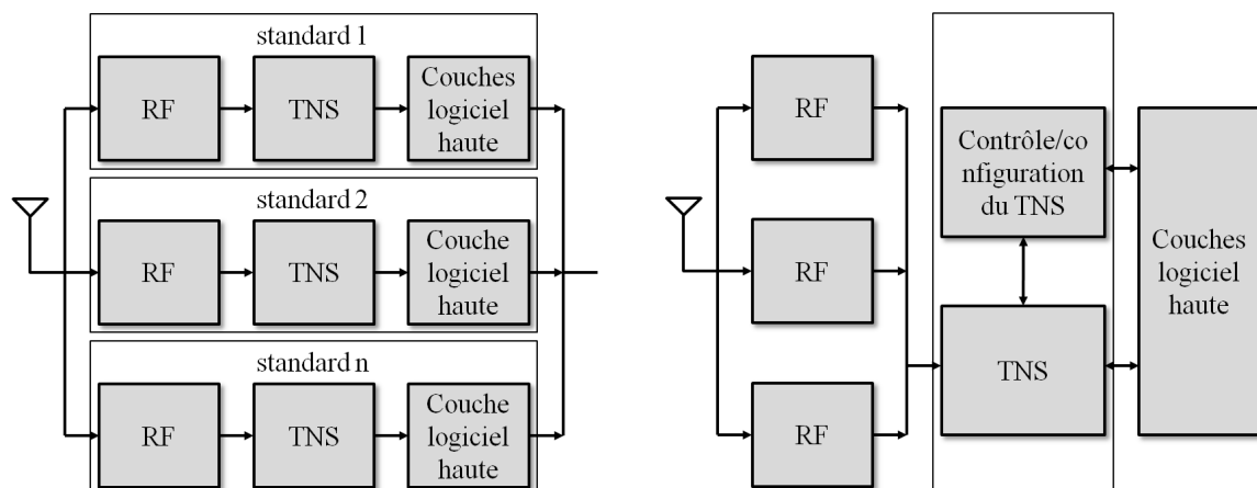
Figure 14. Architecture superhétérodyne et RLR d'un système de radiocommunications multistandards.
