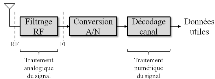
Figure 12. Architecture fonctionnelle idéale d'un système radio logicielle (RL).
