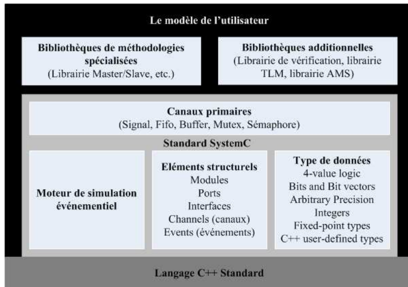
Figure 93. Architecture en couche de la librairie SystemC Erreur ! Source du renvoi introuvable.
