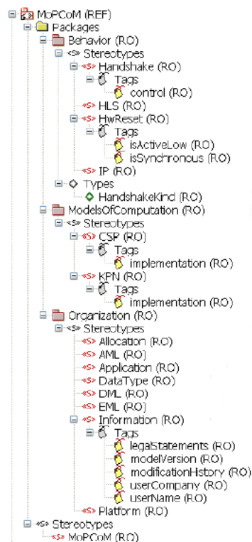
Figure 38. Illustration du profil MOPCOM.
