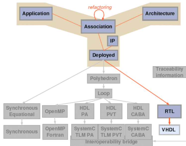
Figure 30. Flot de co-conception basé MDA dans l'environnement GASPARD.
