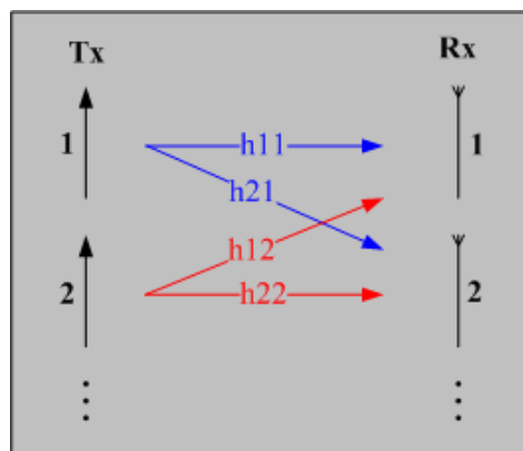
Figure 9. Modèle d'un canal MIMO.
