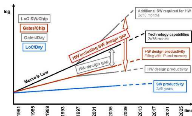
Figure 3. Evolution de la productivité en comparaison de l'évolution de la capacité d'intégration selon Moore[1].
