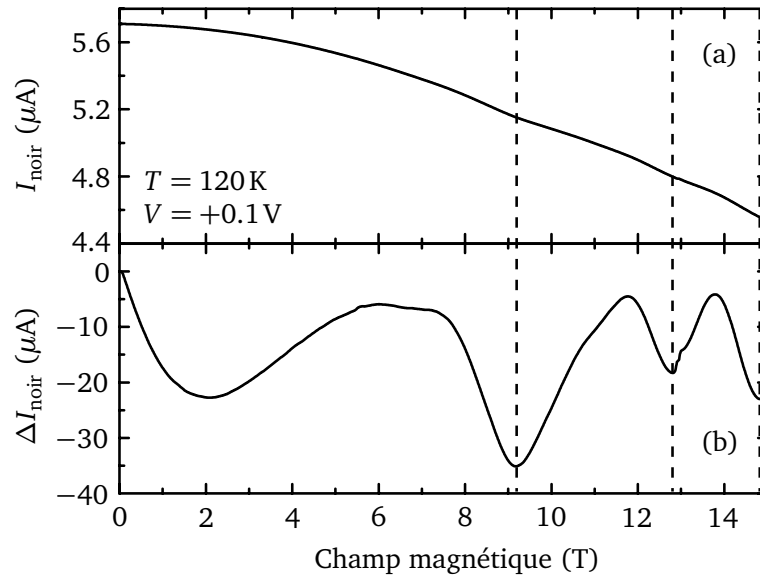
FIGURE 4.11 – (a) Courant noir I_{\text{noir}} en fonction du champ magnétique pour une valeur fixée de la tension V = 0.1\text{ V} à T = 120\text{ K} . (b) Courant noir en fonction du champ magnétique où la contribution de la magnéto-résistance des contacts a été soustraite. D’après la référence [54].
