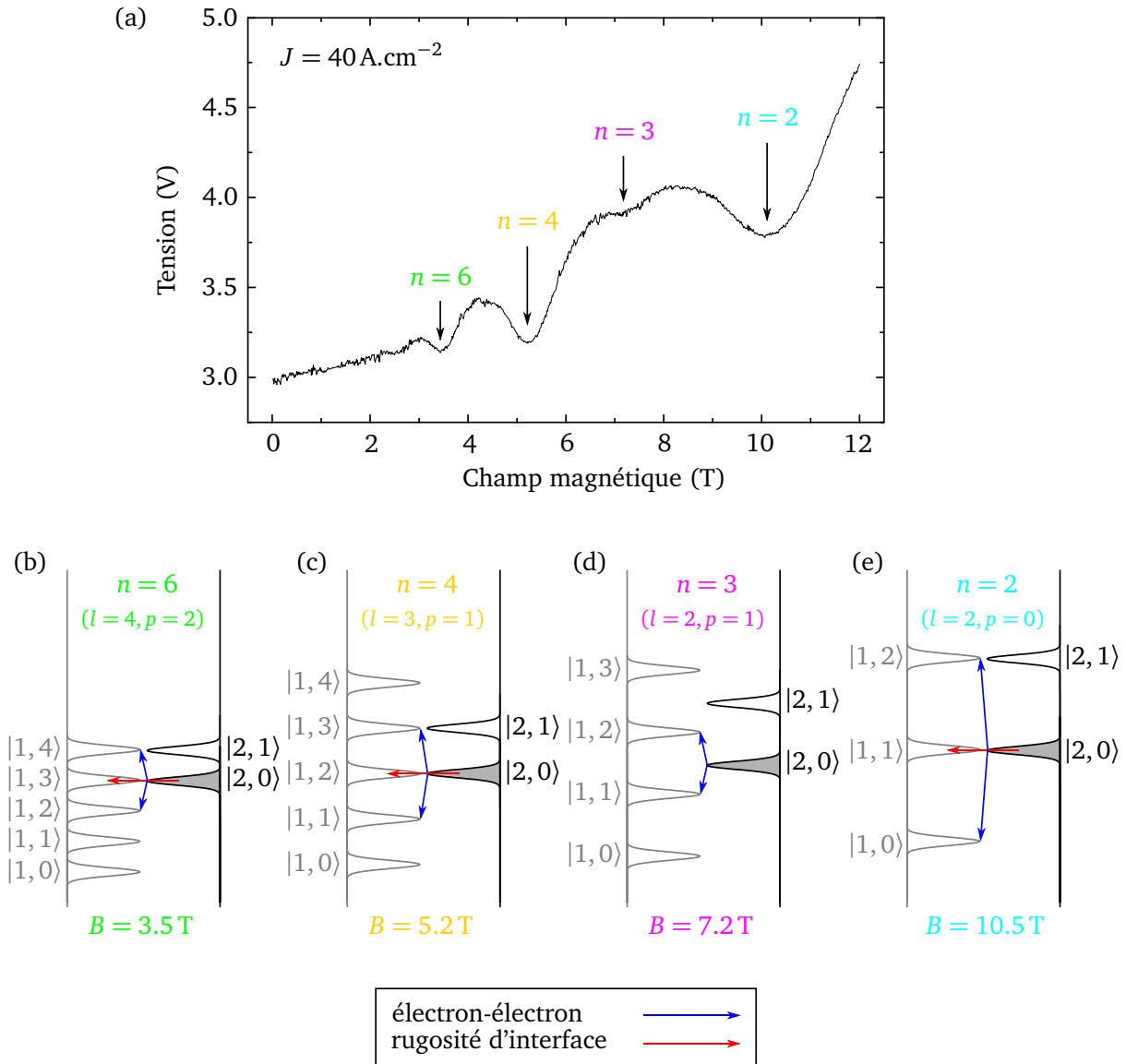
FIGURE 3.22 – Magneto-transport sur le mesa a courant fixé. (a) Tension en fonction du champ magnétique à densité de courant constante J = 40 \text{ A.cm}^{-2} . L'expérience a été réalisée à T = 4.5 \text{ K} le champ magnétique étant balayé de 0 à 12 T. Le QCS est alimenté par des pulses de largeur w = 1 \mu\text{s} avec un taux de répétition \nu_{\text{rép}} = 800 \text{ kHz} (rapport cyclique de 80 %). La surmodulation est f = 470 \text{ Hz} et la vitesse de balayage du champ magnétique est de 1 T/min. (b)-(e) Structure électronique à différents champs magnétiques des niveaux de Landau |2,0\rangle et |1,j\rangle . L'élargissement inhomogène des niveaux de Landau vaut \delta = 1.5 \text{ meV} . Deux mécanismes élastiques sont représentés : l'interaction électron-électron (flèches bleues) et la rugosité d'interface (flèches rouges). La rugosité d'interface joue un rôle pour le transfert des électrons à B = 3.5, 5.2 et 10.5 \text{ T} pour les valeurs paires de n ( n = l + p ). La diffusion électron-électron se produit dans tous les cas.
