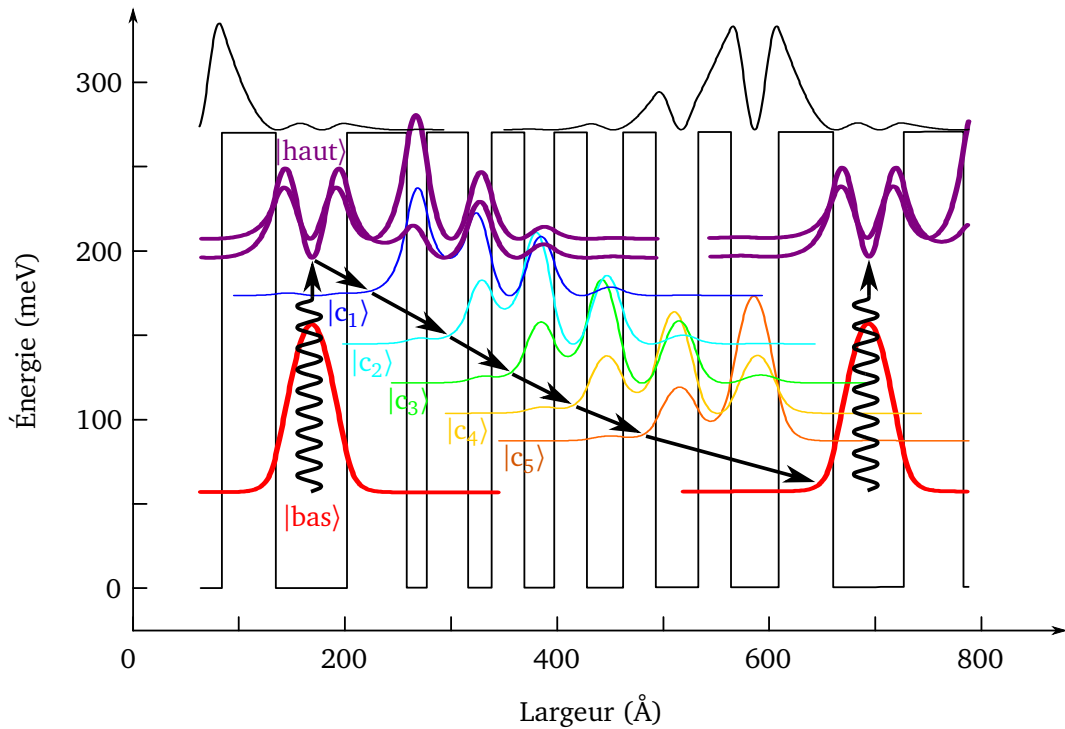
FIGURE 4.4 – Diagramme de la bande de conduction d’une période et module carré des fonctions d’ondes du QCD étudié. L’absorption optique a lieu entre le niveau |bas\rangle et le niveau |haut\rangle à la longueur d’onde 8\ \mu m . Les flèches indiquent le chemin électronique dans la structure lors de la détection d’un photon MIR. L’empilement des couches en partant du premier puits quantique est le suivant (en angström) : 68/57/20/40/23/31/28/31/34/31/40/31/45/51 (les barrières en Al_{0.34}Ga_{0.66}As sont en gras). Le premier puits est dopé n au Si à 5 \times 10^{11}\ cm^{-2} .
