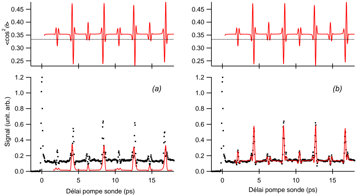
Fig. 4.10: Mesure obtenue par défocalisation croisée ( \bullet ) dans l'azote à température ambiante à un éclairement crête de 58 \text{ TW.cm}^{-2} pour une impulsion de durée 100 fs. Les ajustements numériques ( - ) dans le cas où le paramètre F est (a) fixé à zéro et (b) est numériquement ajusté. Les degrés d'alignements correspondants sont présentés sur les graphiques du dessus.
