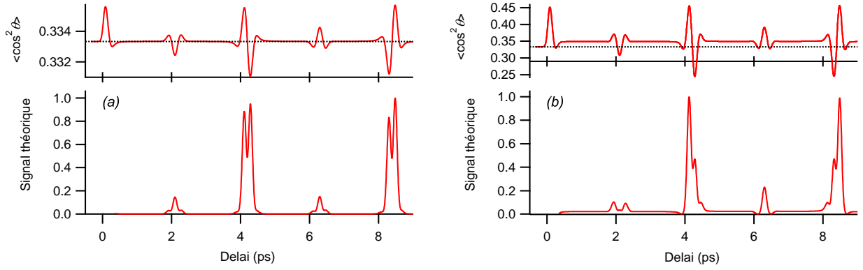
Fig. 3.5: Effet de l'hétérodynage de l'alignement transitoire par l'alignement permanent dans l'azote à température ambiante pour des éclairages théoriques de (a) 1 \text{ TW.cm}^{-2} et (b) 50 \text{ TW.cm}^{-2} et une durée d'impulsion de 100 fs. Les graphiques du dessus montrent les degrés d'alignement et ceux en dessous, les signaux théoriques de la technique de polarisation 1D.
