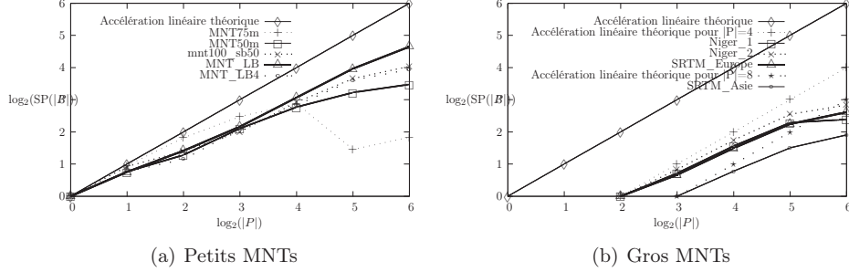
FIGURE 7.8 – Accélération relative en fonction du nombre de processeurs ( |P| )
