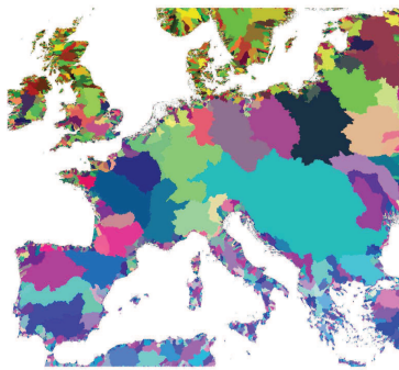
(a) Bassins versants en Europe sur ParaFlow (b) Bassins versants réels ( Source Wikipedia CC )
