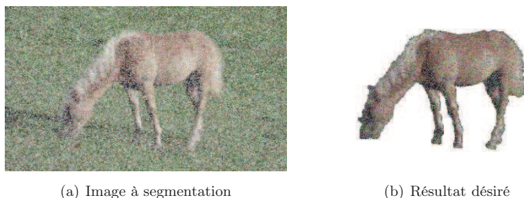
FIGURE 3.1 – Segmentation d'Images dans la Morphologie Mathématique
