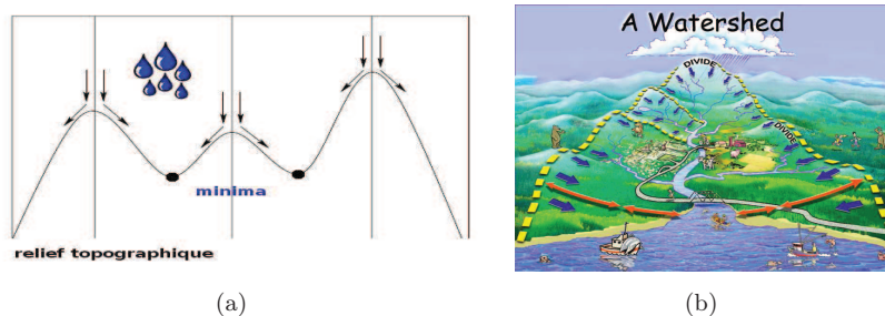
FIGURE 3.3 – Simulation de pluie dans la LPE
