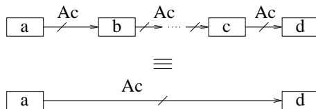
Fig. 3-18 – Equivalence d'une chaîne de liens inconditionnels. Chaque groupe de neurone effectue une compétition tout en étant relié au suivant par un lien de "1 vers 1".
