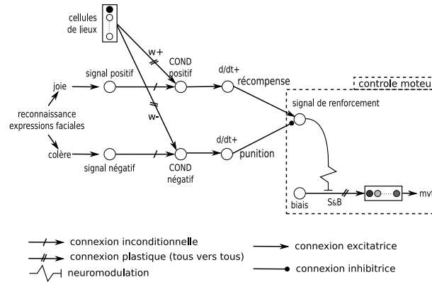
Fig. 8-9 – Modèle du couplage environnemental. En utilisant la règle d'apprentissage des moindres carrés, le conditionnement des neurones permettent l'association entre une cellule de lieux (une zone de l'environnement) et l'expression faciale de l'expérimentateur (modification des poids w^+ et w^- ). La dérivée temporelle du signal expressif prédit est utilisée comme un signal de renforcement (règle d'apprentissage de Sutton&Barto) pour maintenir ou changer la direction du robot mobile. Le lien modifiable entre le biais et le groupe S\&B permet l'apprentissage du mouvement à prendre par le robot.
