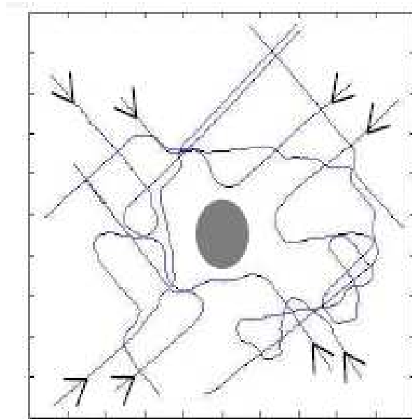
Fig. 8-11 – Les trajectoires du robot ayant pour origine différents points de départ (au départ le robot à une direction fixe) après un apprentissage interactif de la zone grise. La zone grise est associée à une expression faciale négative (l'expression de colère) ce qui implique que le robot est capable de fuir ou d'éviter cette zone. La prédiction d'un renforcement négatif est suffisante pour inhiber un mouvement dans une direction, la zone de danger peut dans ce cas être évitée.
