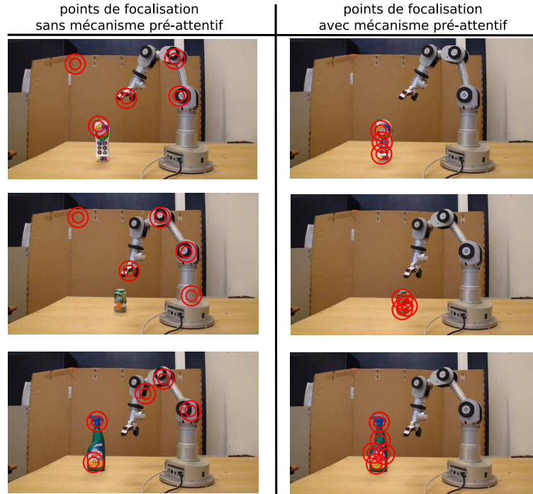
Fig. 7-11 – Processus visuel avec ou sans mécanisme de vision pré-attentive.
