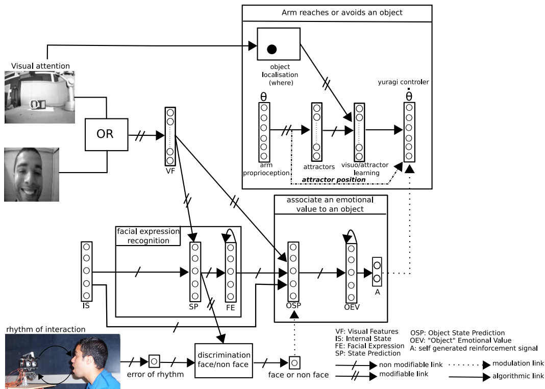
Fig. 7-3 – Modèle de référencement social. Le référencement social émerge des interactions sensori-motrices entre la reconnaissance des expressions faciales, l'attribution de valeur à des objets et l'apprentissage visuo-moteur pour le contrôle du bras robotique. Notre modèle architectural est capable d'apprendre et de reconnaître les expressions faciales ainsi que de discriminer si un partenaire interagit avec lui (détection d'un visage). Le robot focalise sur les objets grâce à un mécanisme pré-attentionnel très rudimentaire utilisant des caractéristiques issues des filtres de Gabor et de la couleur. Après l'apprentissage visuo-moteur, le bras robotique peut dans son espace de travail attraper ou s'éloigner de certains objets qui lui procurent du plaisir ou réciproquement du déplaisir et ceci grâce à un signal de renforcement auto-généré nommé A (valeur émotionnelle venant de la reconnaissance d'expression faciale). A est construit comme la conséquence directe de la reconnaissance des expressions faciales ( A_1 est le neurone correspondant à l'expression faciale de joie, A_2 est le neurone correspondant à l'expression faciale de colère). "OR" signifiant simplement qu'une seule image est analysée à la fois.
