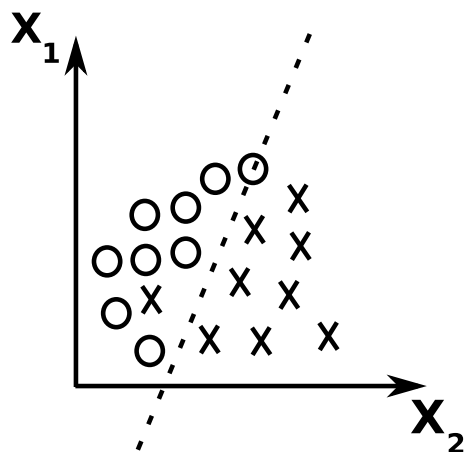
Fig. 3-8 – Hyperplan séparant deux classes dans un problème non linéaire. La règle d'apprentissage de Widrow est capable de déterminer cette frontière dans le cas d'un problème non linéaire. La frontière s'est adaptée en fonction de la non linéarité introduite par les entrées.
