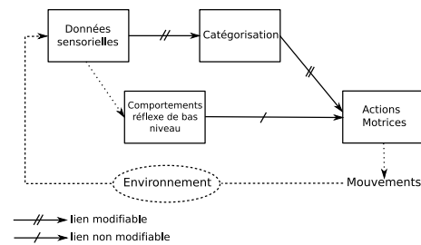
Fig. 3.12 – Schéma de la l'architecture PerAC (Perception/Action).
