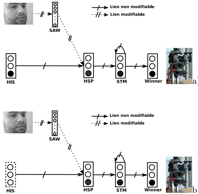
Fig. 9-6 – Architecture capable d’apprendre et de reconnaître la direction du regard de l’expérimentateur. a) représente l’architecture avant l’apprentissage, les flèches pointillés montrent les poids synaptiques n’influençant pas la reconnaissance de l’orientation du regard. Le robot n’a pas encore appris l’association entre ses mouvements oculaires et les caractéristiques visuelles décrivant la direction du regard de l’expérimentateur. b) montre l’architecture après l’apprentissage, la voie correspondant à la reconnaissance de la direction du regard (lien modifiable) est suffisante pour déclencher des mouvements oculomoteurs. La boîte en pointillée correspond à l’inhibition de l’orientation réflexe du regard. 2 neurones codent pour deux positions extrêmes (regard à droite et à gauche) et le troisième neurone code pour la position neutre correspondant à l’expérimentateur regarde en face.
