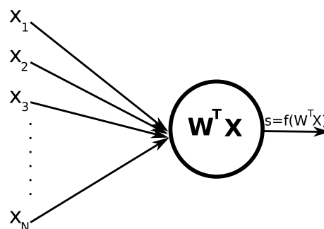
Fig. 3-3 – Schéma d'un neurone formel. Neurone formel de Mc. Culloch et Pitts
