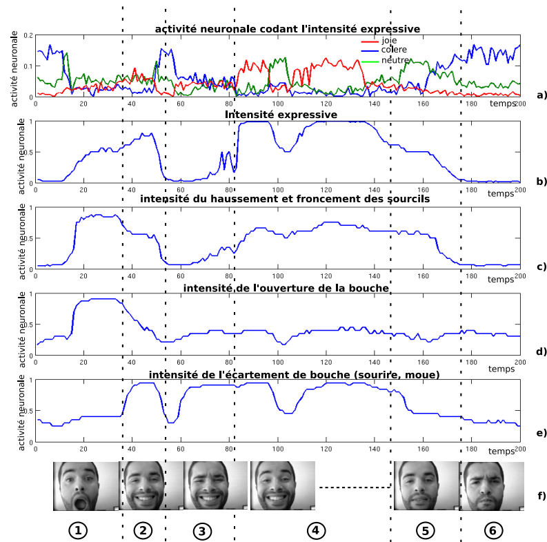
Fig. 6-14 – Résultats lors d’une séquence d’interaction en ligne avec la tête de robot expressive (le robot imite l’humain). Ces courbes montrent les différents signaux utiles à la reconnaissance des expressions émotionnelles, cependant ces dernières n’influencent pas la reconnaissance des intensités motrices. a) montre l’activité neuronale des 3 neurones codant pour les 2 expressions faciales (joie et colère) et le visage neutre. b) montre l’effet du neural field sur la reconnaissance des intensités expressives émotionnelles. c) montre l’effet du neural field sur la reconnaissance des intensités motrices pour le haussement et froncement des sourcils. d) montre l’effet du neural field sur la reconnaissance des intensités motrices pour l’ouverture de la bouche. e) montre l’effet du neural field sur la reconnaissance des intensités motrices pour les coins de la bouche (sourire et moue). f) montre la séquence d’image analysée.
