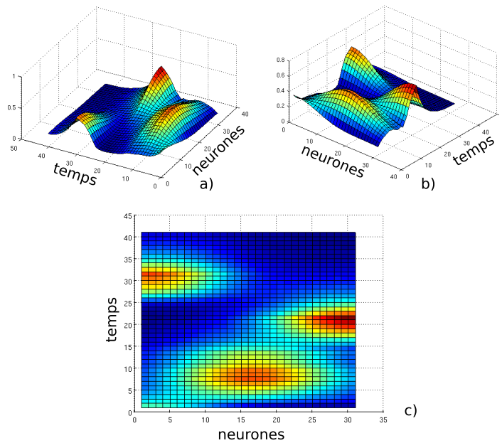
Fig. 9-11 – Activité temporelle du champ de neurone. Les courbes a) b) c) montrent l’activité temporelle du champ de neurones lors d’une séquence d’orientation de regard.
