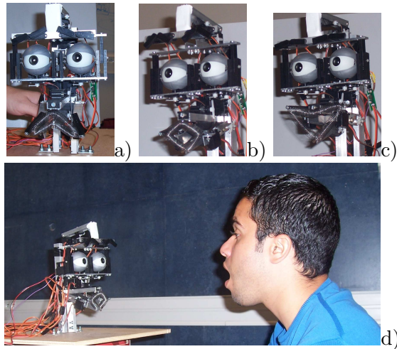
Fig. 4-1 – Exemples d’expressions faciales que le robot est capable de reproduire: a) tristesse, b) surprise, c) joie. d) situation typique du robot et de l’humain dans le cas d’un jeu d’interaction.
