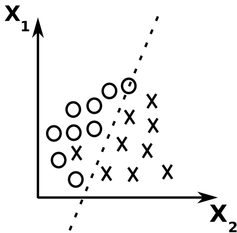
Fig. 3-8 – Hyperplan séparant deux classes dans un problème non linéaire. La règle d'apprentissage de Widrow est capable de déterminer cette frontière dans le cas d'un problème non linéaire. La frontière s'est adaptée en fonction de la non linéarité introduite par les entrées.
