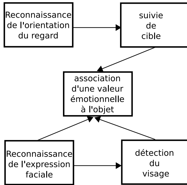
Fig. 9-15 – Schéma bloc: prémices d'attention conjointe dans un contexte de référencement social. La reconnaissance des expressions faciales, l'attribution de valeur émotionnelle à des objets et la reconnaissance de la direction du regard permet de donner un sens émotionnel à l'objet lors d'une interaction avec un expérimentateur.
