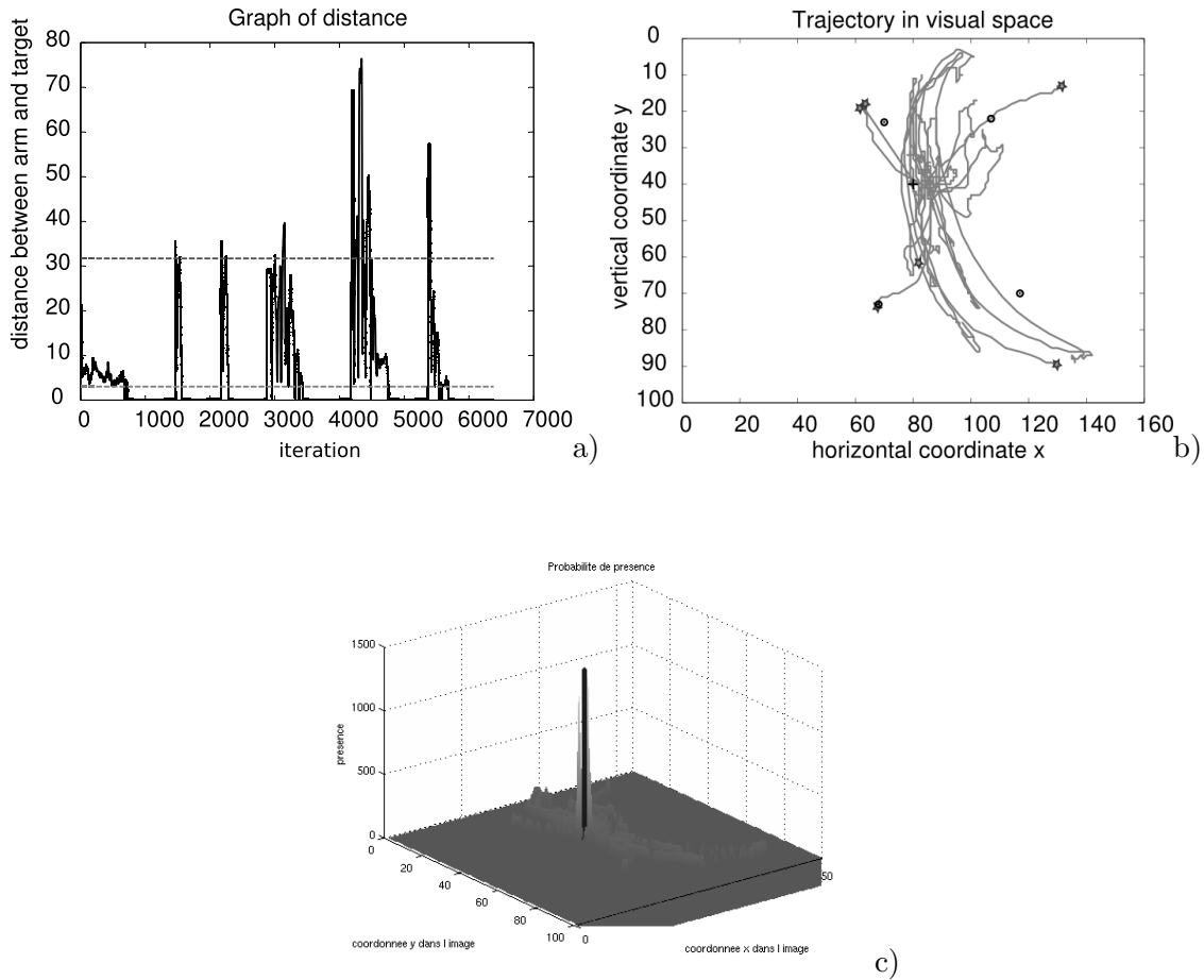
Fig. 7-18 – Trajectoire montrant la convergence du bras robotique. a) montre la distance à la cible. b) montre la trajectoire du bras robotique lorsque la cible à rejoindre est entre plusieurs attracteurs. Les cercles noirs correspondent aux différents attracteurs appris. La croix correspond à la cible à rejoindre et les étoiles correspondent aux différents points de départ. Quatre attracteurs sont activés. c) montre l’histogramme de la trajectoire (endroit où se situe le bout de la pince). Le pic noir est la cible à rejoindre et les pics blancs correspondent à la présence du bout de la pince.
