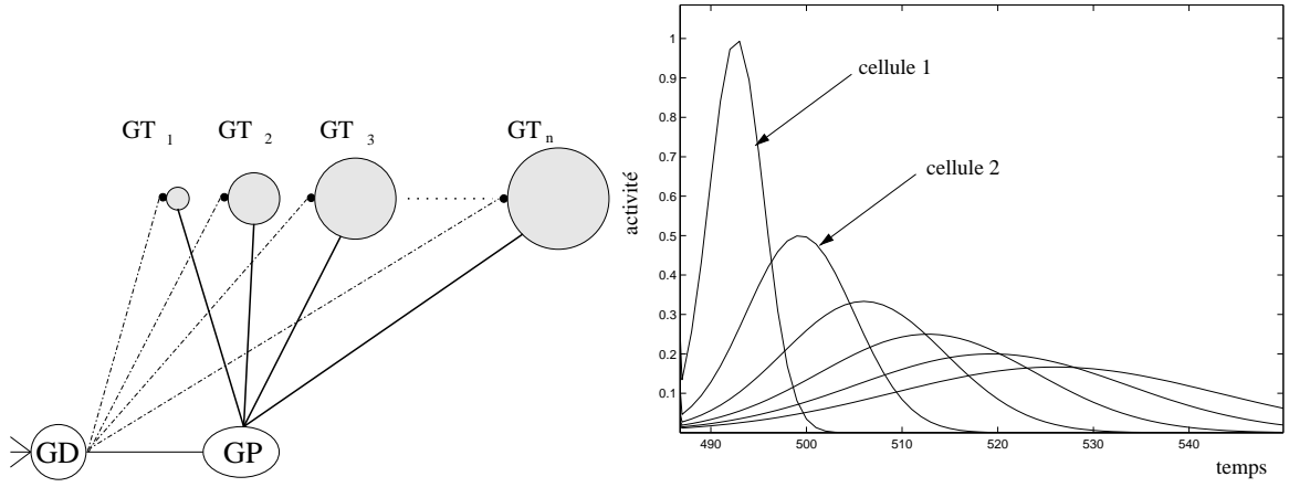
Fig. 5-2 – A Gauche: Détail des connexions entre un neurone GD , une batterie de neurones GT et un neurone GP . A droite: courbes d'activité de 6 cellules d'une ligne du groupe temporel. La ligne est activée à t=485 s, et chaque cellule décharge dans le temps, permettant de conserver une trace à court terme de l'événement (ici sur une minute environ)
