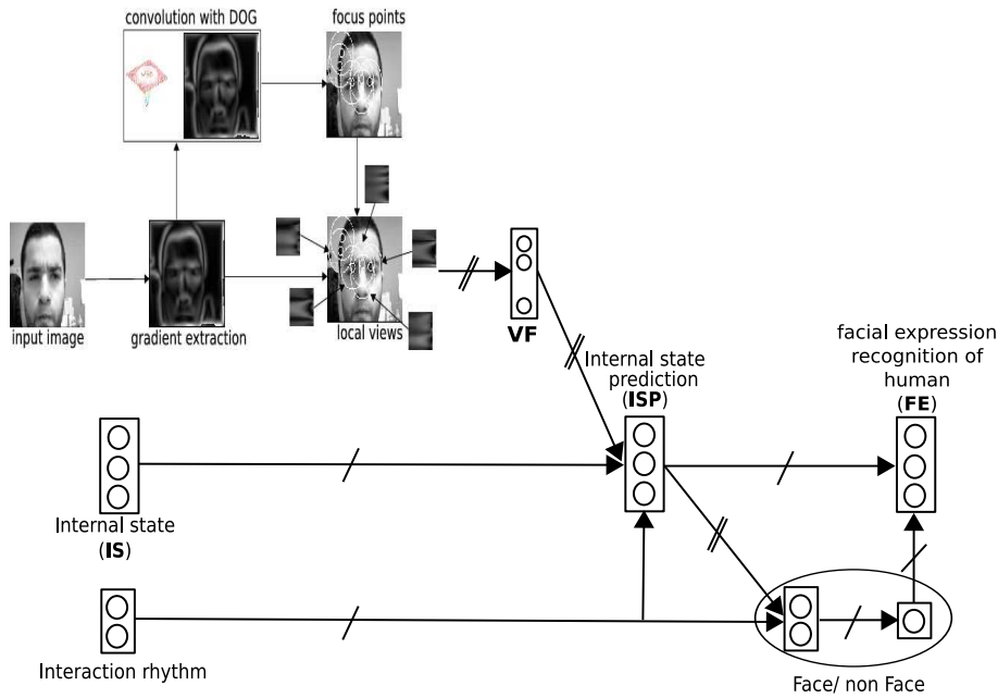
Fig. 7.4 – Modèle intégrant la reconnaissance des expressions faciales et la détection de visage.
