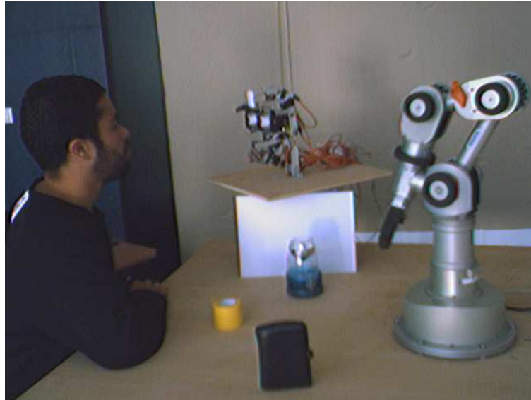
Fig. 7-1 – Set-up expérimental pour le référencement social. Nous utilisons une tête robotique capable de reconnaître et d'imiter les expressions faciales et un bras robotique capable de prendre des objets à valence positive ainsi que de s'éloigner des objets dits négatifs.
