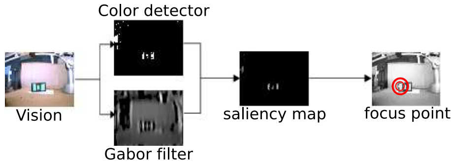
Fig. 7-7 – Vision pré-attentive. Le robot peut focaliser sur certains objets dans l'espace de travail. Une carte de saillance est activée pour focaliser sur les zones intéressantes de l'image. Les primitives visuelles calculées indépendamment (couleur, caractéristiques issus de filtres de Gabor) sont fusionnées par la suite pour trouver la zone que le robot doit analyser.
