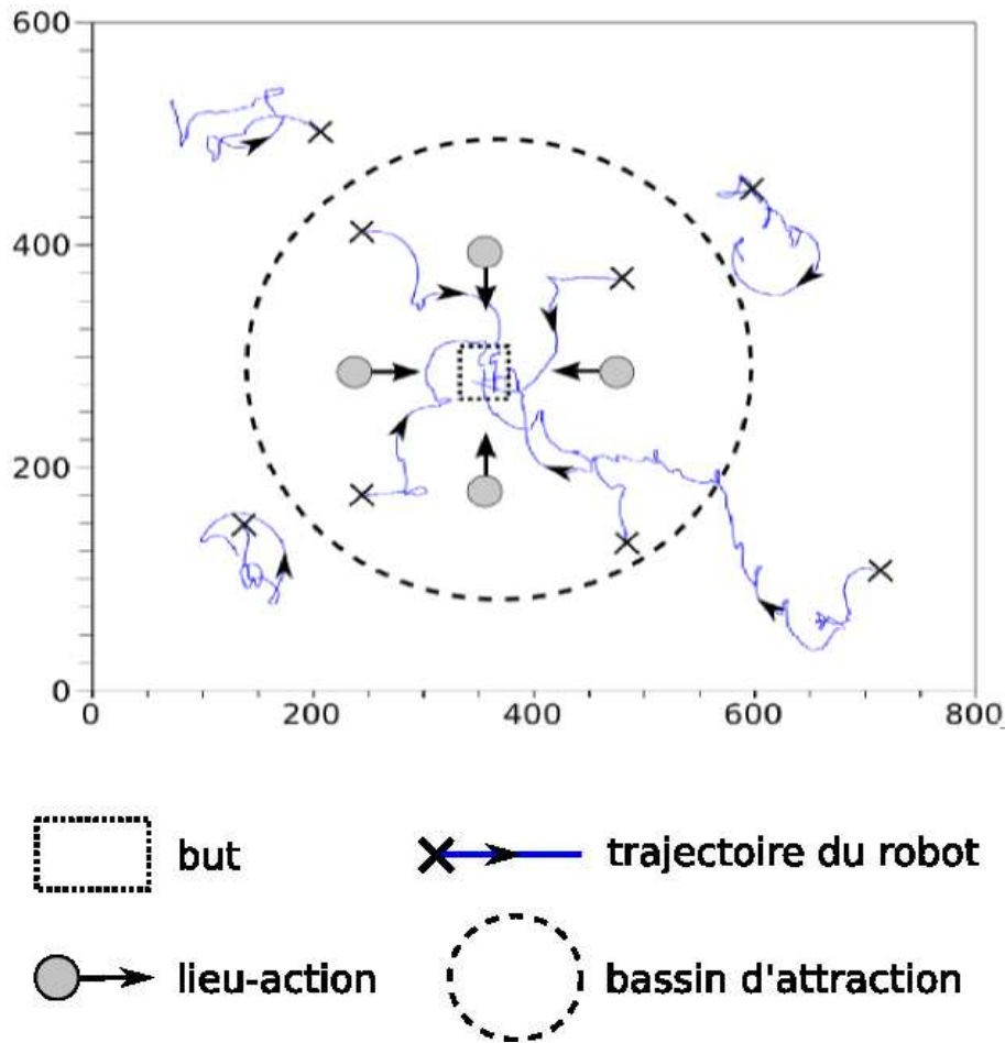
Fig. 8-5 – Trajectoires du robot ayant appris un bassin d'attraction autour d'un but. Le robot a appris quatre couples lieu-action convergeant vers un but. Quand il est dans le bassin d'attraction, ses actions le rapprochent de son but. En dehors du bassin d'attraction, le robot navigue aléatoirement. Il est possible que le robot rejoigne le bassin d'attraction mais cela repose sur le hasard et non sur un apprentissage.
