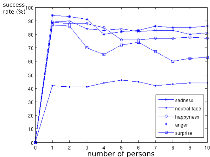
Fig. 4-13 – Le taux de succès pour chaque expression faciale (tristesse, joie, colère, surprise et visage neutre) avec la transformée log-polaire. Ces résultats sont obtenus durant une interaction naturelle avec la tête robotique. 10 personnes ont interagi avec le dispositif robotique (32 images par expressions par individus). Durant la phase d’apprentissage (2 minutes d’interaction), les individus doivent imiter le robot et une fois cette phase d’apprentissage finie l’on bascule le système en mode reproduction où le robot dans ce cas doit imiter l’humain. Pour fabriquer les statistiques, chaque image a été annotée en fonction de la réponse du robot. Les images annotées ont été analysées pour vérifier s’il y avait correspondance entre l’expression réalisée par le robot et celle réellement exprimée par l’humain.
