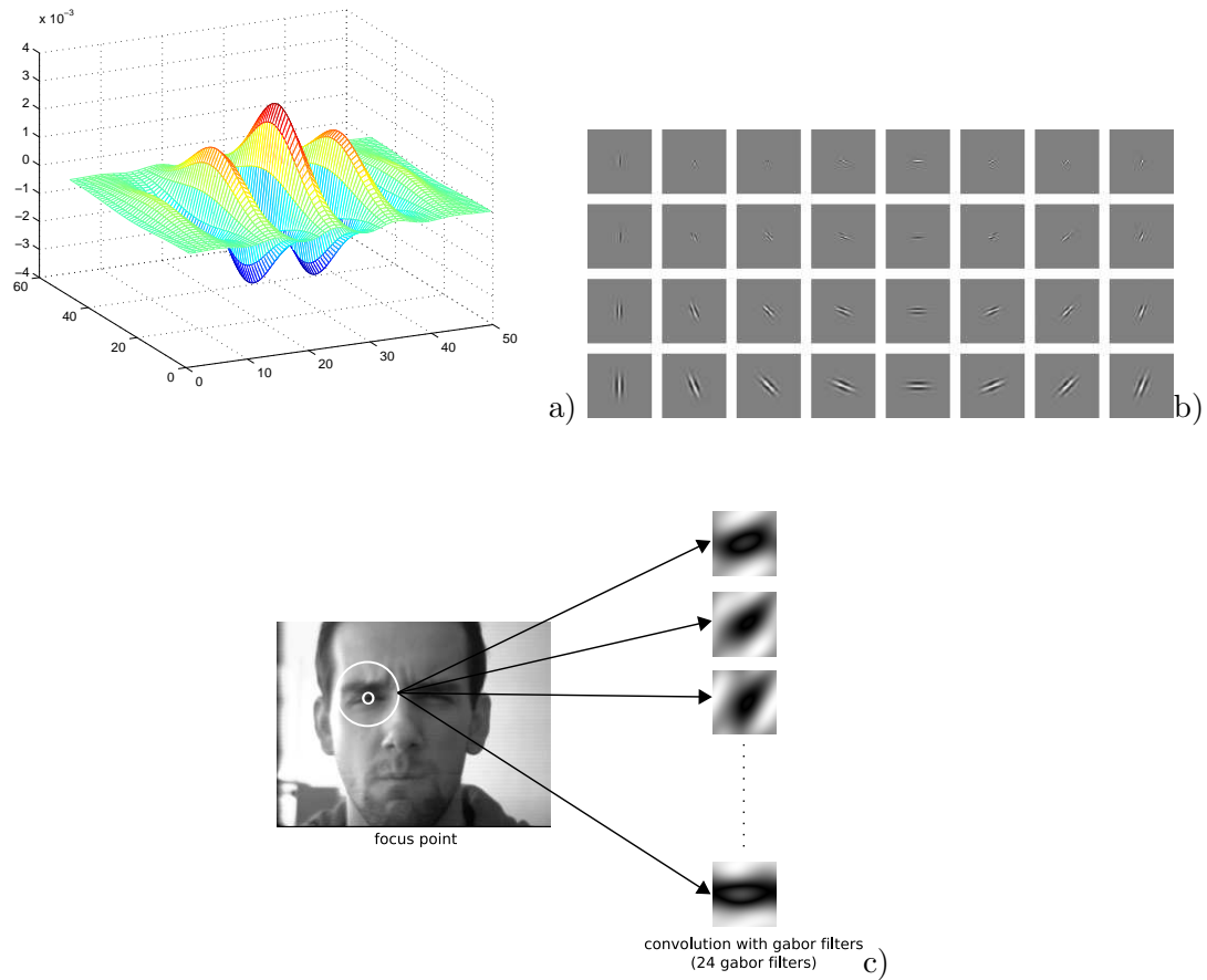
Fig. 4-10 – Visualisation du processus utilisant les filtres de Gabor. a) montre un filtre de Gabor avec les paramètres suivant \sigma = 8 , \gamma = 3 , \theta = \pi/3 . Visualisation d’une Gabor dans un espace 3 dimensions. b) montre différents filtres de Gabor avec différentes orientations et fréquences. Enfin c) montre le résultat d’une convolution avec les 24 filtres de Gabor utilisés pour un point caractéristique donné (au niveau de l’oeil).
