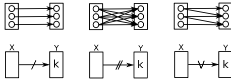
Fig. 3-15 – Schéma formalisant les 3 types de connexions entre noeuds. De gauche à droite: les connexions de 1 vers 1 (lien réflexe), les connexions de 1 vers tous (lien apprenant), les connexions de 1 vers un voisinage (lien pouvant apprendre ou projection).
