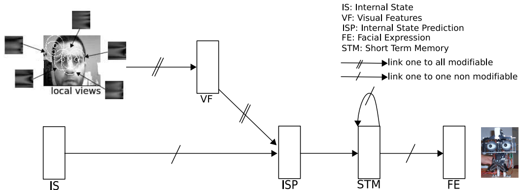
Fig. 4-6 – Architecture imitant les expressions faciales. Processus visuel permettant d'extraire les vues locales de manière séquentielle. La prédiction de l'état interne (groupe ISP ) apprend l'association entre les vues locales et l'état interne (groupe IS ).
