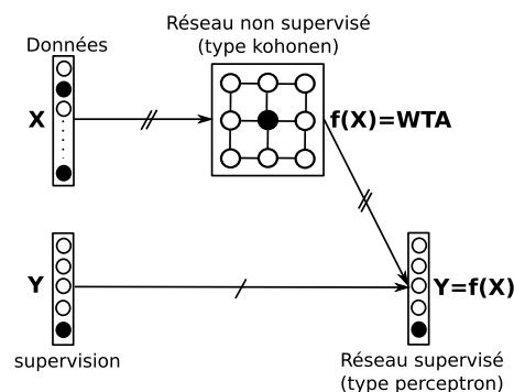
Fig. 3-11 – Schéma de la counter propagation. Architecture neuronale à deux couches. Une première couche servant de quantification vectorielle (réseau de neurone de type kohonen). Une seconde servant à catégoriser les classes déjà prédéfinies (réseau de neurone de type perceptron)
