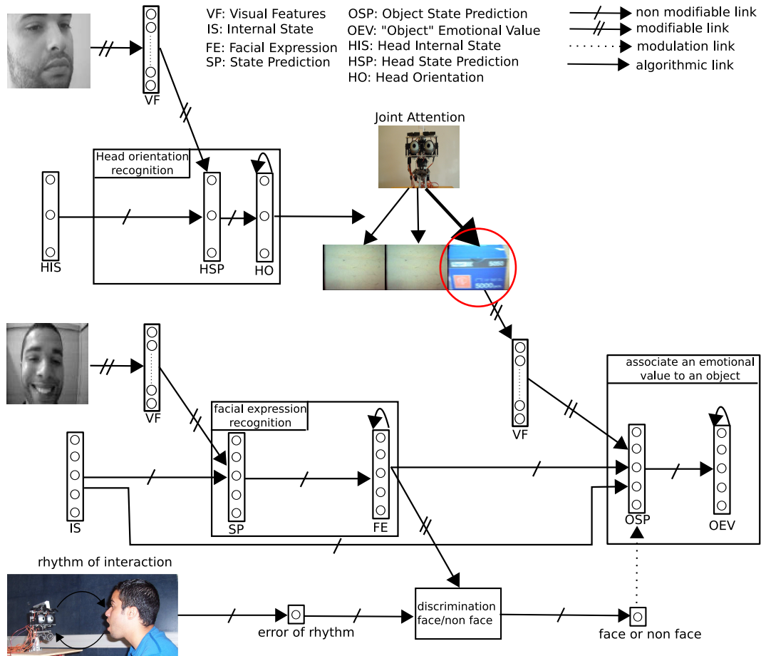
Fig. 9-16 – Modèle intégrant un prémices d'attention conjointe dans un contexte de référencement social. Les interactions sensori-motrices entre la reconnaissance des expressions faciales, l'attribution de valeur à des objets et la reconnaissance de la direction du regard permet d'une part d'orienter l'attention du robot sur un objet que regarde l'expérimentateur et d'autre part donner un sens émotionnel à l'objet. Le robot dirige son regard sur un objet en suivant celui de l'expérimentateur. Une fois que l'objet est dans le champ de vision du robot, l'expérimentateur peut communiquer de l'information grâce à l'expressivité faciale. Par conséquent, un objet peut avoir une valeur émotionnelle positive ou négative selon l'expressivité de l'expérimentateur.
