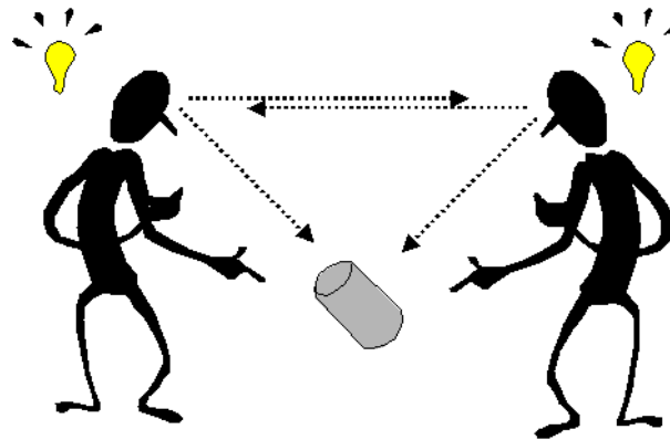
Fig. 2-5 – Attention conjointe.
