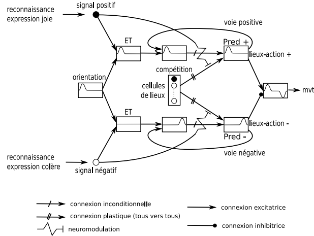
Fig. 8-6 – Modèle du couplage comportementale. Quand l’un des groupes de conditionnement Pred- ou Pred+ reçoit une neuromodulation venant de la reconnaissance des expressions faciales (dans le cas décrit, il s’agit de l’expression de joie), l’association entre la localisation courante du robot (perception d’une cellule de lieux gagnante spécifique) et sa direction courante donnée par le compas (sommée avec ce qui a déjà été appris par ce groupe de neurone dans le passé) est apprise. Les neurones correspondant aux signaux ”positifs” et ”négatifs” sont associés à la reconnaissance de l’expression faciale de joie ou de colère du partenaire social interagissant avec la tête de robot.
