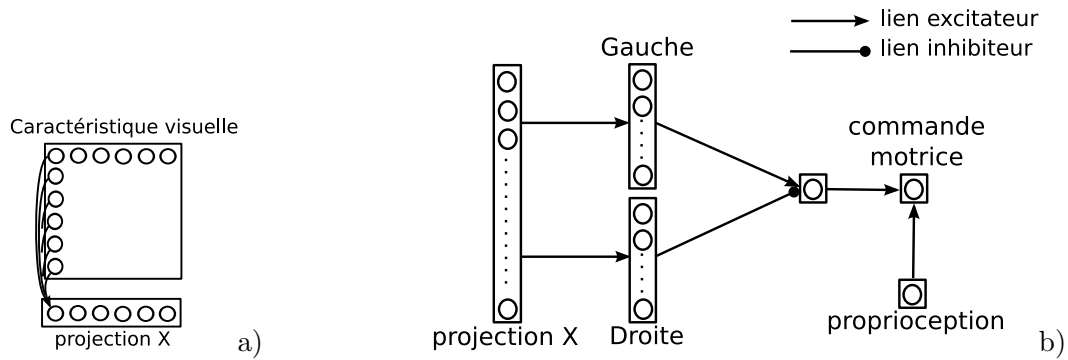
Fig. 9-13 – Architecture contrôlant le suivi d’une cible. a) montre la projection horizontale qui est réalisée grâce aux connexions synaptiques (projection neuronale). Les caractéristiques visuelles utilisées sont la couleur et les filtres de Gabor. b) montre l’architecture contrôlant le centrage d’une cible. La commande motrice correspond au degré de liberté contrôlant l’orientation du regard du robot (angle moteur correspondant au Pan ).
