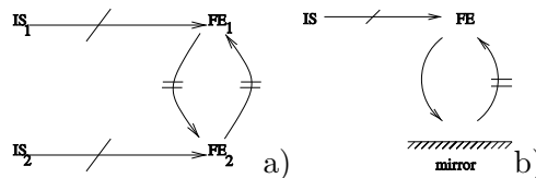
Fig. 4-5 – a) simplification finale du réseau représentant l'interaction entre nos deux agents (capacité à exprimer et comprendre des "émotions"). b) Architecture minimale permettant à l'agent d'apprendre les associations entre les "états internes" et l'expression faciale.
