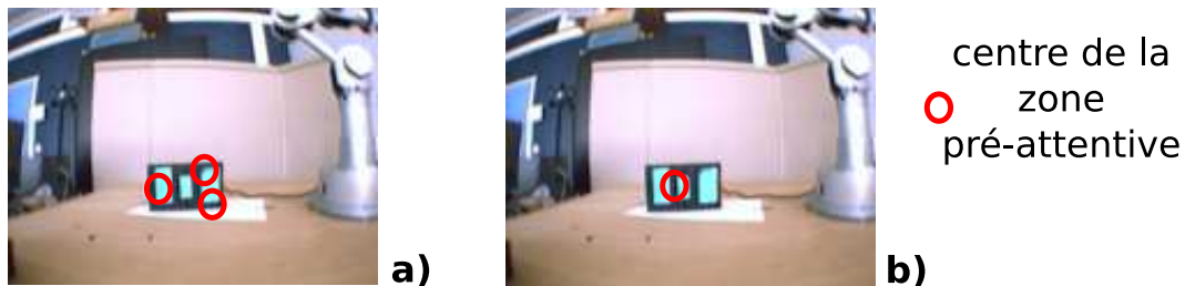
Fig. 7-10 – Les cercles rouges montrent le centre de la zone pré-attentive sélectionnée. a) montre le traitement sans le champ de neurones où le premier point trouvé change d'une image à l'autre. b) montre l'influence du champ de neurones sur la stabilité de la zone pré-attentive. Le système se stabilise sur une seule zone pré-attentive dont le centre est représenté par le cercle rouge.
