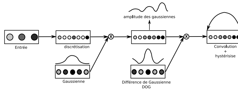
Fig. 6-6 – Modèle du Neural Field (champ de neurones). L'équation du neural field peut être facilement découpée en une succession de groupe de neurone. Les champs de neurone ont des propriétés intéressantes pour un contrôle moteur stable. Les champs de neurone sont utilisés pour obtenir un signal plus stable dans le temps (propriété temporelle) ainsi qu'une capacité de bifurcation.
