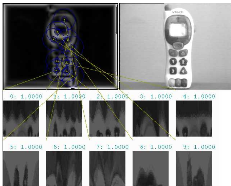
Fig. 7-12 – Traitement visuel. Le processus visuel utilisé est le même que pour la reconnaissance des expressions faciales. Les points de focalisations sont le résultat d’une convolution entre une Différence de Gaussiennes (DOG) et l’image, focalisant particulièrement sur les zones de courbures. Une transformation log-polar est utilisée pour obtenir plus de robustesse vis à vis de la vue locale.
