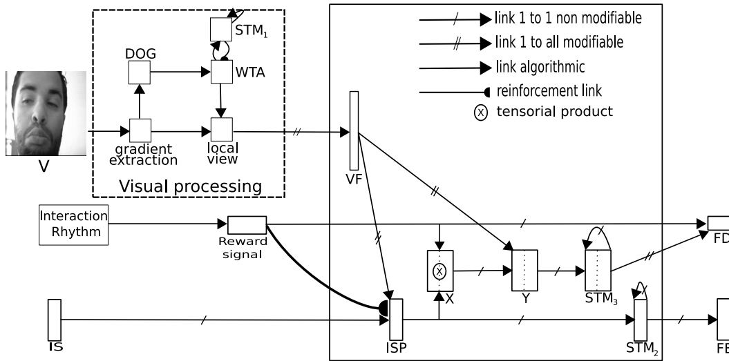
Fig. 5-8 – L’architecture globale pour reconnaître l’expressivité d’un partenaire, imiter et discriminer le visage d’un non visage. Le processus visuel permet d’extraire séquentiellement les vues locales. Le groupe VF (reconnaissance de la vue locale) apprend les vues locales. Chacun des groupes de neurones suivant IS , ISP , STM_2 et FE contiennent 5 neurones correspondant aux 4 expressions faciales et au visage neutre. Un produit tensoriel est réalisé entre ISP (prédiction de l’état interne correspondant à une sorte d’état émotionnel) et un signal de récompense sélectionnant le neurone devant apprendre. Y apprend l’association entre une vue locale et une expression faciale, un neurone spécifique est activé suivant que le lien de récompense venant de l’interaction est présent ou non. Le groupe FD (détection du visage) apprend lui l’association entre le produit tensoriel et le signal de récompense. Son activité correspond quand à elle à la reconnaissance ou au contraire à l’absence d’un visage dans la scène. Le signal de récompense permet également de moduler la vitesse d’apprentissage des expressions faciales en fonction de la situation interaction/non interaction.
