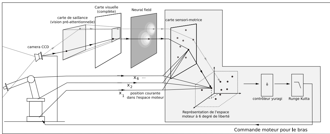
Fig. 7-15 – Modèle montrant l'architecture capable de contrôler le bras robotique à 6 degrés de liberté. La carte sensori-motrice peut apprendre à associer un stimulus visuel et des informations proprioceptives du bras de robot impliquant après apprentissage l'activation d'un ou plusieurs attracteurs dans l'espace moteur. Si la position courante du bras est différente des attracteurs sélectionnés alors une loi de commande est envoyée au bras robotisé pour atteindre la position cible. Cette loi de commande est régie par une équation dynamique (équation de Langevin): le contrôleur Yuragi.
