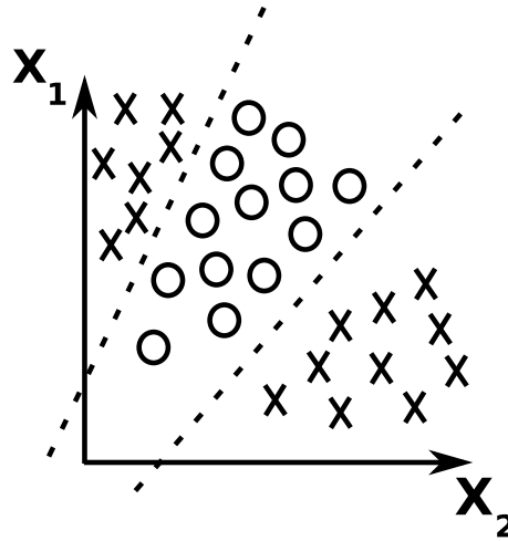
Fig. 3-9 – Hyperplans séparant deux classes dans un problème non linéaire. Le perceptron multicouche est capable de trouver plusieurs frontières à l’aide des couches cachées lorsque les motifs d’entrées sont non linéaires. Dans cet exemple, le MLP trouve deux hyperplans (ligne pointillé) séparant les deux classes.
