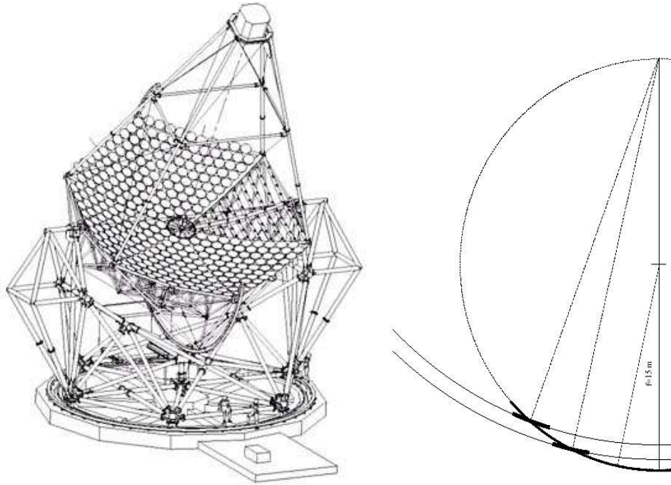
FIG. 2.6 – Gauche : Schéma d'un des télescopes de HESS. Droite : Schéma du montage Davies-Cotton utilisé pour les réflecteurs de HESS. La focale du réflecteur est 15 m. Ces figures sont tirées de [47].
