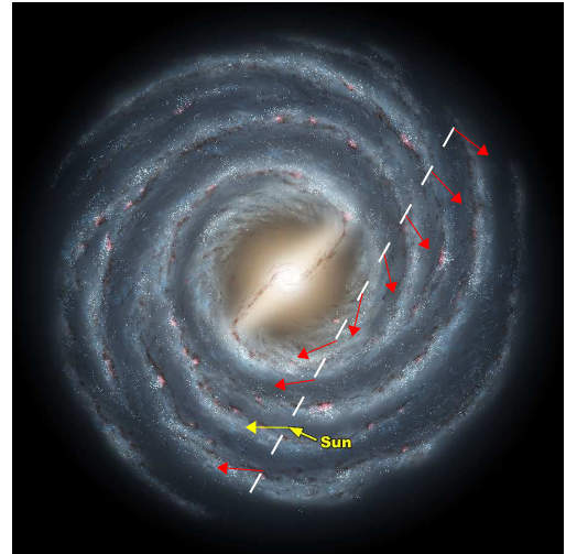
FIG. 4.5 – Gauche : Évolution de la vitesse de rotation autour du centre de la Galaxie en fonction de la distance au système Solaire. La paramétrisation est tirée de [71]. Droite : Vue schématique de la Voie Lactée telle qu'observée au travers des mesures d'abondance de l'hydrogène neutre H_I . La répartition de vitesses de rotation autour du centre de la Galaxie le long d'une ligne de visée arbitraire est représentée. La longueur des flèches est arbitraire.
