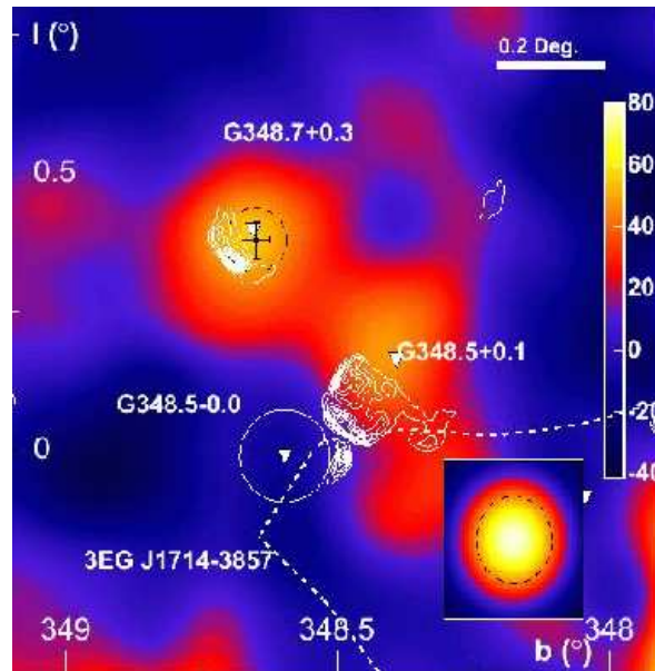
FIG. 7.1 – Carte d'excès de la région du complexe de supernova CTB 37, obtenue avec les observations de 2004. La carte est lissée à l'aide d'une Gaussienne de rayon 0.07^\circ . Les contours blancs sont les contours de la cartographie en ondes radio de Molonglo [107]. Le cercle blanc représente l'extension du vestige de supernova G348.5+0.0. La courbe blanche pointillée représente le contour de 68 % de confiance de la position de la source EGRET 3EG J1714-3857. La fonction d'étalement de l'instrument est représentée en bas à droite. Les coordonnées sont exprimées dans le référentiel galactique. Cette figure est tirée de [106].
