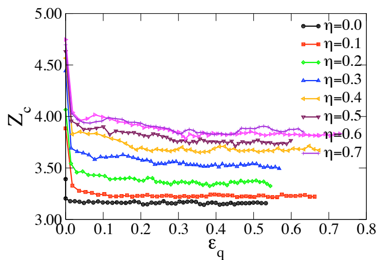
FIGURE 4.25 – Evolution du nombre de connectivité Z_c au cours du cisaillement en fonction de \eta pour les empilements cohésifs.
