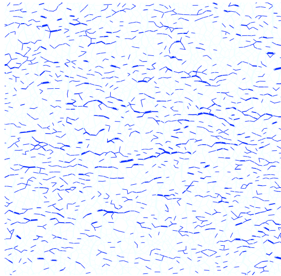
FIGURE 4.51 – Réseau de forces en traction au début de l'essai de compression simple ( \varepsilon_{yy} < 0,001 ) pour l'échantillon \eta = 0,1 .
