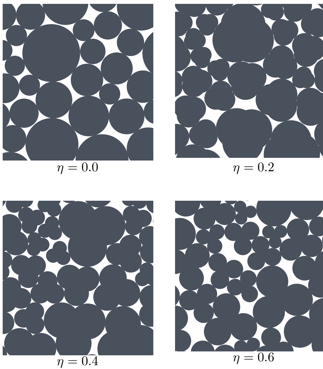
FIGURE 2.10 – Vues d'échantillons pour différentes valeurs de \eta à l'issue d'une compression isotrope.
