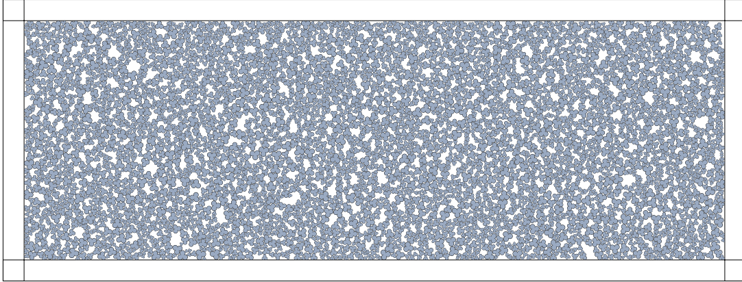
FIGURE 2.9 – La configuration des agrégats cohésifs avec \eta = 0,5 à la fin d'une compaction uniaxiale (compression œdométrique).
