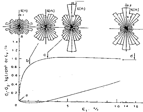
FIGURE 1.9 – La contrainte de cisaillement \sigma_1 - \sigma_3 et la déformation volumique cumulée \varepsilon_v en fonction de la déformation axiale \varepsilon_1 dans un test de compression bi-axiale sur un échantillon de disques. La distribution des orientations des contacts est représentée par un diagramme polaire à plusieurs stades de déformation. A l'état initial, il y a plus de contacts avec une orientation horizontale. Le nombre de contacts avec une orientation verticale augmente au cours de la compression verticale et devient prépondérant dans l'état critique [74].
