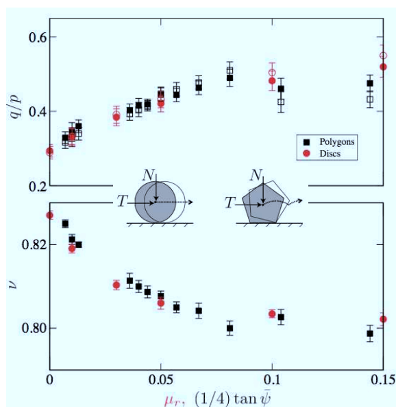
FIGURE 1.15 – La résistance au cisaillement q^*/p et la compacité critique \nu^* de deux systèmes composés respectivement de disques interagissant par un coefficient de frottement de roulement \mu_r (en plus d'un frottement de glissement) et de polygones réguliers avec un nombre croissant du nombre de côtés. Le paramètre \psi est inversement proportionnel au nombre de côtés d'après [33].
