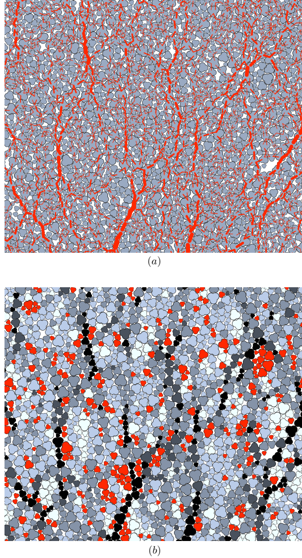
FIGURE 3.13 – Cartes du réseau de forces normales de contact (a) et du réseau des contraintes moyennes sur les particules (b). Les traits représentent les forces normales et leur épaisseur est proportionnelle à l'intensité de la force. Les particules en rouge ne subissent aucun effort et pour les autres particules le niveau de gris est proportionnel à la contrainte qu'elles supportent.
