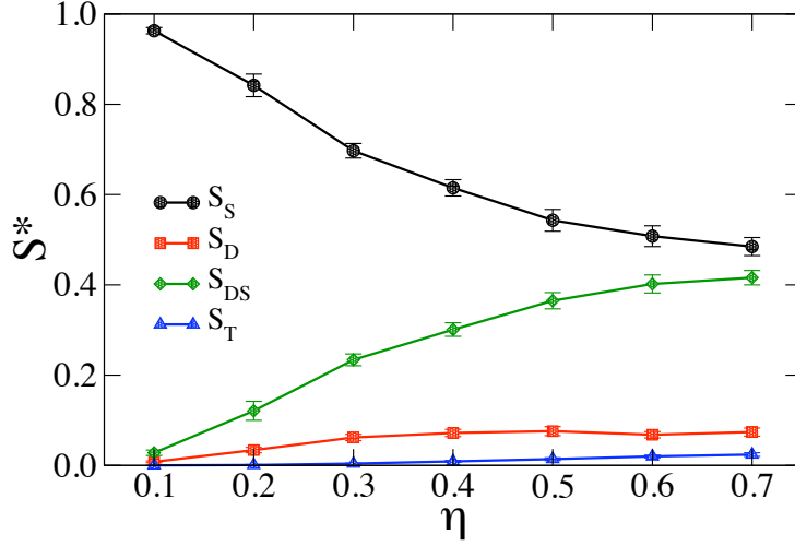
FIGURE 3.20 – Proportion des contacts critiques de différents types dans l'état critique en fonction de la non-convexité. Les barres d'erreur représentent l'écart-type des fluctuations autour de la valeur moyenne.
