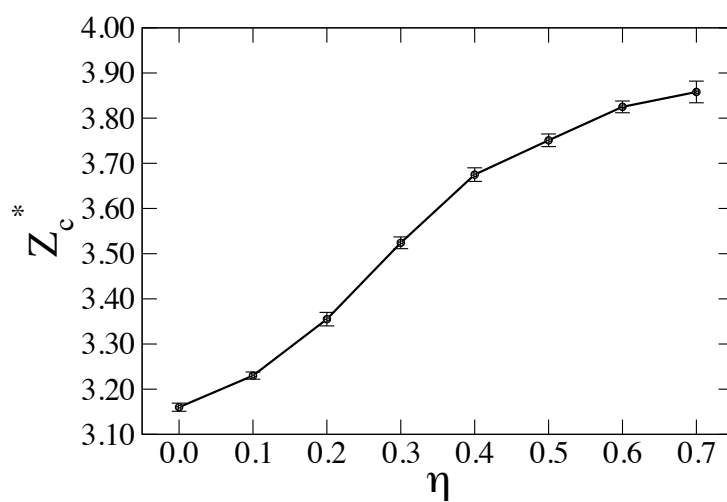
FIGURE 4.26 – Evolution de la valeur moyenne du nombre de connectivité Z_c dans l'état critique en fonction de \eta pour les empilements cohésifs. Les barres d'erreur désignent les fluctuations autour des valeurs moyennes dans l'état critique.
