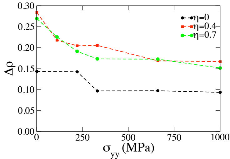
FIGURE 4.43 – Evolution du degré d'hétérogénéité de compacité \Delta\rho en fonction de la contrainte appliquée \sigma_{yy} pour les échantillons \eta = 0, \eta = 0,4 et \eta = 0,7 . L'échelle d'analyse est de l_c = 5\langle d \rangle .
