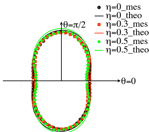
FIGURE 3.14 – Représentation polaire des distributions angulaires des forces normales moyennes \langle f_n \rangle(\theta) / \langle f_n \rangle ainsi que des approximations harmoniques dans l'état résiduel pour 3 valeurs de \eta .
