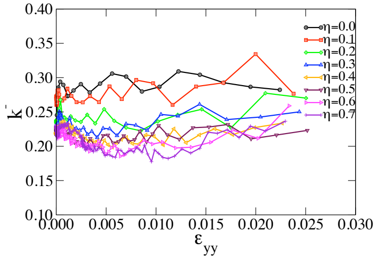
FIGURE 4.53 – Evolution de la proportion des contacts en traction k^- avec la déformation axiale \epsilon_{yy} .
