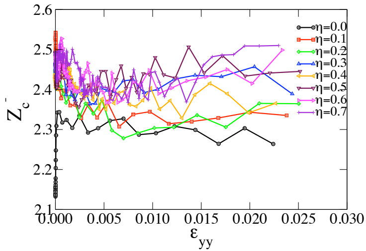
FIGURE 4.54 – Evolution du nombre de connectivité Z_c^- pour les contacts en traction en fonction de la déformation axiale \epsilon_{yy} .
