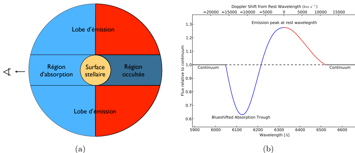
FIG. 2.5 – (a) Représentation géométrique d’une photosphère en expansion entraînant la formation de profil P-Cygni. (b) Représentation schématisique d’un profil P-Cygni. La partie bleue en absorption provient de la zone d’absorption en expansion vers l’observateur. Le pic d’émission, centré sur la longueur d’onde centrale dans son référentiel au repos, résulte de la diffusion dans les lobes d’émission.
