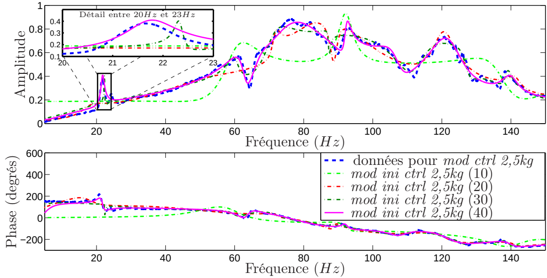
FIG. 2.7 – Modèles mod ini ctrl 2,5kg dans le domaine fréquentiel obtenus avec l'algorithme N4SID pour les ordres 10, 20, 30 et 40
