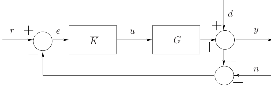
FIG. 3.6 – Configuration en boucle fermée
