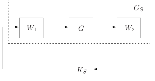
FIG. 4.2 – Schéma LSDP
